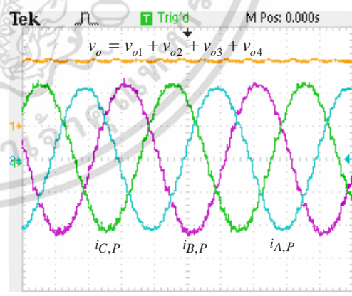
(ข) แรงดันด้านออกและกระแสด้านปฐมภูมิทั้ง 3 เฟส รูปที่ 9 แรงดันด้านออกและกระแสด้านปฐมภูมิทั้ง 3 เฟสของวงจรเรียงกระแส 24 พัลส์
