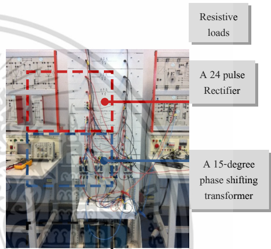
รูปที่ 7 ฮาร์ดแวร์วงจรเรียงกระแส 24 พัลส์ที่ใช้ในการทดสอบ
