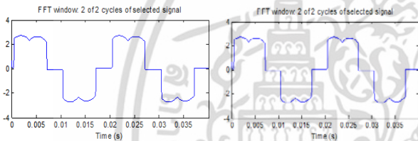
(ก) กระแสด้านทุติยภูมิชุดที่ 1 ( i_{s1} ) และสเปกตรัม
