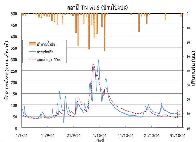
รูปที่ 4 ผลการปรับเทียบแบบจำลองที่สถานี TNwt.6
