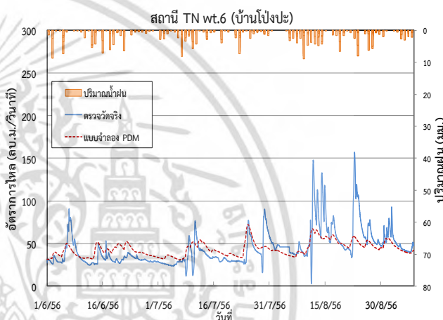
รูปที่ 5 ผลการตรวจพิสูจน์แบบจำลองที่สถานี TNwt.6
