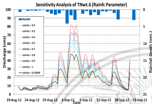
รูปที่ 6 ผลการวิเคราะห์ความไวของตัวแปร rainfac จากแบบจำลอง PDM
