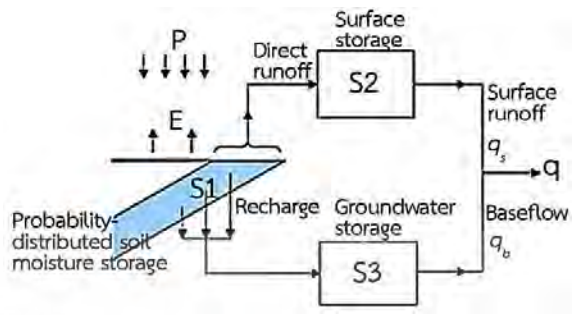
รูปที่ 3 ผังการทำงานของแบบจำลอง InfoWorks PDM
