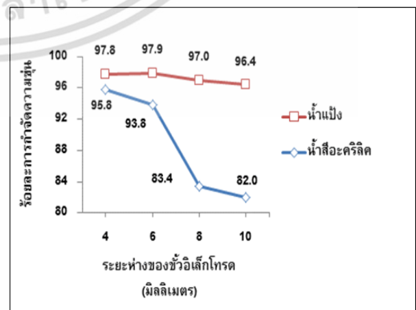
รูปที่ 5 ร้อยละการกำจัดความขุ่นด้านการค้า
