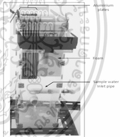
รูปที่ 2 ถังปฏิกรณ์ที่ติดตั้งขั้วซึ่งอิเล็กโทรด
