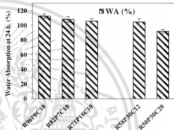
รูปที่ 7 ผลกระทบของปริมาณเส้นใยผลตาลโตนดและแป้งมันสำปะหลังต่อเปอร์เซ็นต์การดูดซับน้ำ
