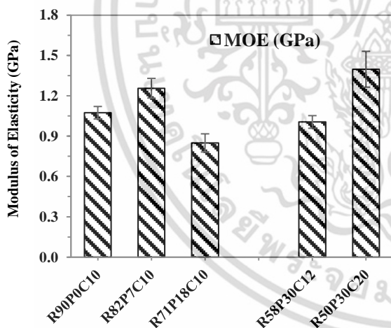
รูปที่ 5 ผลกระทบของปริมาณเส้นใยผลตาล โคนดและแป้งมันสำปะหลังต่อค่ามอดูลัสการดัด
