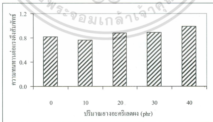
รูปที่ 9 ผลของปริมาณยางอะครีเลตผงต่อสมบัติความทนทานต่อความร้อนของยางคงรูป
