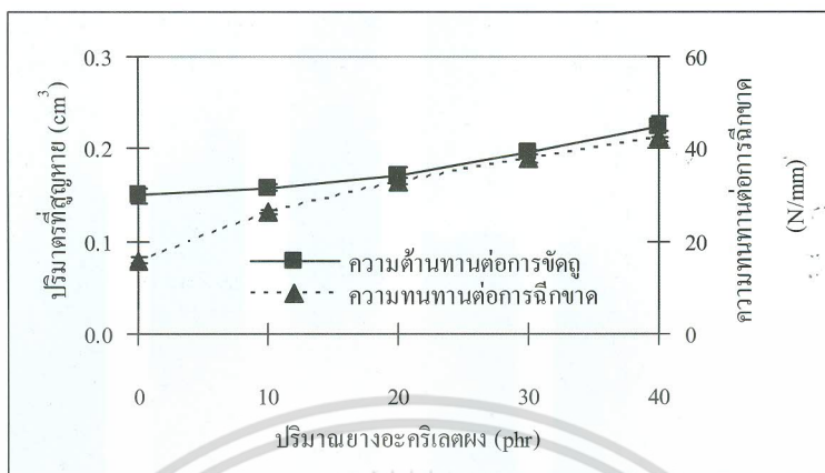
รูปที่ 7 ผลของปริมาณยางอะครีเลตผงต่อความทนทานต่อการฉีกขาดและความต้านทานต่อการขีดข่วนของยาง
