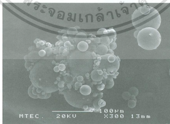
รูปที่ 1 SEM ไมโครกราฟของยางอะคริเลตผสมที่กำลังขยาย 300 เท่า
