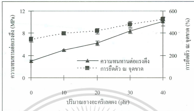
รูปที่ 5 ผลของปริมาณยางอะครีเลตผงต่อความทนทานต่อแรงดึงและการยืดตัว ณ จุดขาดของยางคงรูป
