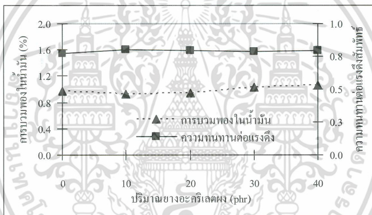
รูปที่ 8 ผลของปริมาณยางอะครีเลตผงต่อสมบัติความทนทานต่อน้ำมันของยางคงรูป
