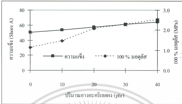
รูปที่ 2 ผลของปริมาณยาง อะครีเลตฟงต่อความแข็งและ 100% มอดุลัสของยางคงรูป
