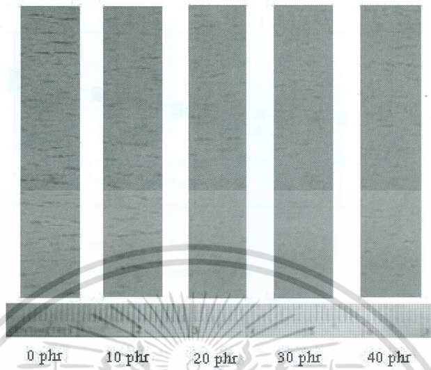
รูปที่ 10 ผลของปริมาณยางอะครีเลตผดงต่อความทนทานไอโซนของยางกรุป
