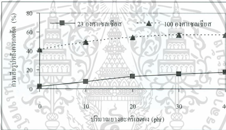
รูปที่ 3 ผลของปริมาณยางอะครีเลตฟงต่อค่าการเสีรูปดาวรหลังกดของยางคงรูป
