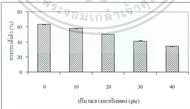
รูปที่ 4 ผลของปริมาณยางอะครีเลตฟงต่อค่าการกระเซ็งกระดอนของยางคงรูป
