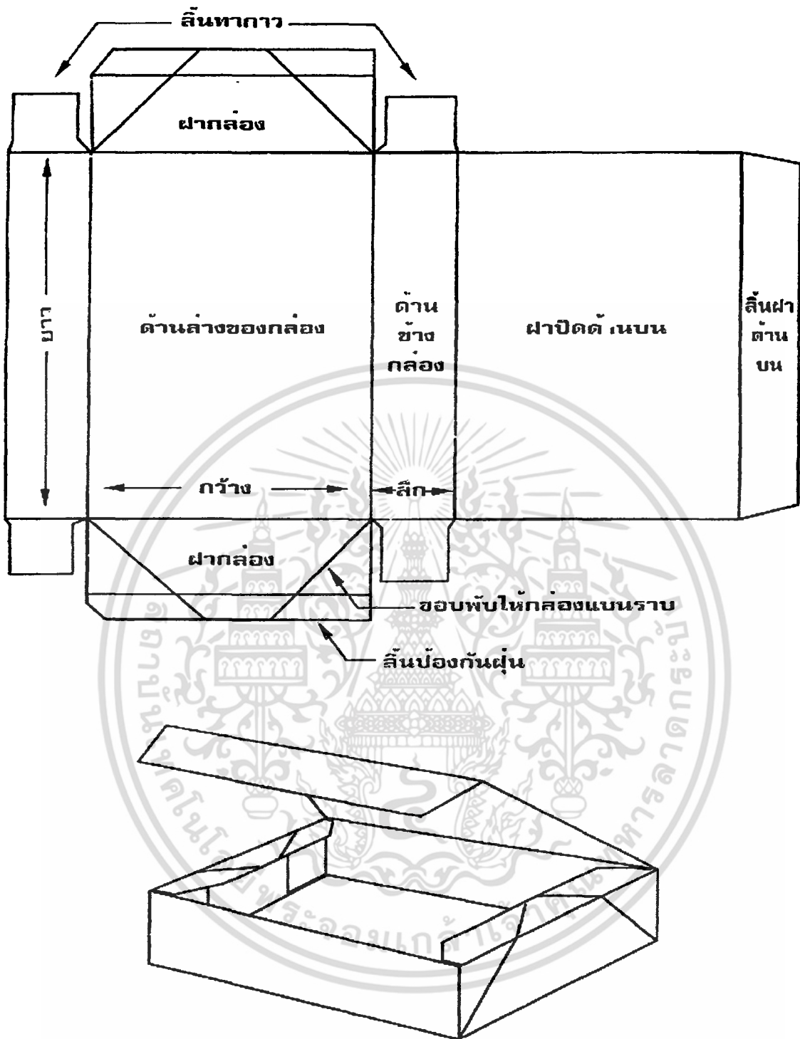
ภาพที่ 2.5 กล่องกระดาษแบบถาด
