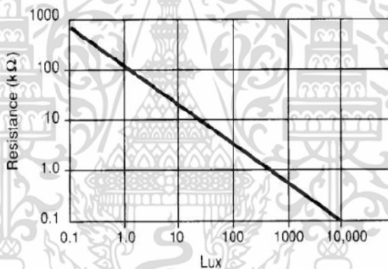
รูปที่ 3.15 กราฟแสดงความสัมพันธ์ระหว่างความต้านทานกับความเข้มแสง
