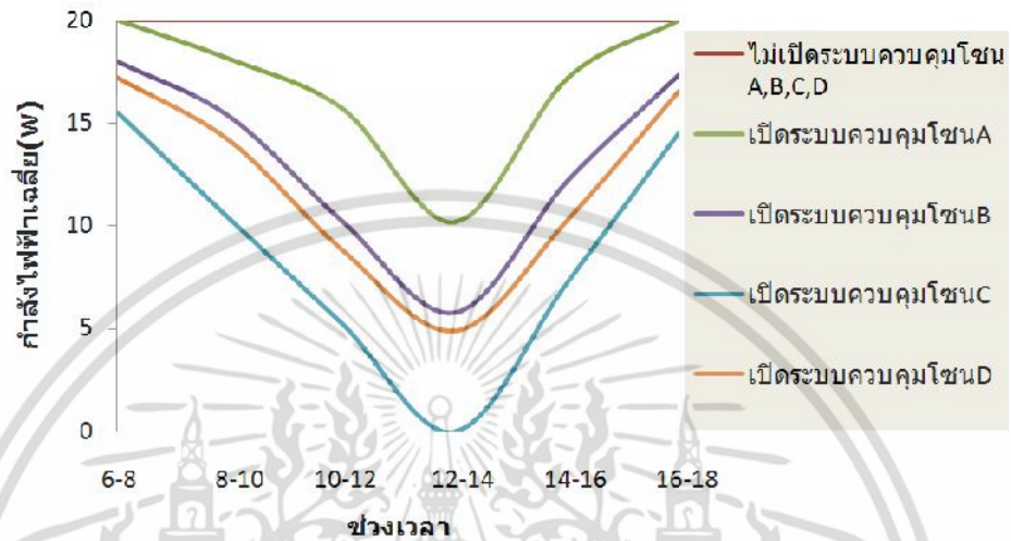
รูปที่ 4.7 กำลังไฟฟ้าเฉลี่ยในแต่ละช่วงเวลา
