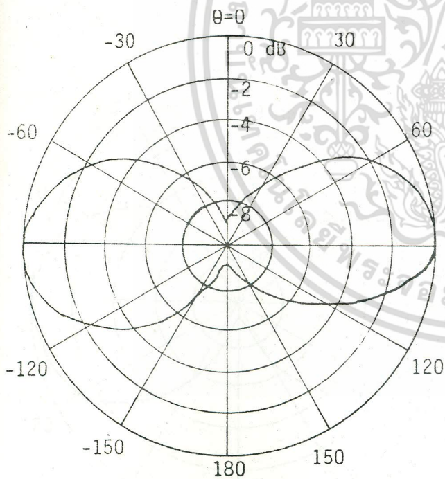
(ค) C_\lambda = 0.189
