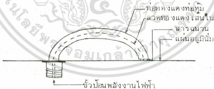
รูปที่ 5.1 ภาคตัดขวางการวางสายอากาศห้วงครึ่งวงรีห่อหุ้มบนกราวด์-อลูมิเนียม
