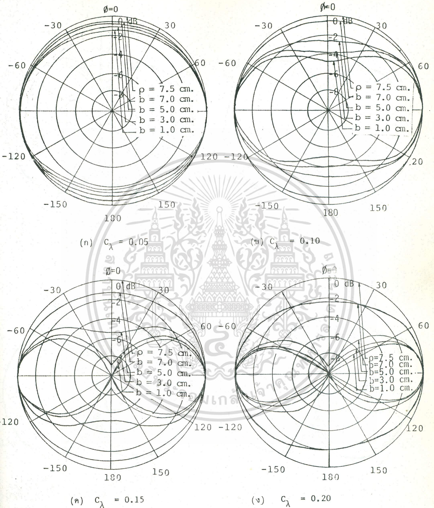
รูปที่ 4.2 ผลการคำนวณแพทเทิร์นการแพร่คลื่นของสายอากาศห่องวงรีขนาดเล็กในระนาบสนาม
