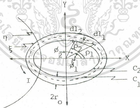
รูปที่ 4.6 ลักษณะการวางสายอากาศห้วงวงรีเปลี่ยน บนแกน X, Y
