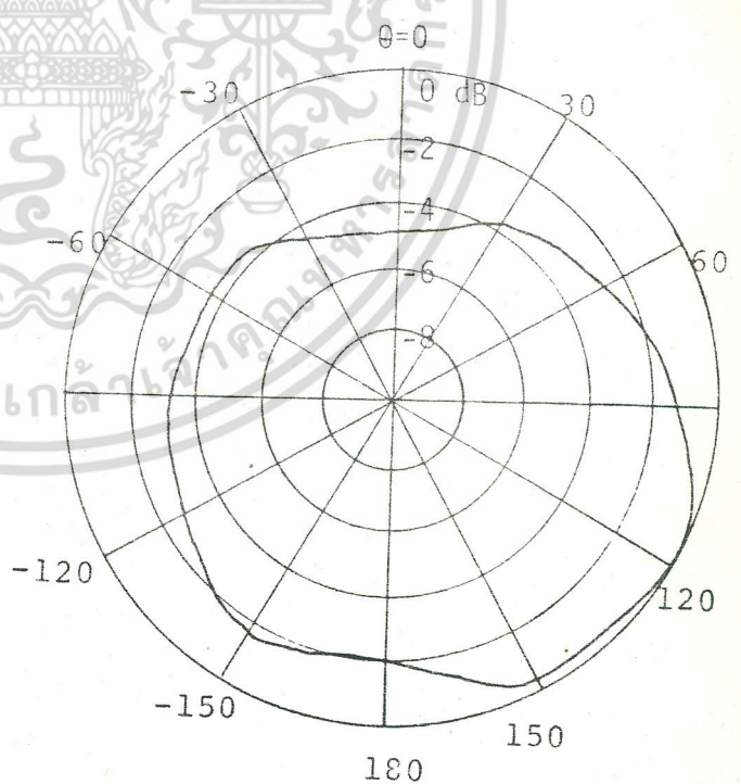
(ง) C_\lambda = 0.192
