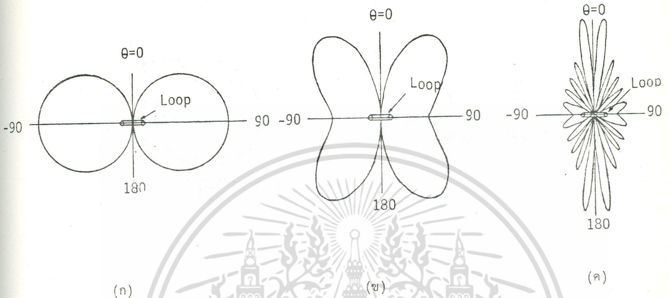
รูปที่ 2.2 แพทเทิร์นการแผ่คลื่นของสายอากาศห่วงเปลี่ยนขนาดต่างๆ (H-Plane) (ก) 2p \ll \lambda (ข) 2p = \lambda (ค) 2p = 5\lambda
