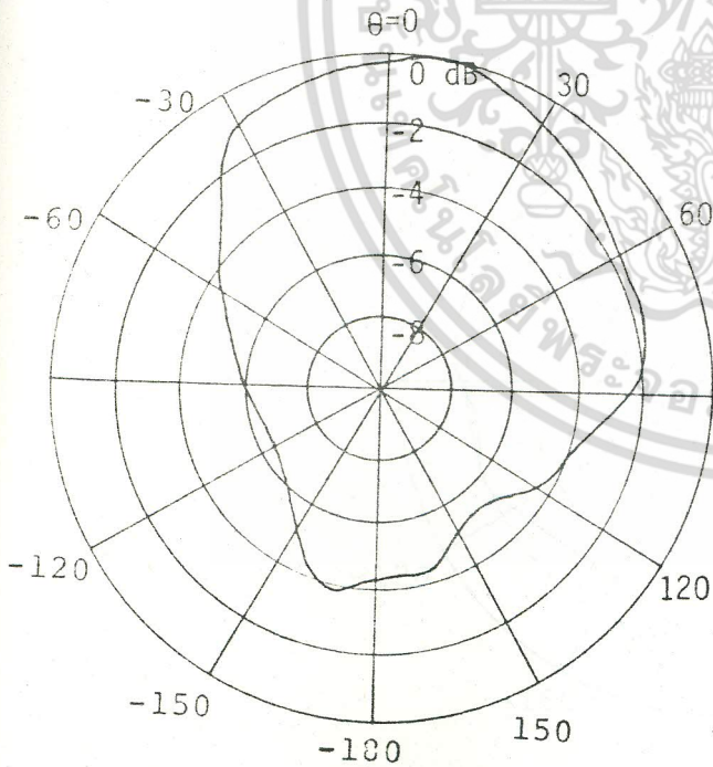
(ค) C_\lambda = 0.189
