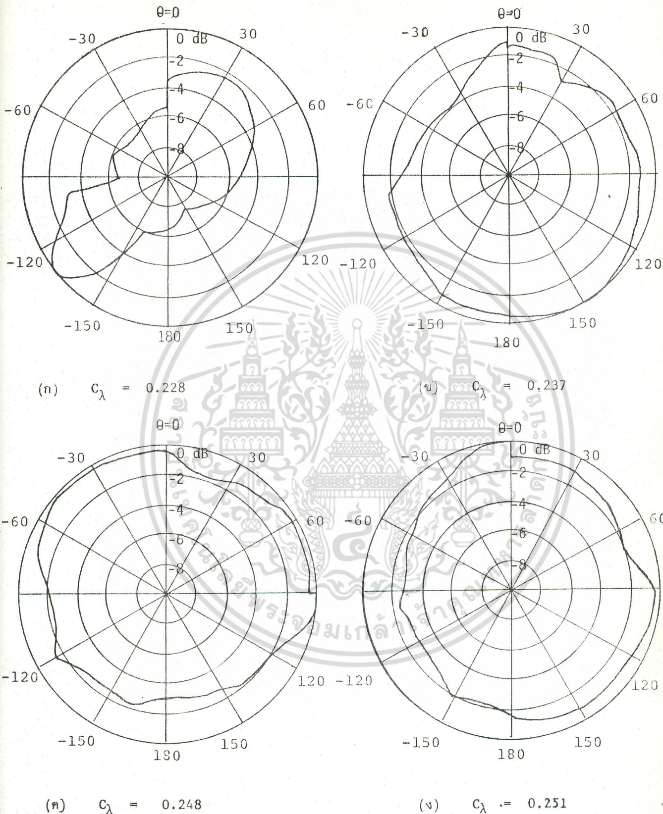
รูปที่ 5.2 ตัวอย่างแพทเทิร์นการแพร่คลื่นระนาบสนามแม่เหล็ก ท่วงวงกลมเบสิค
