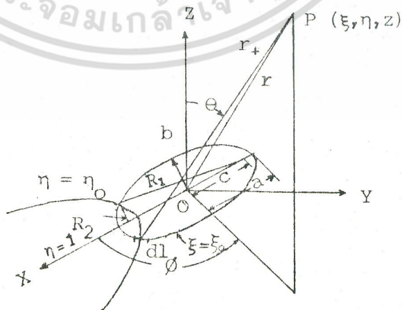
รูปที่ 4.1 ลักษณะการวางสายอากาศห้วงวงรีที่หุ้มในโคออร์ดิเนตทรงกระบอกวงรี
