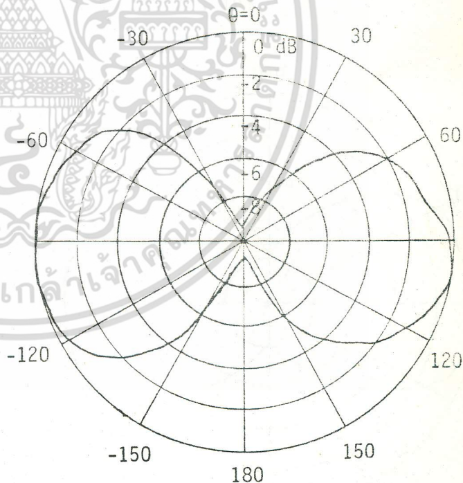
(ง) C_\lambda = 0.192
