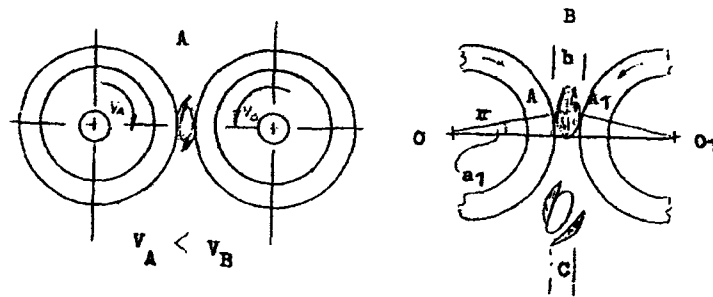
ภาพที่ 2.6 หลักการกะเทาะของเครื่องกะเทาะแบบลูกยาง [33]
