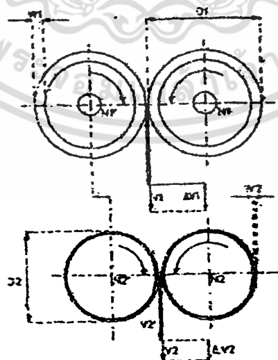
ภาพที่ 2.7 ความสัมพันธ์ระหว่างเส้นผ่าศูนย์กลางลูกยางและความสามารถของเครื่องกะเทาะ [33]
