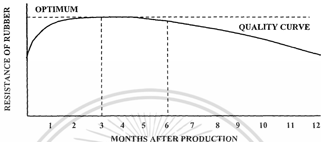
ภาพที่ 2.8 ความสัมพันธ์ระหว่างความคงทนของลูกยางและอายุการเก็บรักษาลูกยางดัดแปลงมาจาก [33]
