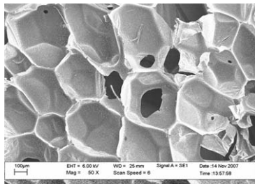
สูตร A2 ผสมเศษด้ายไหม 5 กรัม
