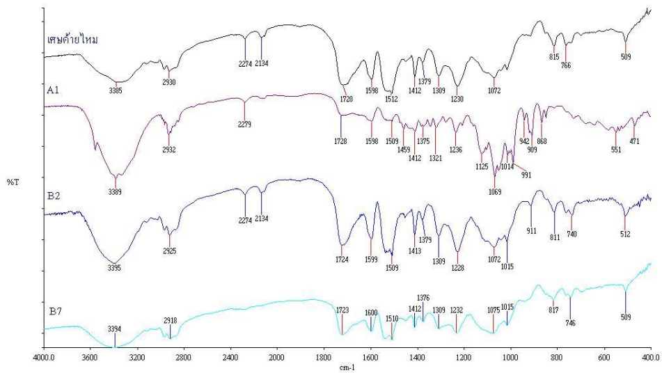
รูปที่ 5 FTIR ของเศษด้ายไหม โฟมพอลิยูรีเทน สูตร A1 สูตร B2 และ สูตร B7
