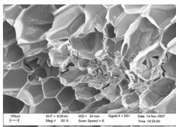
สูตร B2 ผสมเศษด้ายไหม 5 กรัม
