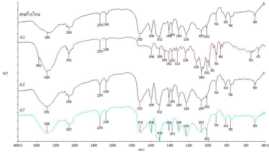
รูปที่ 4 FTIR ของเศษด้ายไหม โฟมพอลิยูรีเทน สูตร A1 สูตรA2 และ สูตร A7
