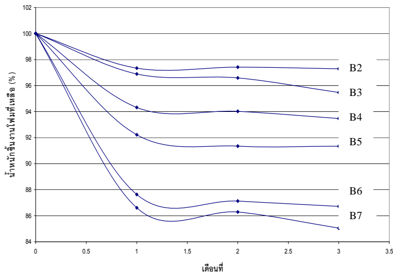
รูปที่ 7 ร้อยละน้ำหนักที่เหลือของชิ้นงาน โฟมพอลิยูรีเทนสูตรต่างๆ ที่เตรียมด้วยวิธี B หลังจากนำไปทดสอบการย่อยสลาย 3 เดือน
