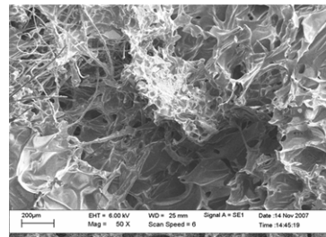
สูตร A7 เศษด้ายไหมปริมาณ 30 กรัม
