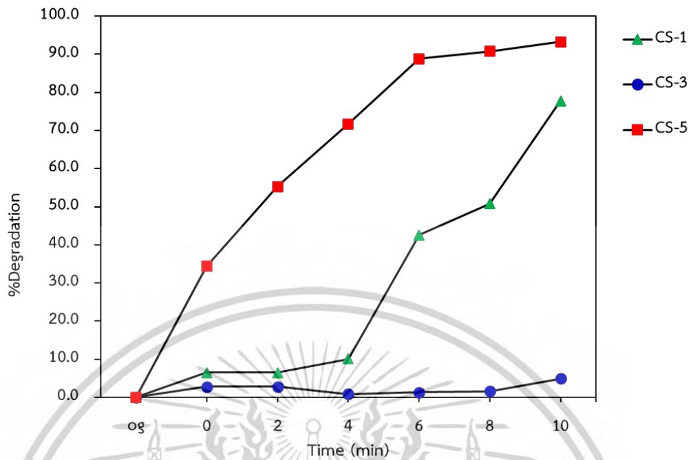
รูปที่ ข.2 เปอร์เซ็นการสลายตัวของ MO ที่เวลาต่าง ๆ หลังทำปฏิกิริยารีดักชันด้วย \text{NaBH}_4 มีอนุภาค คอปเปอร์ที่สังเคราะห์ได้เป็นตัวเร่งปฏิกิริยา
