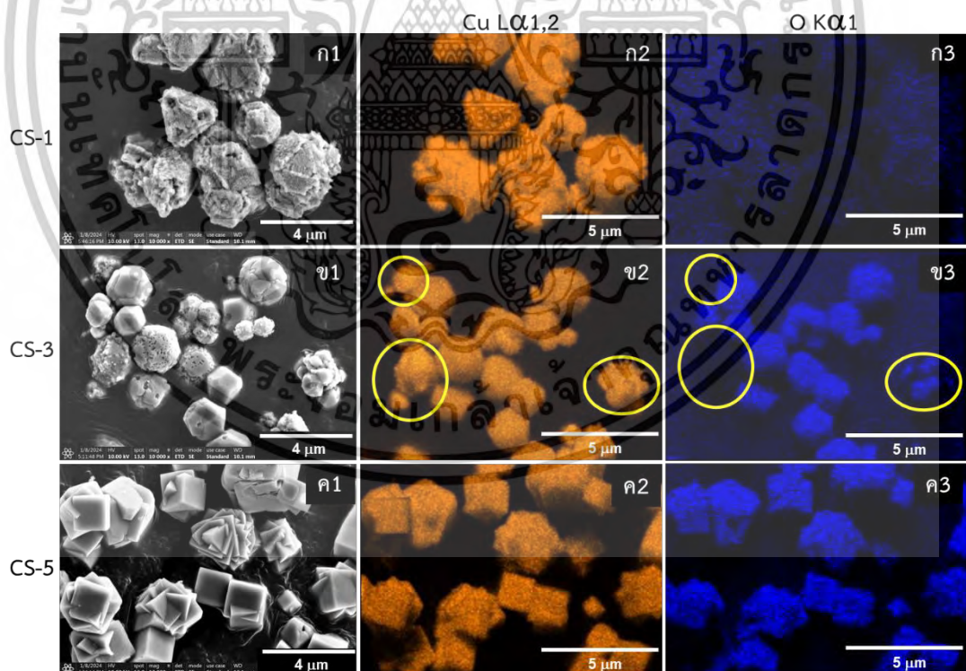
รูปที่ 4.7 การวิเคราะห์การกระจายตัวของธาตุคอปเปอร์และออกซิเจนเชิงพลังงาน (EDS mapping) ของอนุภาคคอปเปอร์ (ก) CS-1, (ข) CS-3, และ (ค) CS-5 วงกลมสีเหลืองแสดงอนุภาคคอปเปอร์ที่ไม่เอกสารนี้เป็นเอกสารที่สงวนไว้สำหรับการใช้งานเพื่อการศึกษาเท่านั้น เมื่ออนุญาตให้นำไปใช้ประโยชน์ด้านการค้าไม่ว่ากรณีใดๆทั้งสิ้น อีกทั้งห้ามมิให้ดัดแปลงเนื้อหา และต้องอ้างอิงถึงเจ้าของเอกสารทุกครั้งที่มีการนำไปใช้
