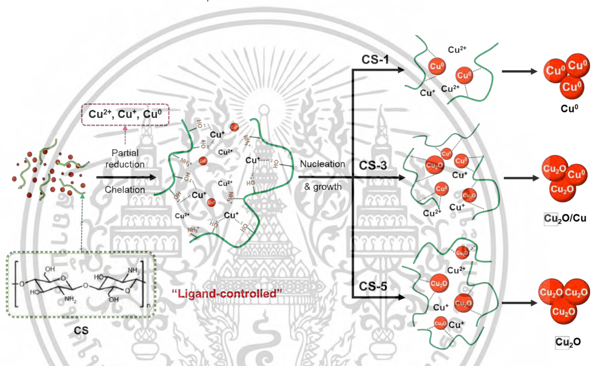
รูปที่ 4.12 กลไกการเกิดอนุภาคคอปเปอร์ ( \text{Cu}^0 ) และคิวปริสออกไซด์ ( \text{Cu}_2\text{O} ) ด้วยไคโตซานและกรดแอสคอร์บิกโดยวิธีการสังเคราะห์ด้วยเครื่องนึ่งแรงดันไอน้ำ (Autoclave)
