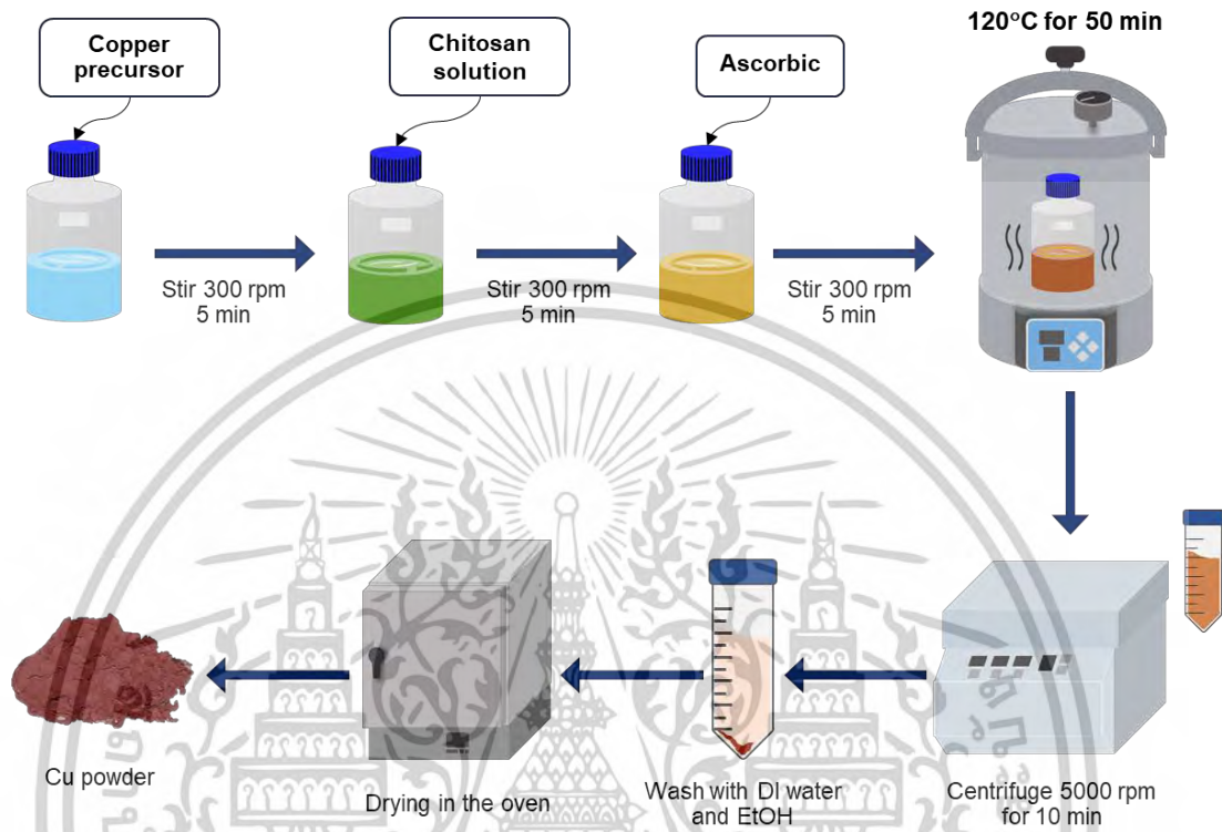
รูปที่ ข.1 แผนผังการสังเคราะห์อนุภาคคอปเปอร์ด้วยเครื่องนึ่งแรงดันไอน้ำ (Autoclave-assisted method)
