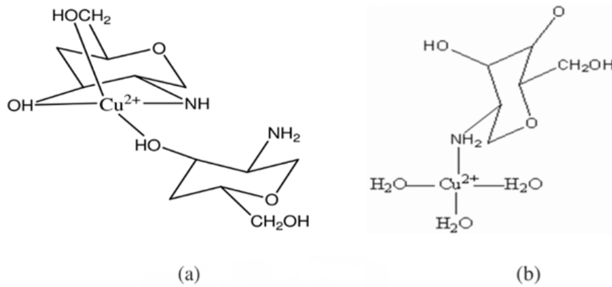
รูปที่ 2.6 โครงสร้างสารประกอบโคโคโตซานจับกับโลหะคอปเปอร์ไอออน (a) Bridge fashion (b) pendant fashion [22]
