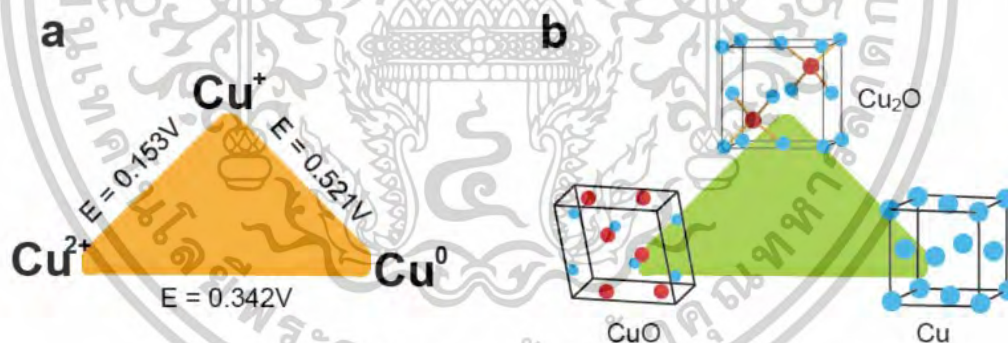
รูปที่ 2.1 (a) ค่า Reduction potential (b) โครงสร้างผลึกของคอปเปอร์ (FCC; \text{Cu}^0 ) คอปเปอร์ออกไซด์ (Monoclinic; \text{CuO} ) และ คิวปริสออกไซด์ (Cubic; \text{Cu}_2\text{O} ) [16]
