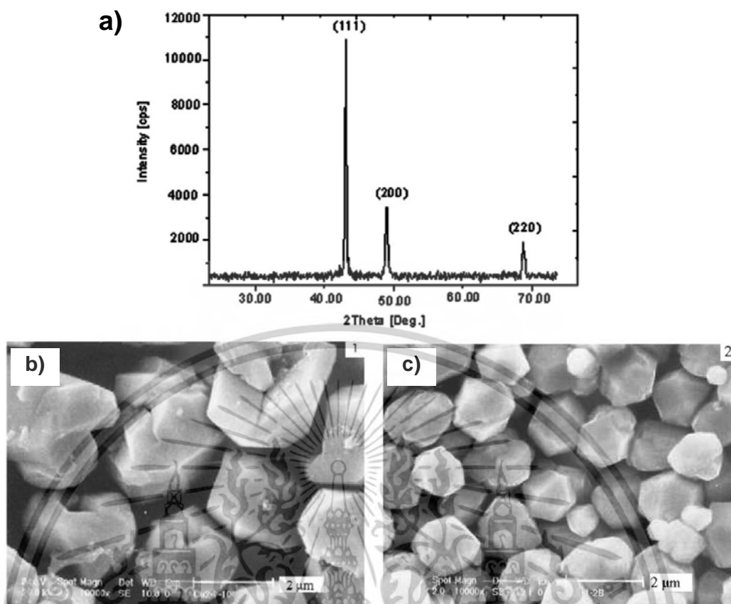
รูปที่ 2.11 (a) รูปแบบการเลี้ยวเบนของรังสีเอกซ์ และรูป SEM ของอนุภาคคอปเปอร์ที่ค่า pH แตกต่างกัน (b) pH 2.2 (c) pH 6 [23]
