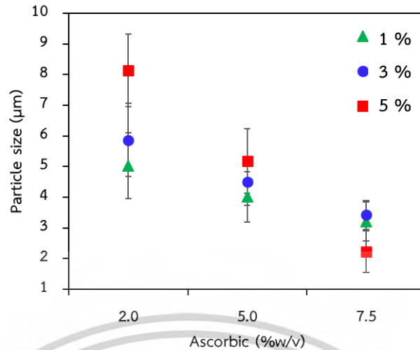
รูปที่ 4.6 ขนาดอนุภาคโดยเฉลี่ยของอนุภาคคอปเปอร์ที่ปริมาณโคโตซาน 1 3 และ 5 % และกรดแอสคอร์บิกแตกต่างกัน สังกะหราะห์ในเครื่องนึ่งแรงดันไอน้ำ (Autoclave) ที่อุณหภูมิ 120 องศาเซลเซียส ความดัน 15 ปอนด์ต่อตารางนิ้ว เป็นเวลา 50 นาทีโดยการวัดขนาดอนุภาคจากโปรแกรม ImageJ เป็นจำนวน 100 อนุภาค
