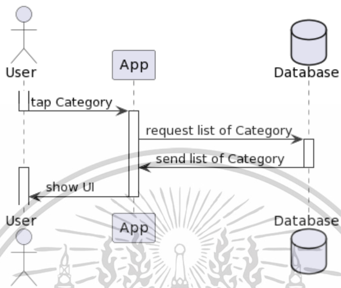
รูปที่ 3.9 Sequence Diagram ของการเรียกดูหน้าหมวดหมู่
