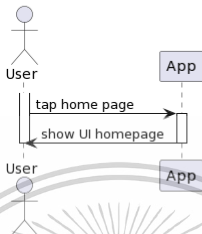
รูปที่ 3.4 Sequence Diagram ของการใช้งานหน้าHome
