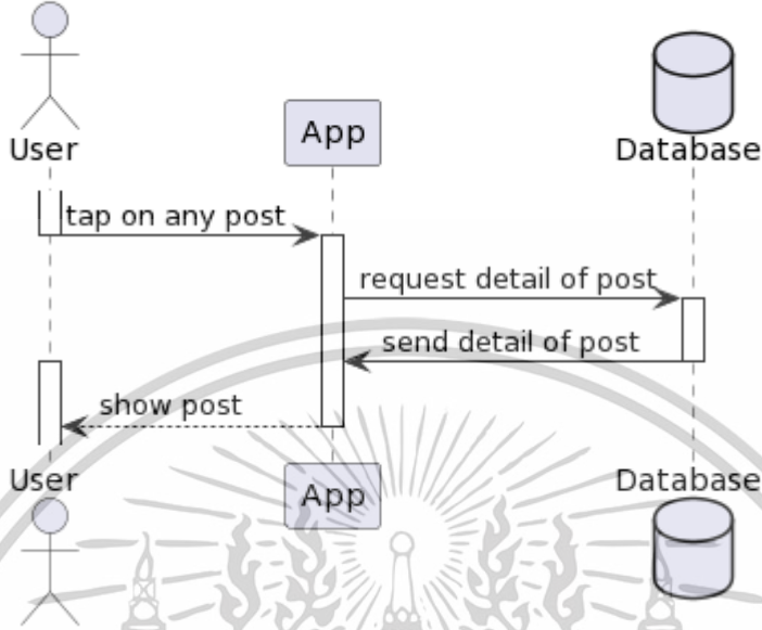
รูปที่ 3.8 Sequence Diagram ของการเรียกดูหน้าโพสต์ที่ต้องการ
