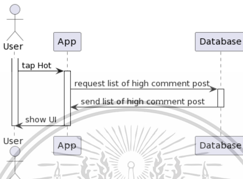
รูปที่ 3.5 Sequence Diagram การเรียกดูลิสต์โพสต์ยอดนิยมในหน้าแรก
