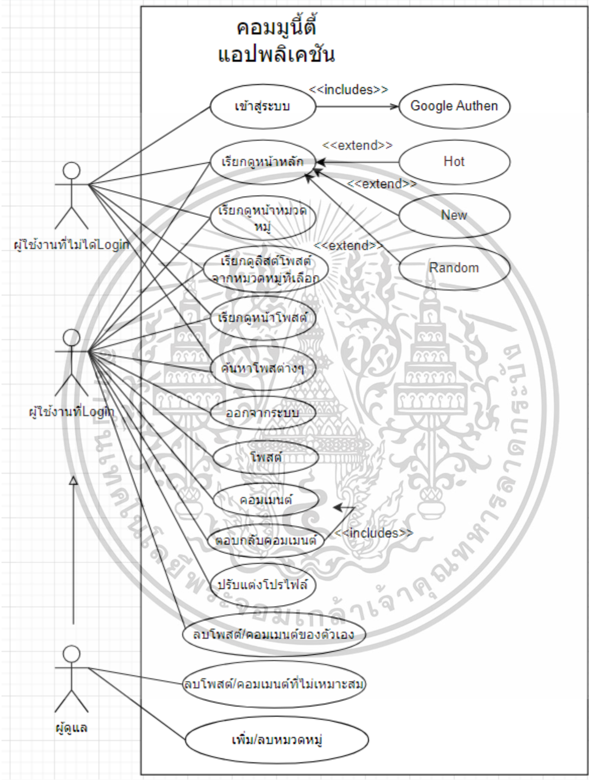
รูปที่ 3.2 Use Case Diagram ของแอปพลิเคชันสังคมออนไลน์
