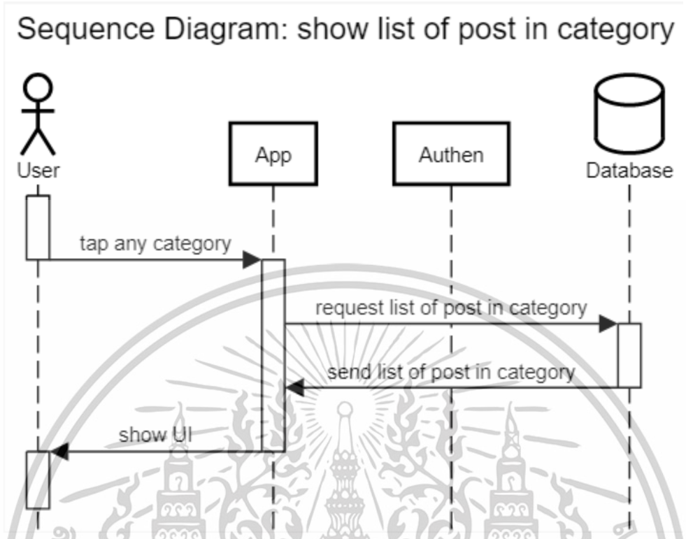
รูปที่ 3.10 Sequence Diagram ของการเรียกดูลิสต์โพสต์จากหมวดหมู่ที่เลือก
