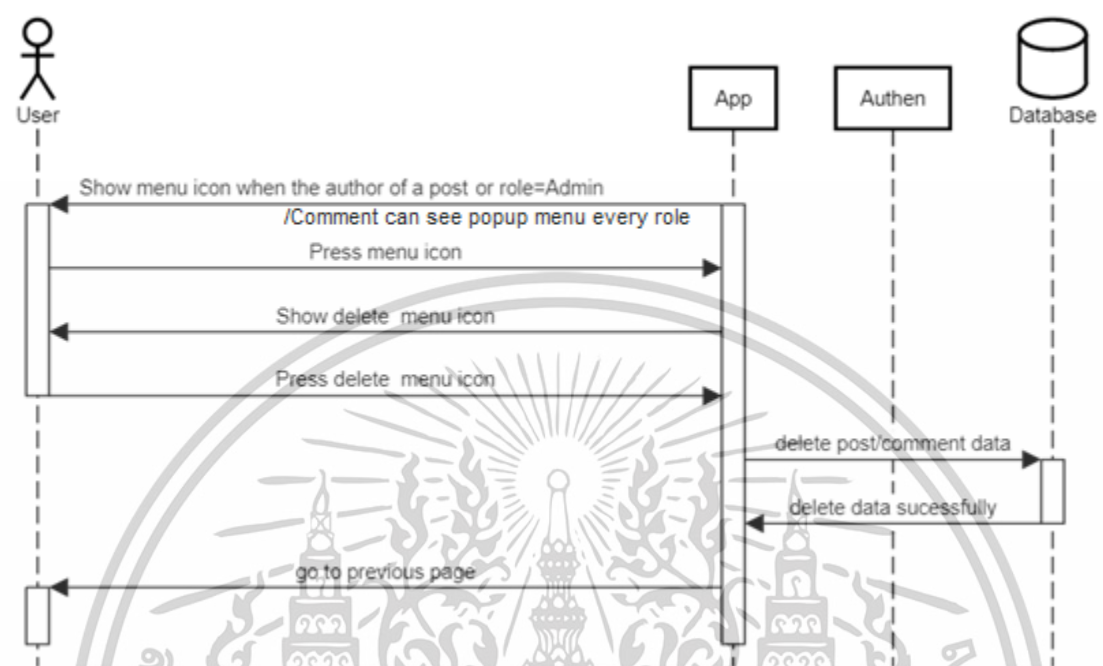
รูปที่ 3.15 Sequence Diagram ของการลบโพสต์/คอมเมนต์
