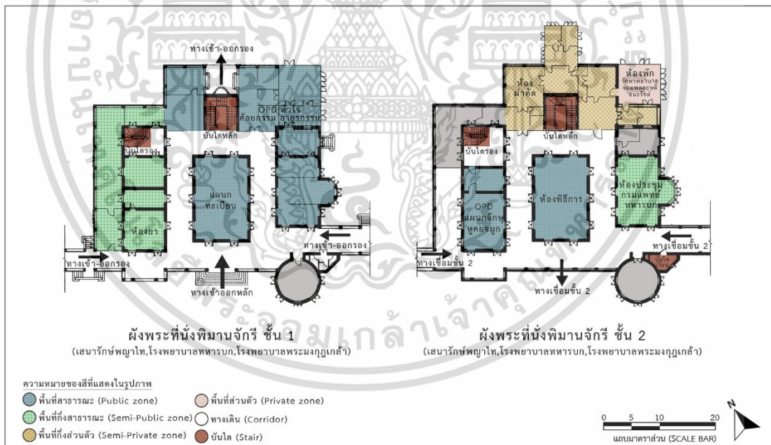
รูปที่ 4.7 ผังพระที่นั่งพิมานจักรี ยุคโรงพยาบาล (พ.ศ.2475-2512)
