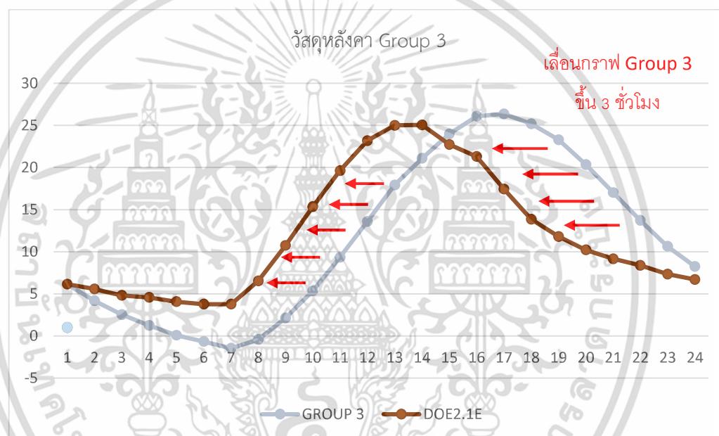
รูปที่ 4.34 แสดงวิธีการเปรียบเทียบปริมาณ Heat Gain ของวัสดุหลังคารายชั่วโมง ด้วยวิธี CLTD/CLF (Group 3) กับการคำนวณโดยจำลองด้วยโปรแกรม DOE2.1E
