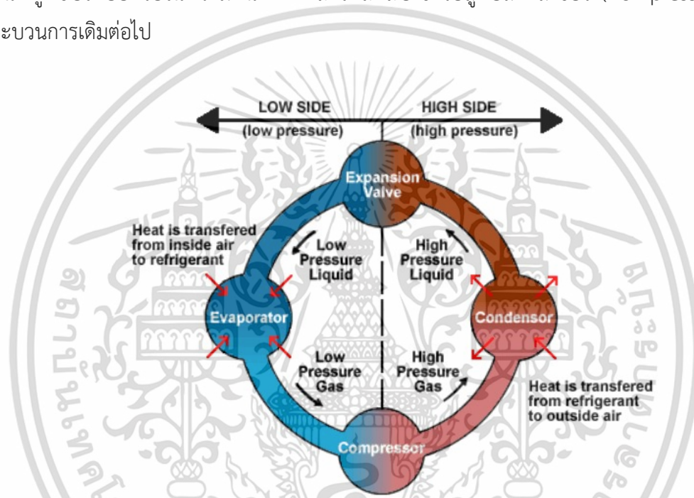
รูปที่ 2.3 แสดงวงจรการทำงานของเครื่องปรับอากาศ
