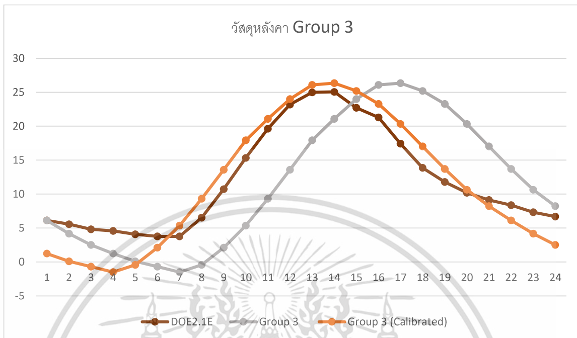
รูปที่ 4.35 แสดงการเปรียบเทียบปริมาณ Heat Gain ของวัสดุหลังคารายชั่วโมง ด้วยวิธี CLTD/CLF (Group 3) กับการคำนวณโดยจำลองด้วยโปรแกรม DOE2.1E ที่มา : ผู้วิจัย
