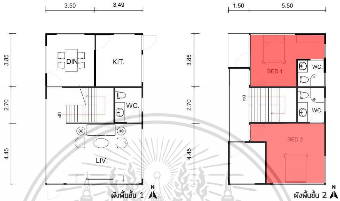
รูปที่ 3.2 แสดงผังบ้านพักอาศัยพื้นฐานและตำแหน่งพื้นที่ปรับอากาศ ที่มา : ผู้วิจัย
