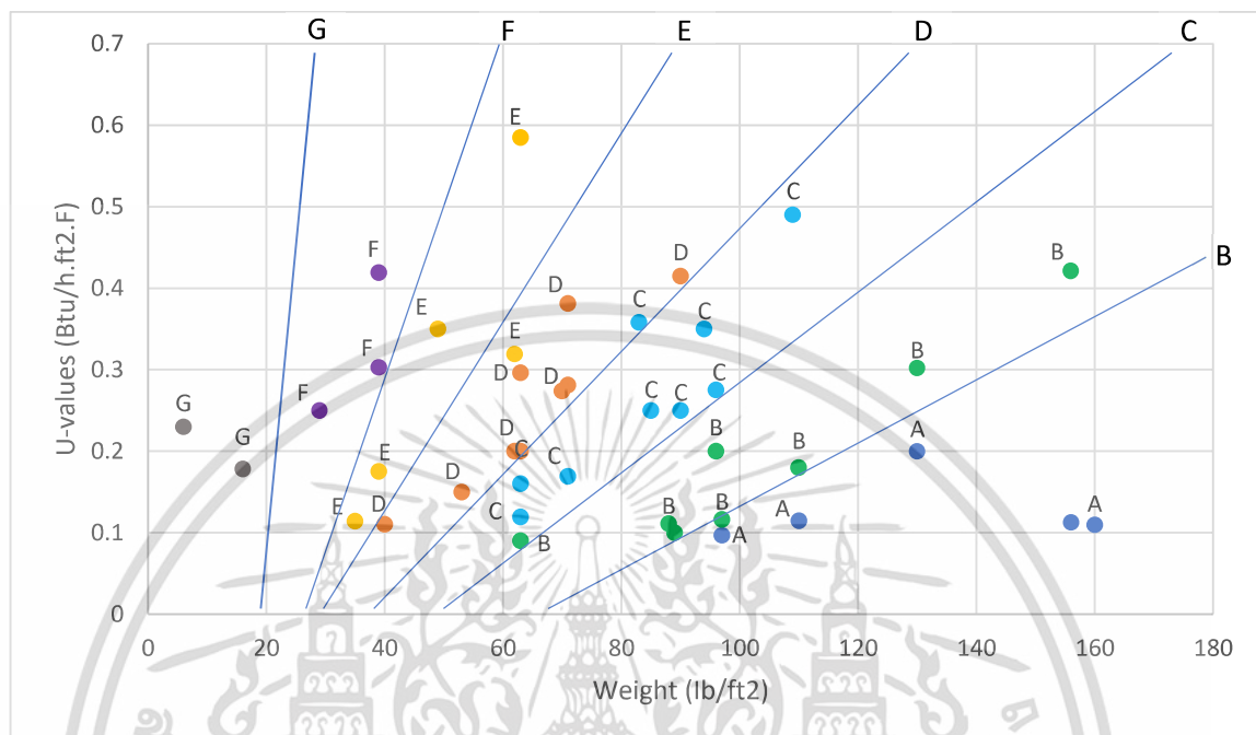
รูปที่ 4.3 แสดงแผนภูมิการกำหนดการแยกกลุ่มวัสดุผนังสำหรับการคำนวณด้วยวิธี CLTD/CLF
