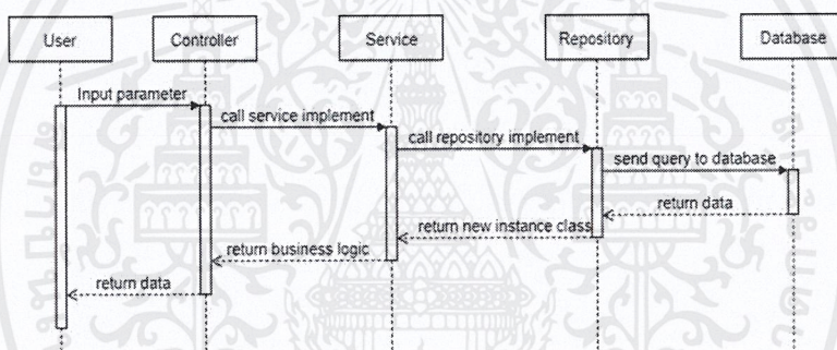
รูปที่ 3.22 Sequence Diagram การทำงานของ API
