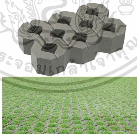
รูปที่ 8-6 บล็อกปูพื้น รุ่น บล็อกสนามหญ้า (SCG, 2563)
