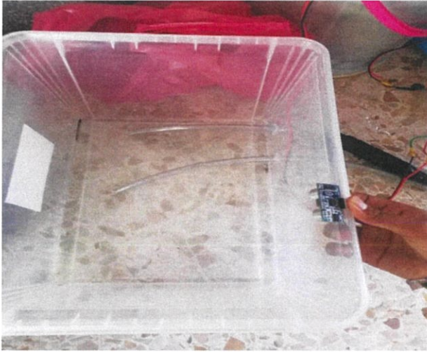
รูปที่ 4.5 ปริมาณน้ำที่วัดได้จากอุปกรณ์รับรู้วัดระยะทาง (Ultrasonic HC-SR04)
