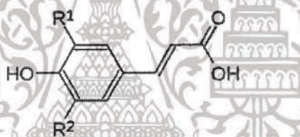
รูปที่ 2.2 โครงสร้างกรดไฮดรอกซีซินนามิก (Hydroxycinnamic acid)
