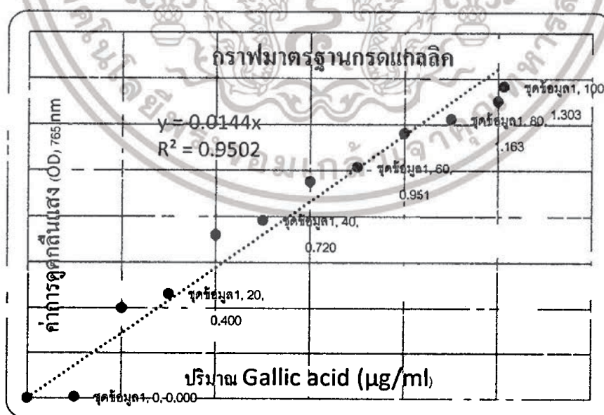
รูปที่ ผ-5 กราฟมาตรฐานของสารละลายมาตรฐานกรดแกลลิกที่ความเข้มข้น 1,000 \mu\text{g/ml}
