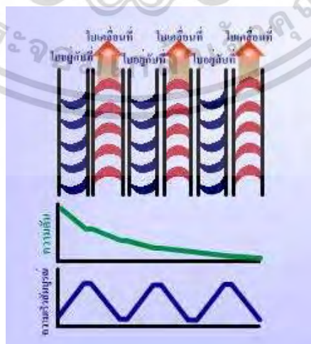
รูปที่ 2.15 กังหันแรงปฏิกริยาสามสเตจ แสดงความดันและความเร็วสัมบูรณ์ของไอน้ำ
