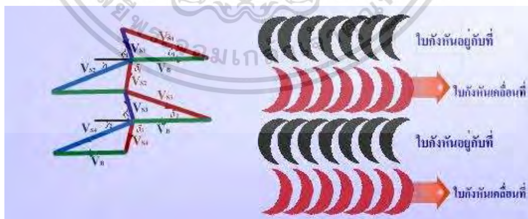
รูปที่ 2.17 แผนภาพความเร็วของกังหันปฏิกิริยาสองสเตจ
