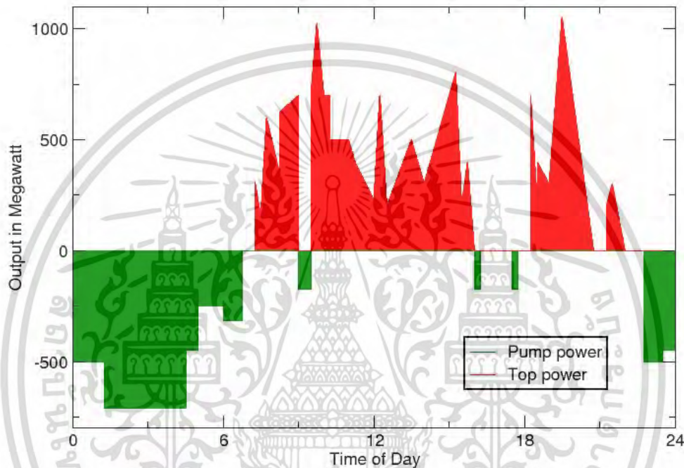
รูปที่ 2.6 กราฟแสดงการใช้ไฟฟ้าและการผลิตไฟฟ้าของโรงไฟฟ้าพลังน้ำแบบสูบกลับ
