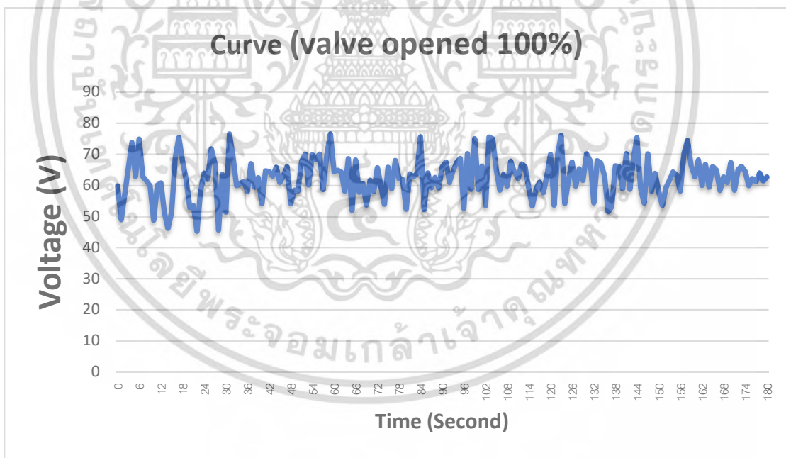
รูปที่ 4.15 กราฟแสดงแรงดันที่ผลิตได้โดยใช้กังหันน้ำแบบ Curve และเปิดวาล์ว 100%
