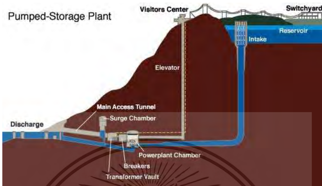
รูปที่ 2.4 โรงไฟฟ้าแบบสูบกลับ
