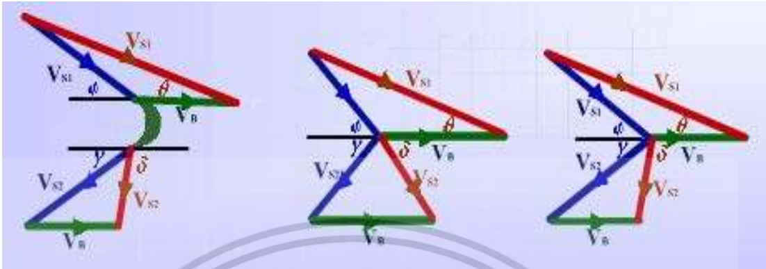
รูปที่ 2.11 ไดอะแกรมความเร็วของใบกังหันและสามเหลี่ยมความเร็วของกังหัน
