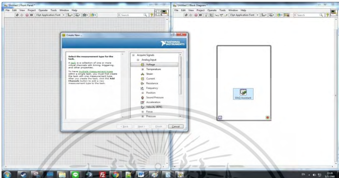
รูปที่ 3.63 ตั้งค่า DAQ Assistance
