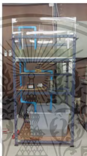
รูปที่ 4.4 การทดสอบประสิทธิภาพกังหันน้ำแบบ Pelton
