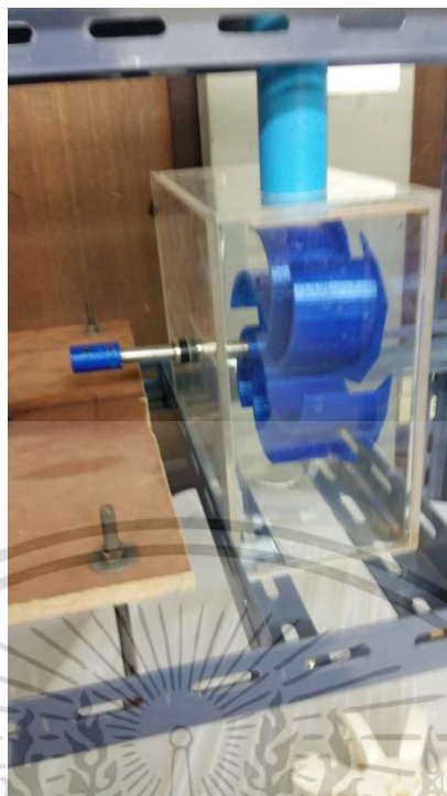
รูปที่ 3ข การติดตั้งกังหันน้ำ 3
