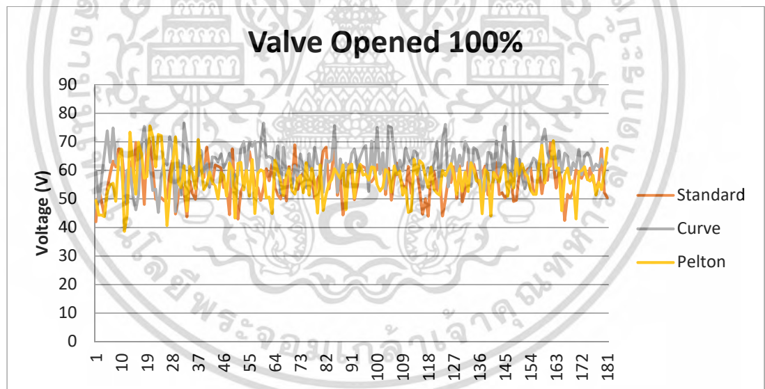
รูปที่ 4.17 กราฟแสดงแรงดันที่ผลิตได้โดยใช้กังหันน้ำทั้ง 3 แบบโดยเปิดวาล์ว 100%
