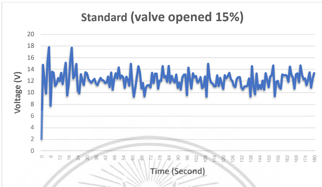
รูปที่ 4.10 กราฟแสดงแรงดันที่ผลิตได้โดยใช้กังหันน้ำแบบ Standard และเปิดวาล์ว 15%
