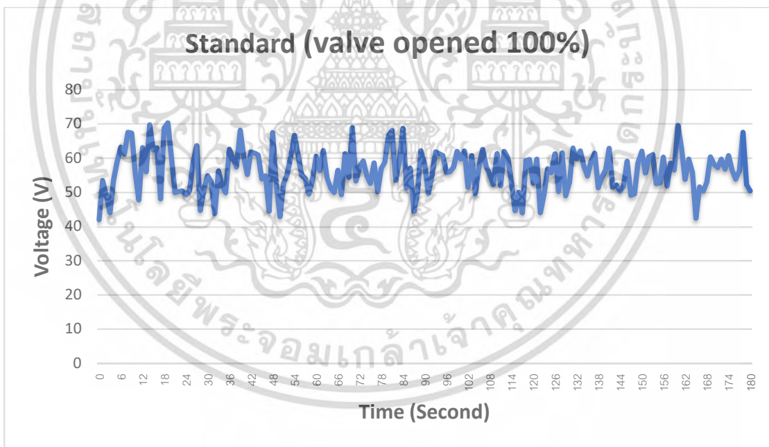
รูปที่ 4.11 กราฟแสดงแรงดันที่ผลิตได้โดยใช้กังหันน้ำแบบ Standard และเปิดวาล์ว 100%
