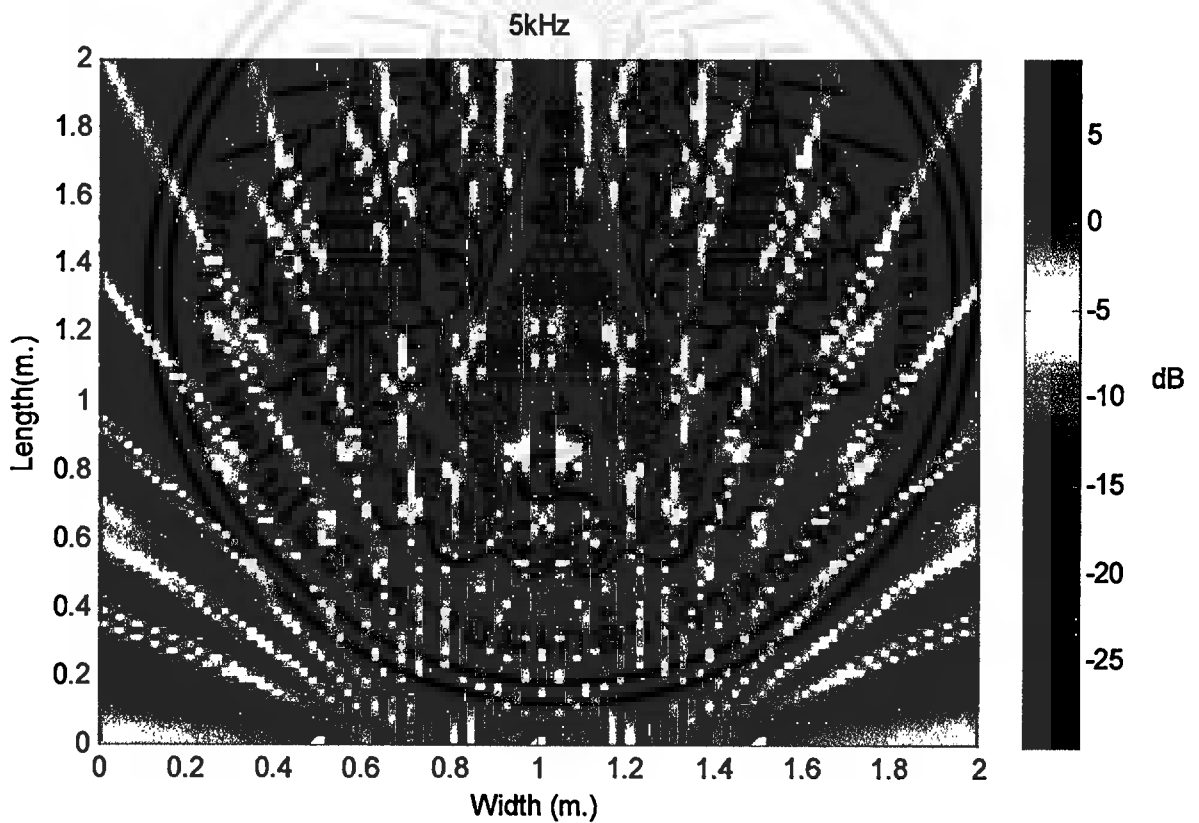
รูป 4.7 จุดรับสัญญาณ 100 จุดที่ความถี่ 5 kHz
