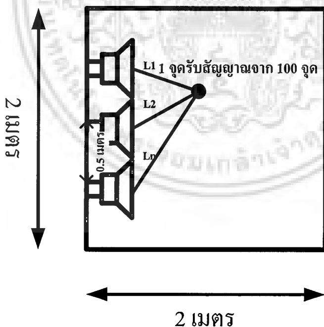
รูป 3.1 การจัดวางลำโพงในพื้นที่ขนาด 2x2 ตารางเมตร
