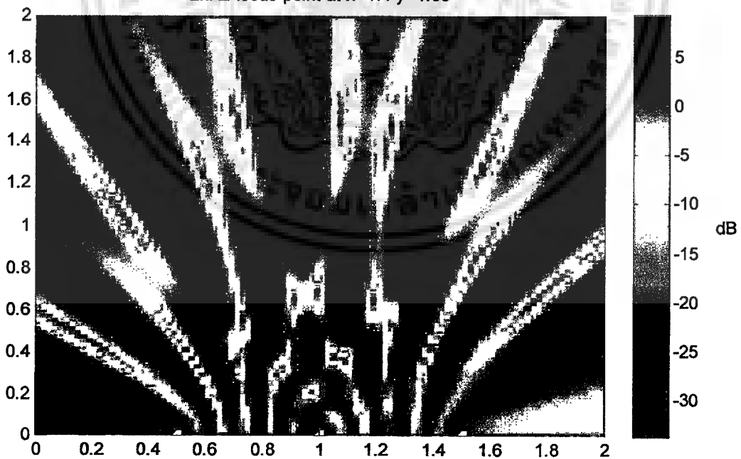
รูป 4.6 จุดโฟกัสที่ x=1.4 เมตร y=1.35 เมตร และความถี่ 2 kHz
