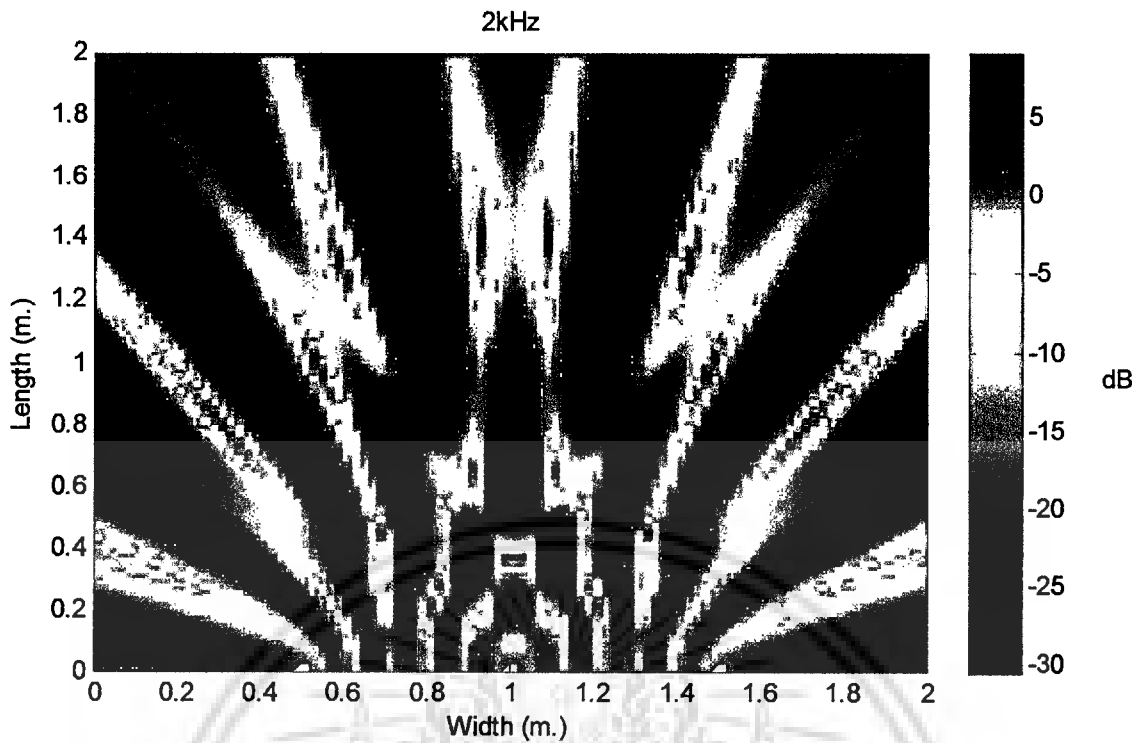
รูป 4.5 จุดรับสัญญาณ 100 จุด ที่ความถี่ 2 kHz
