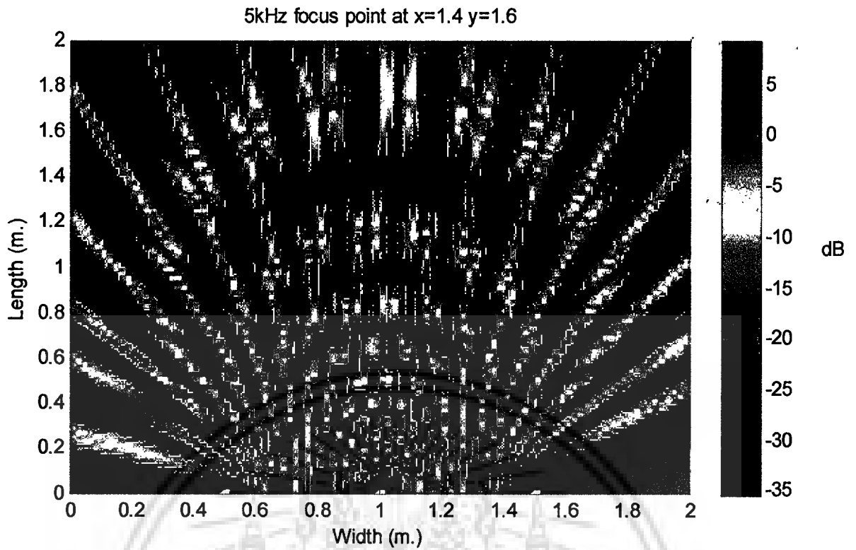
รูป 4.8 จุดโฟกัสที่ x=1.4 เมตร y=1.6 เมตร และความถี่ 5 kHz
