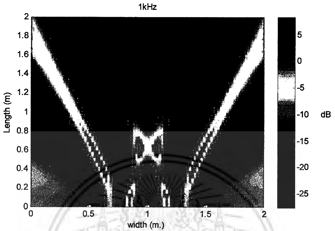
รูป 4.3 จุดรับสัญญาณ 100 จุดที่ความถี่ 1 kHz
