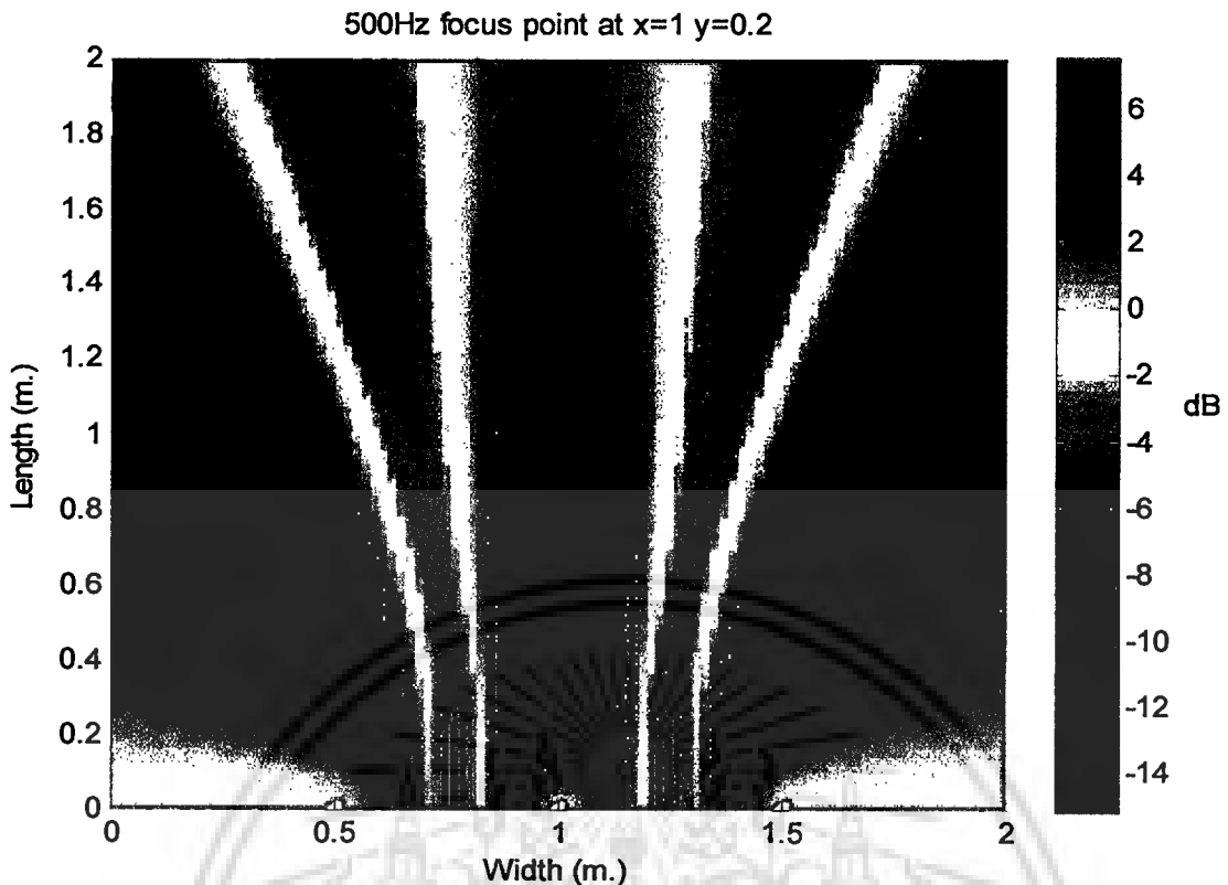
รูป 4.2 จุดโฟกัสที่ x=1 เมตร y=0.2 เมตร และความถี่ 500 Hz
