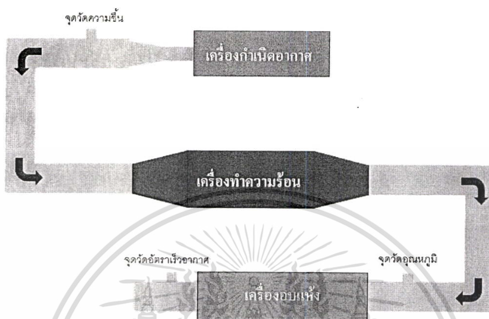
รูปที่ 3.1 แผนภาพเครื่องอบแห้งอุณหภูมิต่ำ
