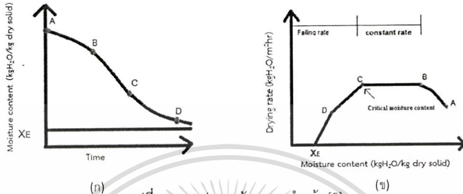
รูปที่ 2.3 กราฟแสดงอัตราการทำแห้ง [5]
