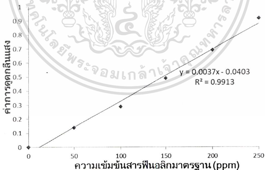
รูปที่ ข.1 กราฟมาตรฐานแสดงค่าการดูดกลืนแสงกับความเข้มข้นสารฟีนอลิกมาตรฐาน
