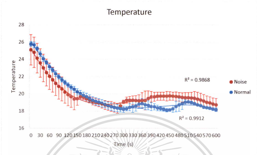
รูปที่ 4.33 กราฟเปรียบเทียบผลการทดลองแสดงอุณหภูมิระหว่างการทำงานปกติกับการมีฝุ่นมีมารบกวนแบบที่ D5
