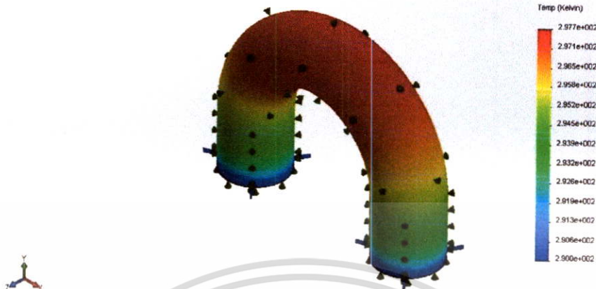
รูปที่ 4.3 ผลการ Simulate มือจับ 2 ข้างแบบที่ 1 เส้นผ่าศูนย์กลาง 2.125 นิ้ว ที่อุณหภูมิ 11 °C
