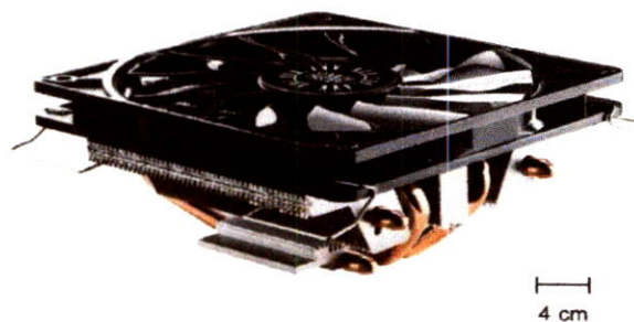
รูปที่ 3.11 Heatsink ของ Cooler Master รุ่น Geminll M4 [16]
