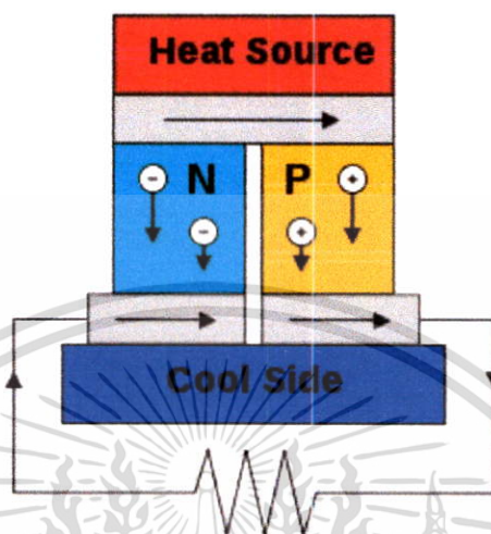
รูปที่ 2.1 ปรากฏการณ์ซีเบค [3]
