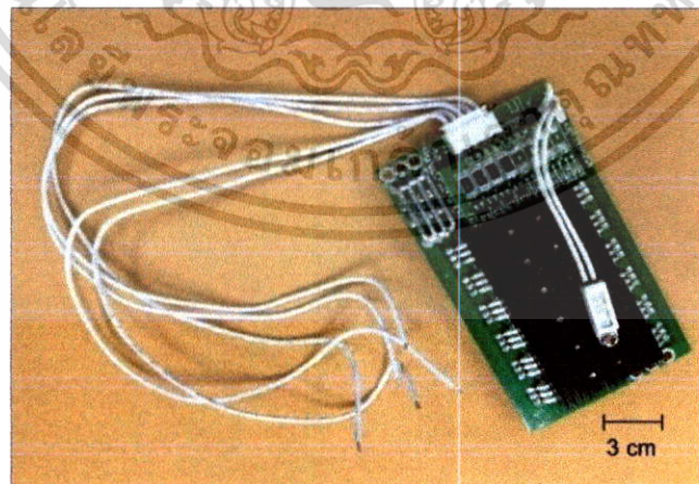
รูปที่ 3.15 แผงวงจร BMS 12.8V 4S LiFePO4 Battery Packs
