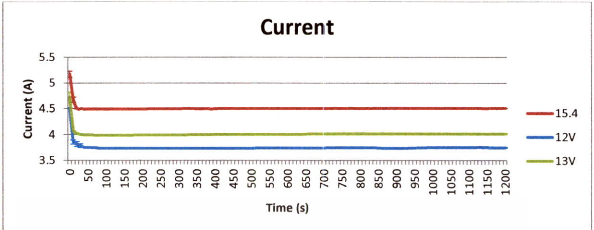
รูปที่ 4.18 กราฟผลการทดลองแสดงกระแสไฟฟ้าที่แรงดัน 12 V, 15.4 V และ 13 V แบบที่ D2
