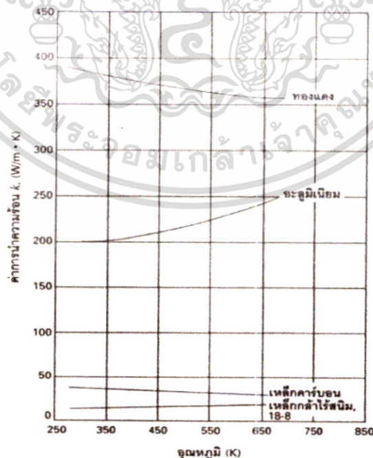
รูปที่ 2.8 ค่าการนำความร้อน k ของโลหะบางชนิดที่แปรตามอุณหภูมิ [7]
