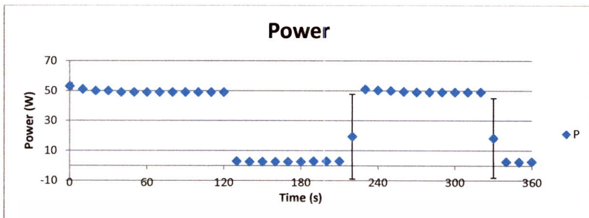
รูปที่ 4.30 กราฟผลการทดลองแสดงกำลังไฟฟ้าที่มีฝ่ามือมารบกววน แบบที่ D4
