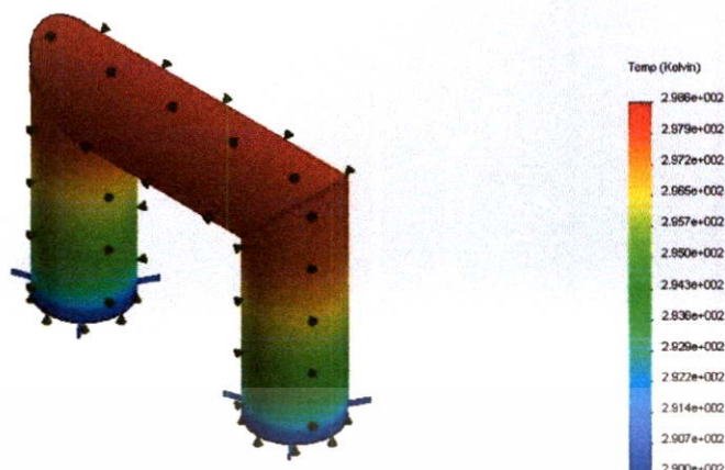
รูปที่ 4.4 ผลการ Simulate มือจับ 2 ข้างแบบที่ 2 เส้นผ่าศูนย์กลาง 2.125 นิ้ว ที่อุณหภูมิ 11 °C
