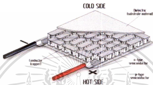
รูปที่ 2.6 ส่วนประกอบของเทอร์โมอิเล็กทริกโมดูล [5]
