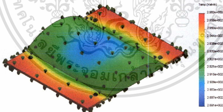
รูปที่ 4.10 ผลการ Simulate มือจับทองแดงแผ่นมีนูนตรงกลาง ที่อุณหภูมิ 16 °C
