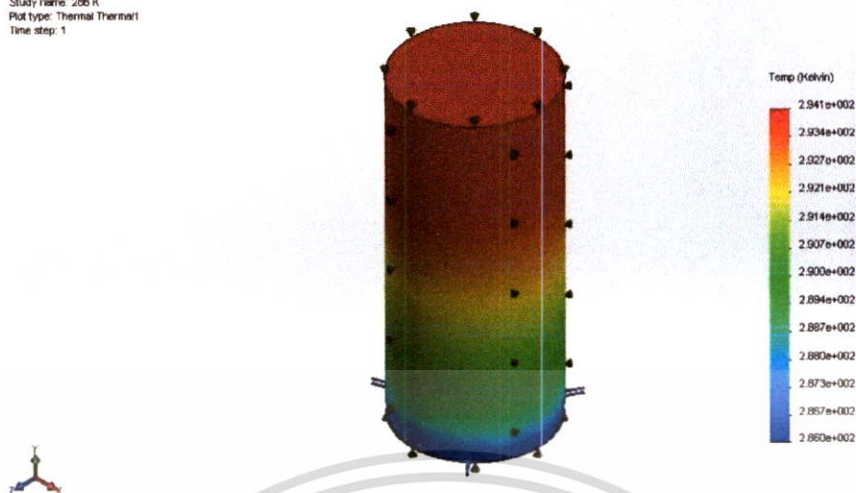
รูปที่ 4.5 ผลการ Simulate มือจับ 1 ซ้าง เส้นผ่าศูนย์กลาง 2.125 นิ้ว ที่อุณหภูมิ 13 °C
