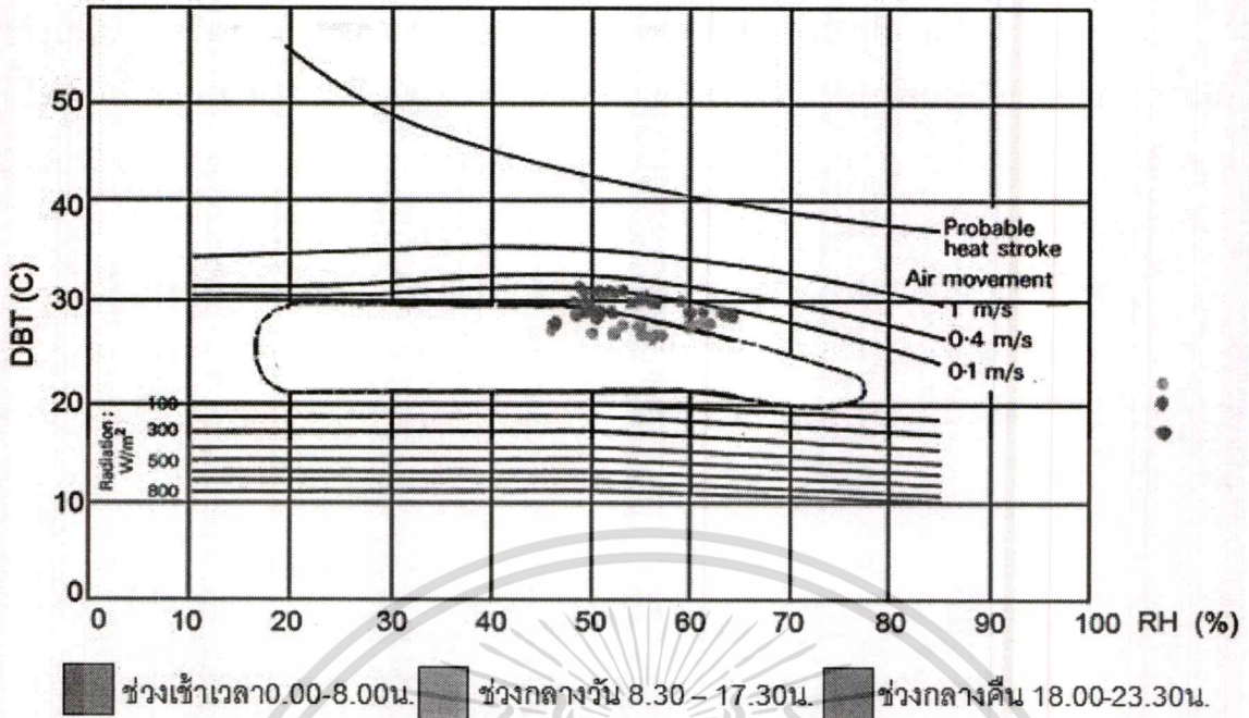
ภาพที่ 4.2 แสดงแผนภูมิไบนโอะโคลเมติกของห้องสตูดิโอฤดูร้อนตามช่วงเวลาของวัน ที่มา: จากการพล็อตค่า, สุภาวดี รัตนมาศ
