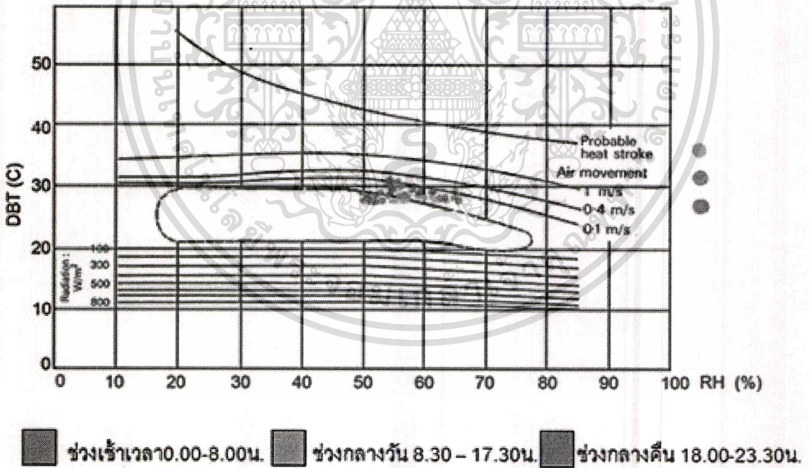
ภาพที่ 4.3 แสดงแผนภูมิไบนโอะโคลเมติกของห้องสตูดิโอฤดูฝนตามช่วงเวลาของวัน
