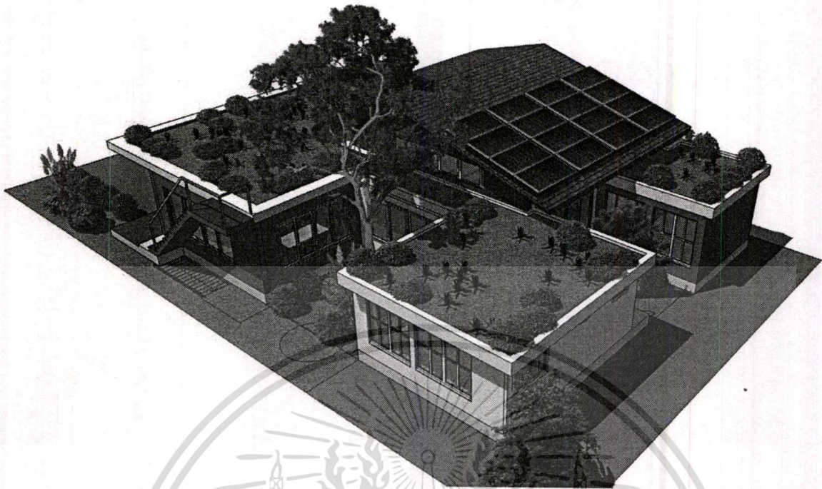
ภาพที่ 5.1 ทศนียภาพรูปแบบบ้านพลังงานแสงอาทิตย์เชิงภูมิอากาศชีวภาพที่ติดตั้งแผงโซลาร์เซลล์ ทำมุม 15 องศาได้พร้อมกรีนรูฟ (หลังคาที่ปลูกพันธุ์ไม้)
