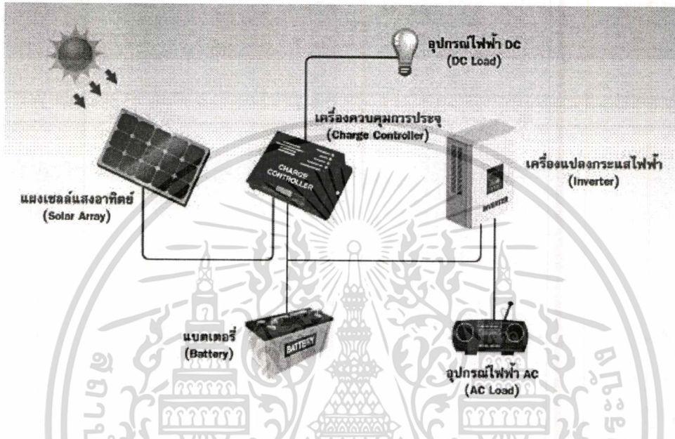
ภาพที่ 2.40 อุปกรณ์สำคัญของระบบการผลิตกระแสไฟฟ้าจากเซลล์แสงอาทิตย์ 42
