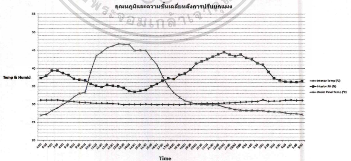
ภาพที่ 4.12 อุณหภูมิในหนึ่งวันหลังปรับยกแผงลอยขึ้น 15 เซนติเมตรจากวัสดุผนังหลังคา
