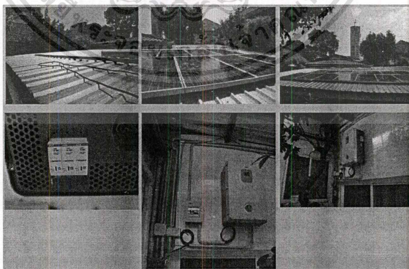
ภาพที่ 3.18 แสดงแผงโซลาร์เซลล์ที่ติดตั้งบนหลังคาด้านทิศเหนือ (แบบ A) อินเวอร์เตอร์และอุปกรณ์ความปลอดภัย
