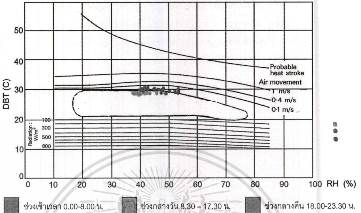
ภาพที่ 3.2 แสดงค่าภาวะสบายภายในห้องนอน เดือนมีนาคม ฤดูร้อน ปี พ.ศ. 2554 ที่มา: สุภาวดี รัตนมาศ และศุทธา ศรีเผด็จ, รายงานวิจัยการพัฒนารูปแบบบ้านพักอาศัย ในเชิงภูมิอากาศชีวภาพเพื่อลดการใช้เครื่องปรับอากาศ, 2554, : 89
