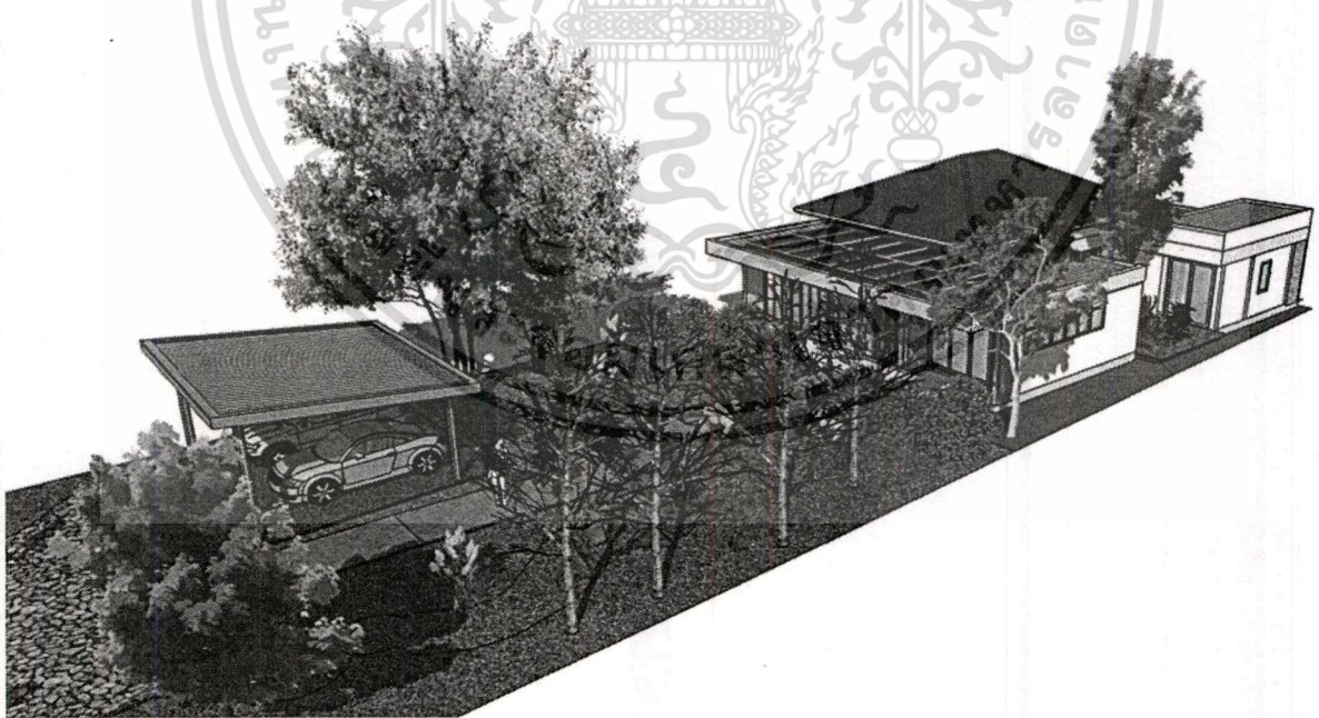
ภาพที่ 2.1 ภาพจำลองบ้านพลังงานแสงอาทิตย์เชิงภูมิอากาศชีวภาพในกรุงเทพมหานคร
