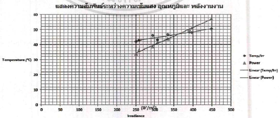
ภาพที่ 4.9 แสดงกราฟค่าพลังงานที่ผลิตได้และค่าอุณหภูมิที่เกิดขึ้นบนแผงโซลาร์เซลล์ในหนึ่งวัน
