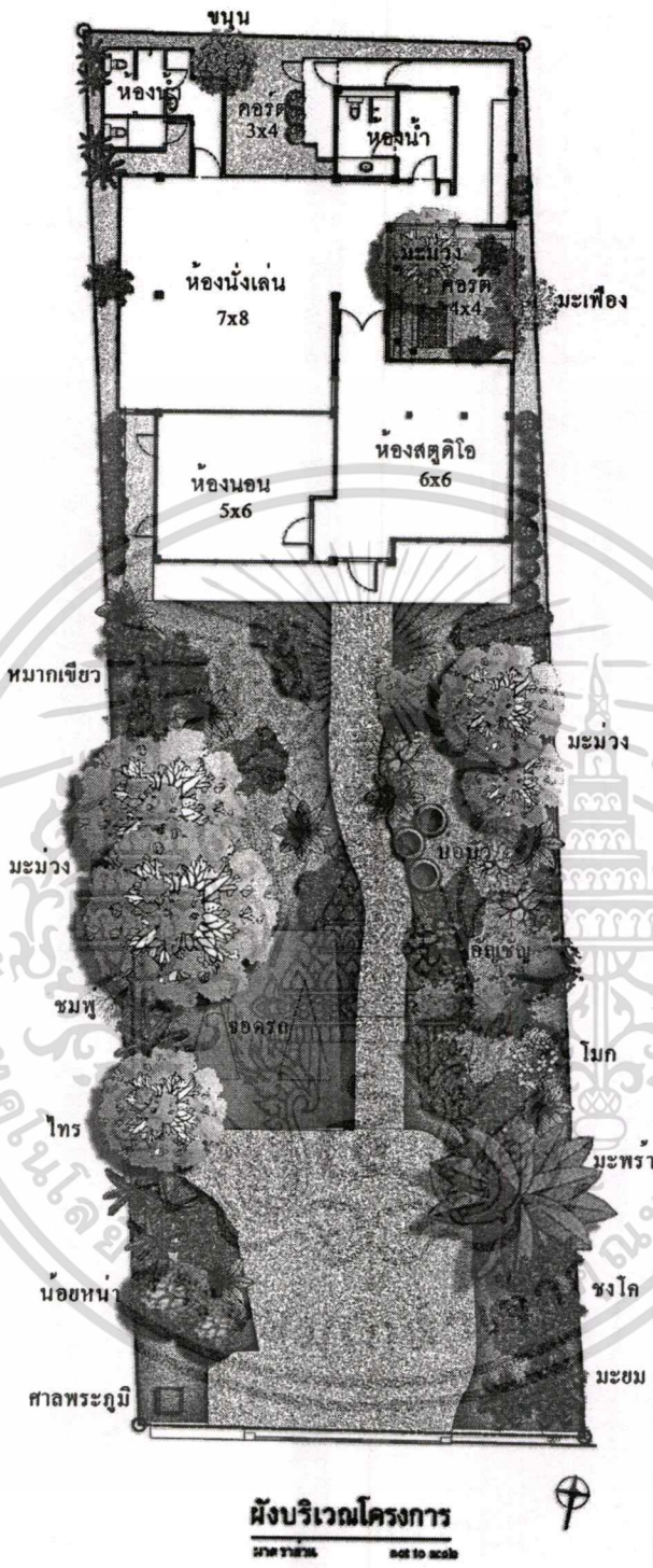
ภาพที่ 3.4 แสดงผังบริเวณบ้านซึ่งรายล้อมด้วยพันธุ์ไม้นานาชนิด มีลานโล่งภายในบ้านและภายนอกบ้าน ทำให้เกิดการระบายอากาศที่ดี ลดอุณหภูมิแวดล้อมลง ทิศเหนือติดถนนซอยพหลโยธิน 19 กว้าง 6.00 เมตร
