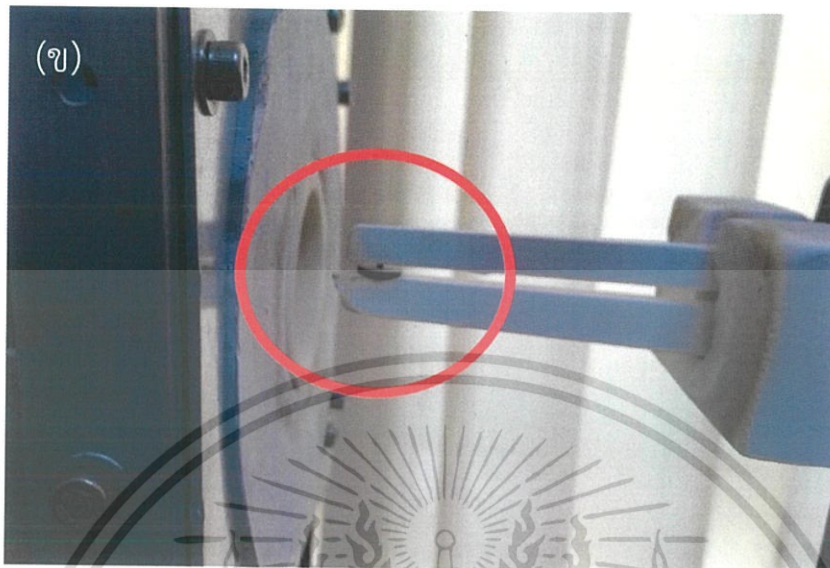
รูปที่ 4.8 (ก) ตัวจับชิ้นงานแบบเก่า และ (ข) ตัวจับชิ้นงานแบบใหม่ที่ผ่านการปรับปรุงแล้ว
