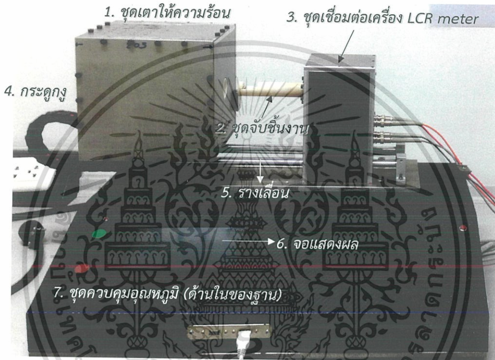
รูปที่ 4.15 (ก) การประกอบชุดเตาให้ความร้อนพร้อมชุดจับชิ้นงานและชุดเชื่อมต่อเครื่อง LCR meter เข้ากับฐานของชุดวัดไดอิเล็กทริก
