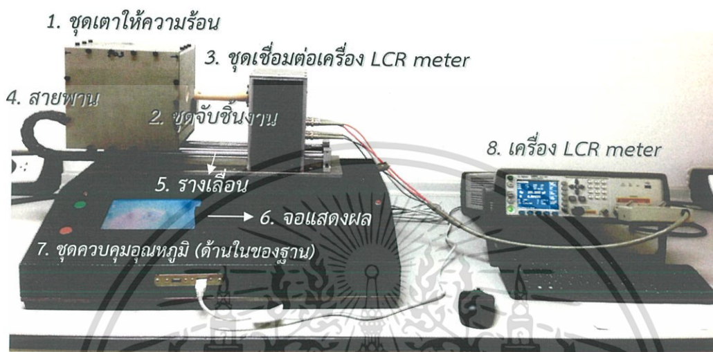
รูปที่ 4.16 ส่วนประกอบของชุดวัดไดโวลีทริกที่เสร็จสมบูรณ์
