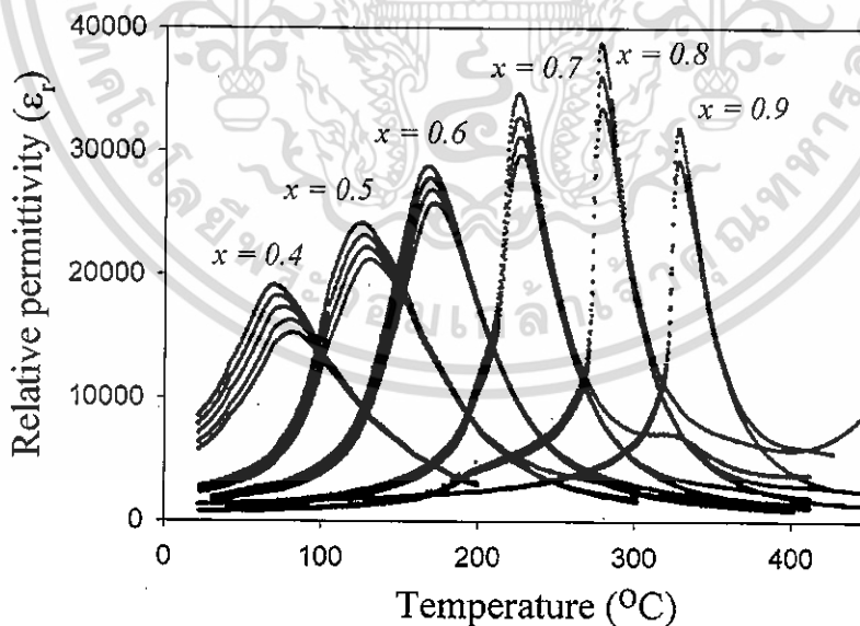
รูปที่ 2.5 แสดงค่าคงที่ไดอิเล็กทริกกับอุณหภูมิของเซรามิก (1-x)\text{PNN}-x\text{PZT}
