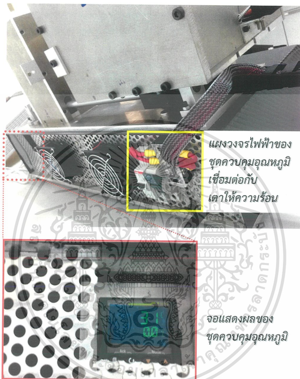
รูปที่ 4.15 (ข) หน้าจอแสดงผลสำหรับชุดควบคุมอุณหภูมิและแผงวงจรไฟฟ้าที่เชื่อมต่อระหว่างชุดควบคุมอุณหภูมิกับเต้าให้ความร้อน
