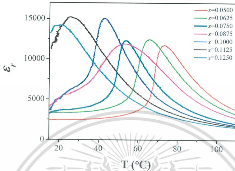
รูปที่ 4.25 ความสัมพันธ์ระหว่างอุณหภูมิการเปลี่ยนแปลงเฟสกับสัดส่วนองค์ประกอบ x ของเซรามิกในระบบ Ba_{0.825+x}Ca_{0.175-x}Ti_{(1-x)}Sn_xO_3
