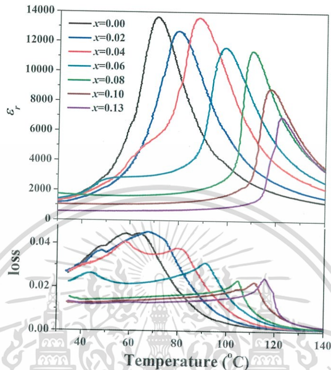
รูปที่ 4.26 ความสัมพันธ์ระหว่างค่าคงที่ไดอิเล็กทริกและค่าประกอบการสูญเสียไดอิเล็กทริกกับอุณหภูมิของเซรามิก 0.87BT-(0.13-x)BZ-xCT
