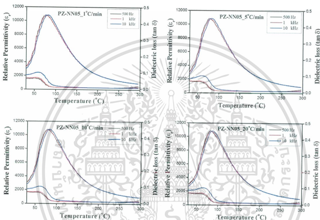
รูปที่ 4.19 กราฟความสัมพันธ์ระหว่างค่าสภาพยอมสัมพัทธ์ ค่าการสูญเสียทางไดอิเล็กทริกและอุณหภูมิของสารตัวอย่างมาตรฐาน PZ-NN โดยทำการวัดที่อัตราการขึ้นลงของอุณหภูมิเท่ากับ 1 5 10 และ 20 °C/นาที
