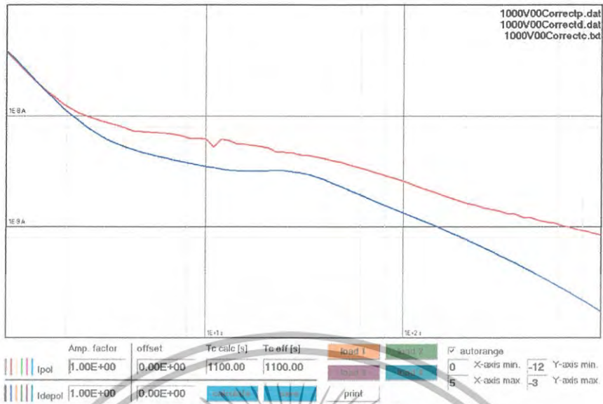
รูปที่ ค.17 กราฟของกระแสไฟฟ้าแรงดันและดีโพลาร์เซชันที่ได้จากการทดสอบหลังจากทำการปรับแก้ค่าแล้ว
