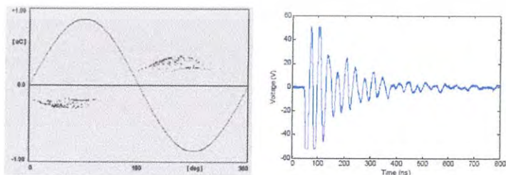
รูปที่ 2.30 ผลของดีสซาร์จเนื่องจากการเชื่อมชิ้นส่วนโลหะไม่แน่น
