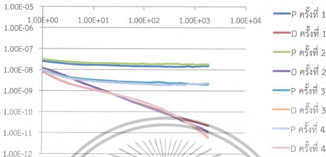
รูปที่ 4.9 กราฟกระแสโพลาร์ไรเซชันและดีโพลาร์ไรเซชันกับเวลาของบัสซึ่ง 33 kV หุ้มฟลอยด์ 2 ใน 3 ส่วน
