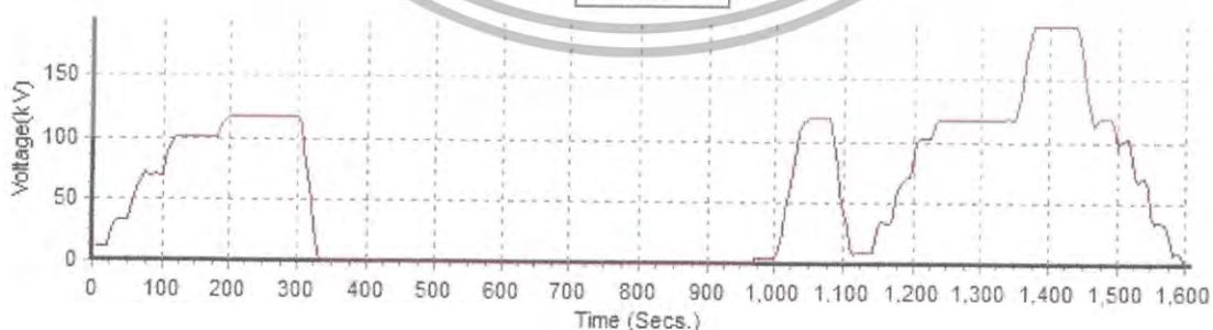
รูปที่ 4.17 การทดสอบการเกิดดีสชาร์จบางส่วนของบุชชิ่ง Bushing7
