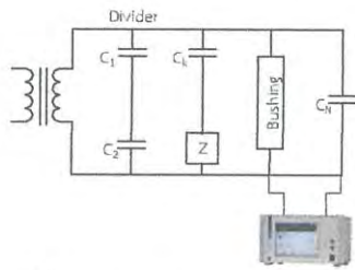
รูปที่ 1 วงจรทดสอบดิสชาร์จบางส่วน
