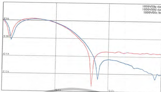
รูปที่ 4.26 การทดสอบกระแสไฟลาระเซชันและดีไฟลาระเซชันของบุชชิ่ง Bushing2
