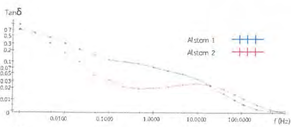
รูปที่ X ผลการทดสอบแฟกเตอร์กำลังสูญเสีย (tanδ) ที่ความถี่ต่างๆ
