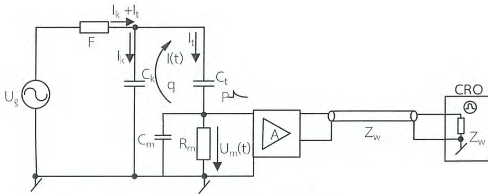
รูปที่ 2.14 วงจรพื้นฐานการวัด PD
