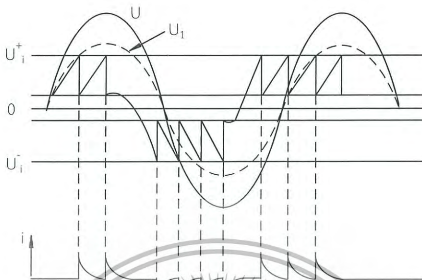
รูปที่ 2.12 ทิสซาร์จภายในเมื่อเปลี่ยนแรงดันกระแสสลับ
