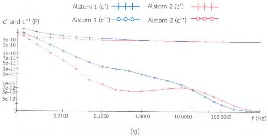
รูปที่ 4.33 กราฟการทดสอบความเป็นอนวนในรูปแบบโดเมนความถี่(FDS) ระหว่าง Alstom1 กับ Alstom2
