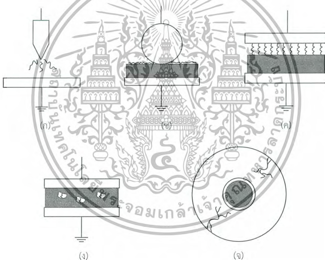
รูปที่ 2.9 รูปแบบของดีสชาร์จบางส่วน (PD) แบบต่างๆ (ก) โคโรนาดีสชาร์จ (ข) ดีสชาร์จตามผิว (ค) ดีสชาร์จภายในรอยต่อ (ง) ดีสชาร์จภายในโพรงก๊าซ (จ) ดีสชาร์จภายในมีสิ่งแปลกปลอม
