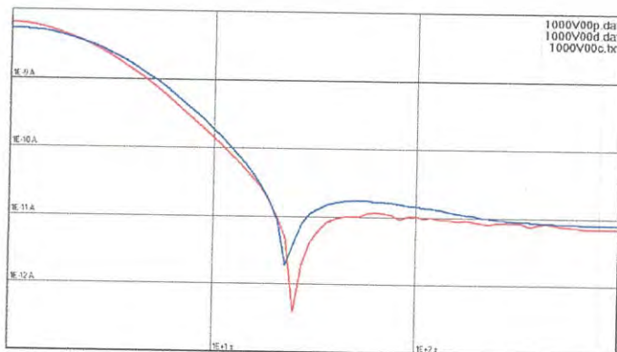
รูปที่ 4.28 การทดสอบกระแสไฟลาระเซชันและดีไฟลาระเซชันของบุชชิ่ง Bushing4
