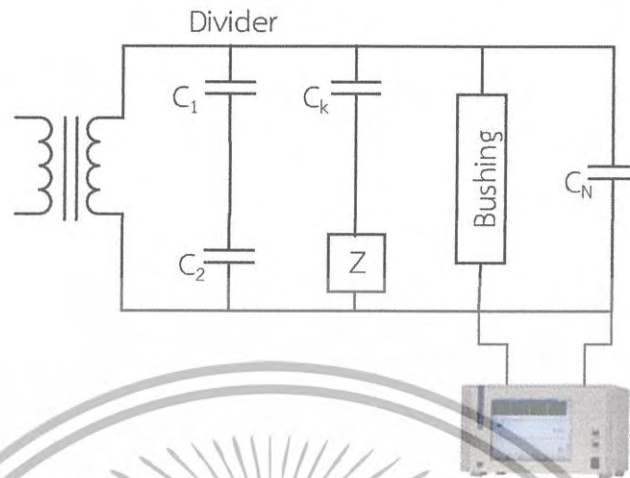
รูปที่ ข.9 วงจรการวัดแพคเตอร์กำลังสูญเสีย
