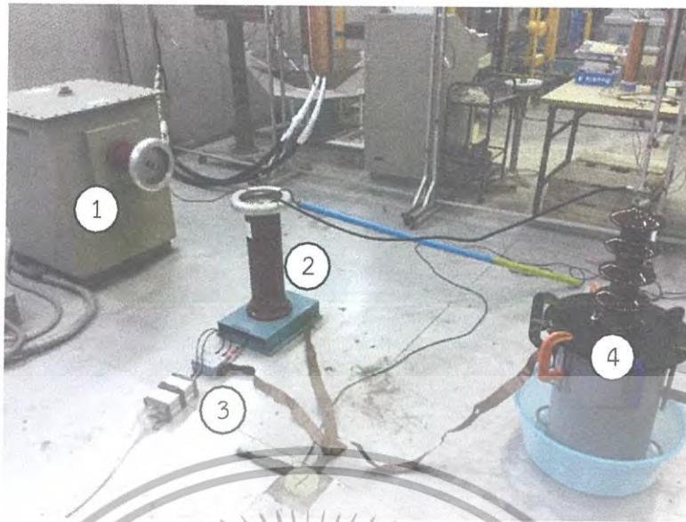
รูปที่ 3.17 การต่อวงจรทดสอบดีสชาร์จบางส่วน
