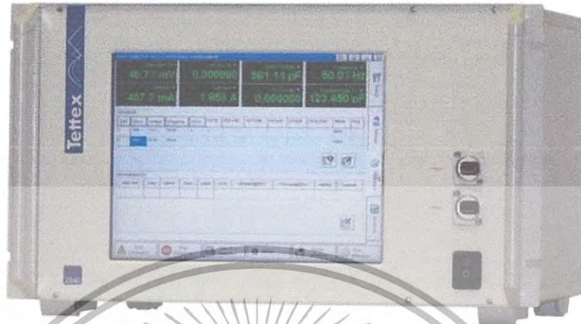
รูปที่ ข.1 เครื่อง Tettex 2840 High Precision C and Tan \delta Measuring Bridge
