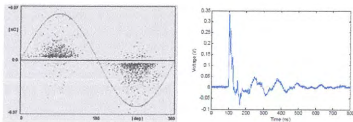
รูปที่ 2.27 ผลของดีสซาร์จเนื่องจากฟองอากาศในน้ำมัน
