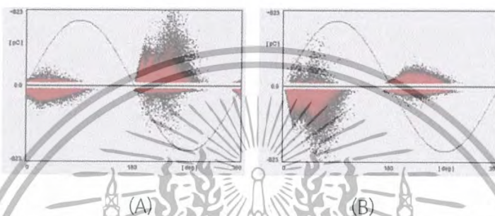
รูปที่ 2.24 รูปแบบการเกิดดีสชาร์จตามผิวบนผิวของฉนวนไมก้า A) High Voltage เชื่อมเข้ากับด้านบนของอิเล็กทรอนิกส์ B) High Voltage เชื่อมเข้ากับแผ่นทองแดงที่มีขอบแหลม
