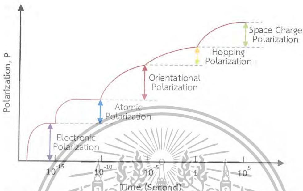
รูปที่ 2.33 ระยะเวลาที่ใช้ในการเกิดโพลาไรเซชันทั้ง 5 แบบภายใต้การป้อนแรงดันรูปขั้น
