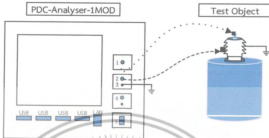
รูปที่ ค.3 วงจรการทดสอบกระแสไหลเวียนและดิฟเฟอเรนเชียล
