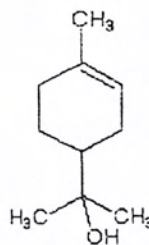
\alpha -Terpineol
