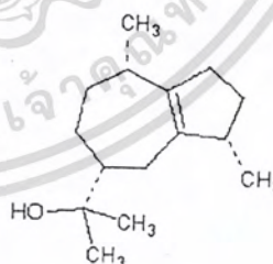
Guaiol
