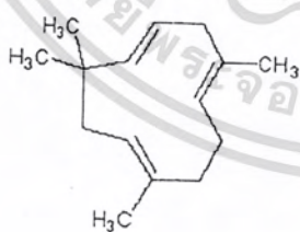
Humulene
