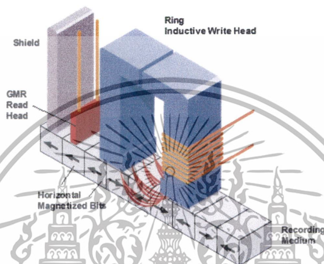
รูปที่ 2.3 รูปแบบการบันทึกข้อมูลแนวอน [10]
