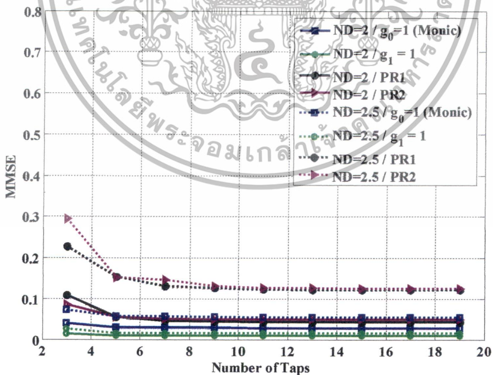
รูปที่ 4.3 ผลเปรียบเทียบค่า MMSE กับจำนวนแท็ปของอีควอลไลเซอร์ในช่องสัญญาณที่เป็นเชิงเส้น
