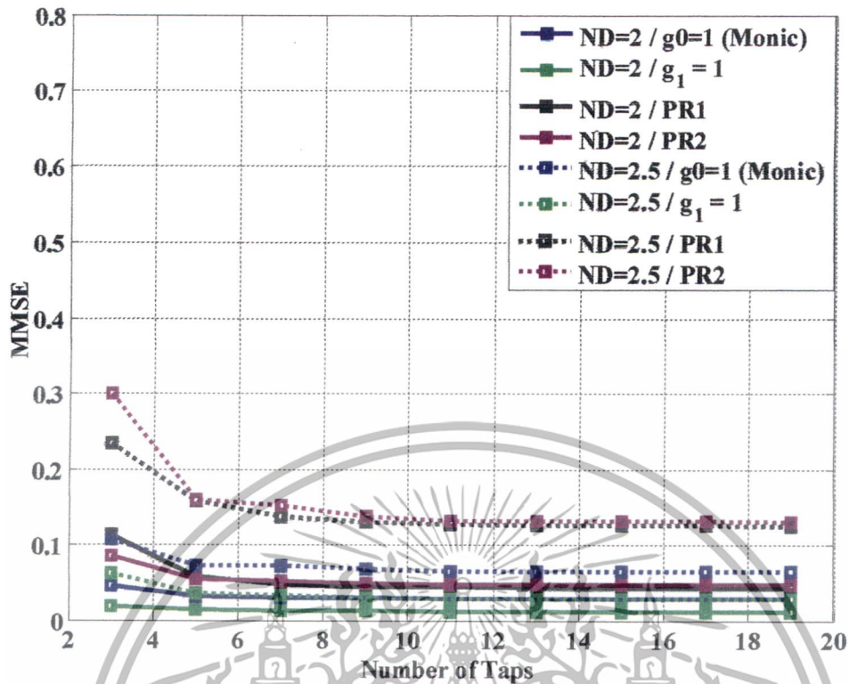
รูปที่ 4.2 ผลเปรียบเทียบค่า MMSE กับจำนวนแท็ปของอีควอลไลเซอร์ในช่องสัญญาณที่เป็นเชิงเส้น เมื่อทาร์เก็ตมีความยาวเท่ากับ 3
