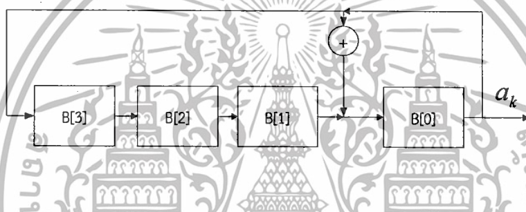
รูปที่ 2.22 วงจรถ่ายข้อมูลแบบย้อนกลับที่สร้างจากสมการพหุนาม h(x)=1+x+x^4
