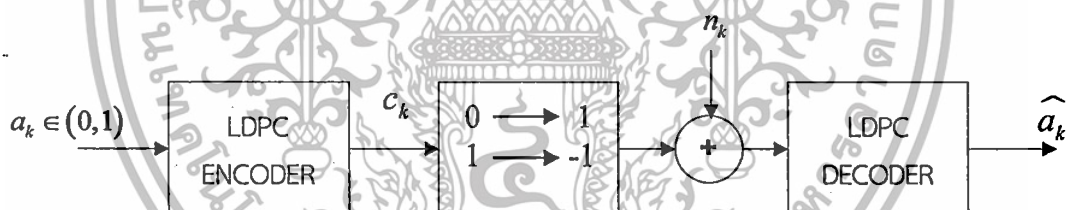
รูปที่ 2.26 การเข้ารหัสและถอดรหัสแอลดีพีซีในช่องสัญญาณรบกวนเกาส์เซียนขาวบวก
