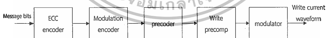
รูปที่ 2.10 แผนภาพกระบวนการเขียนข้อมูล
