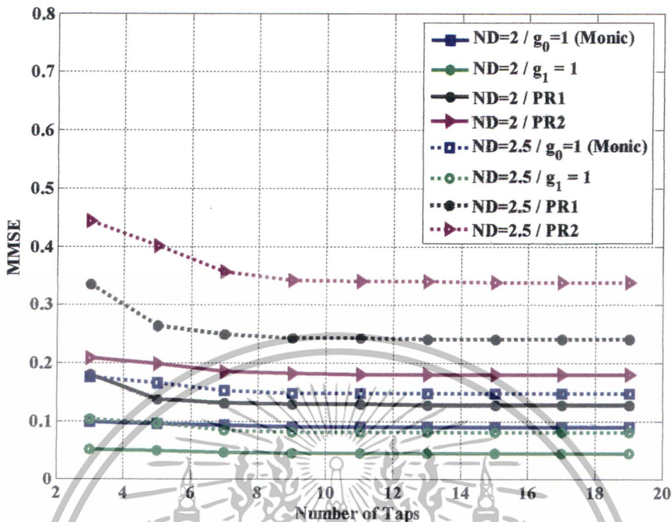
รูปที่ 4.5 ผลเปรียบเทียบค่า MMSE กับจำนวนแท็ปของอีควอไลเซอร์ในช่องสัญญาณไม่เป็นเชิงเส้น เมื่อความยาวของทาร์เกิดเท่ากับ 3
