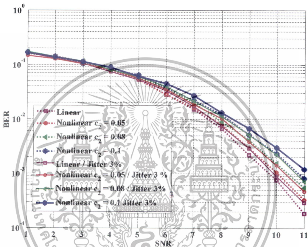
รูปที่ 4.14 อัตราบิดผิดพลาดของระบบที่เป็นเชิงเส้นและไม่เป็นเชิงเส้นที่ได้รับผลกระทบจากสัญญาณรบกวนเกาส์เซียนขาวแบบบวก กับระบบที่ได้รับผลกระทบทั้งสัญญาณรบกวนเกาส์เซียนขาวแบบบวกและสัญญาณรบกวนสื่อบันทึกที่ระดับ 3%
