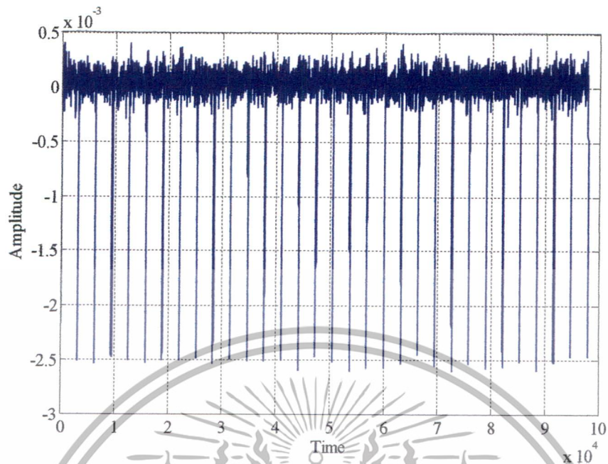
รูปที่ 3.7 สัญญาณสหสัมพันธ์แบบไขว้ของสัญญาณอ่านกลับที่มีการสุ่มตัวอย่างเกินและลำดับสุ่มเทียม
