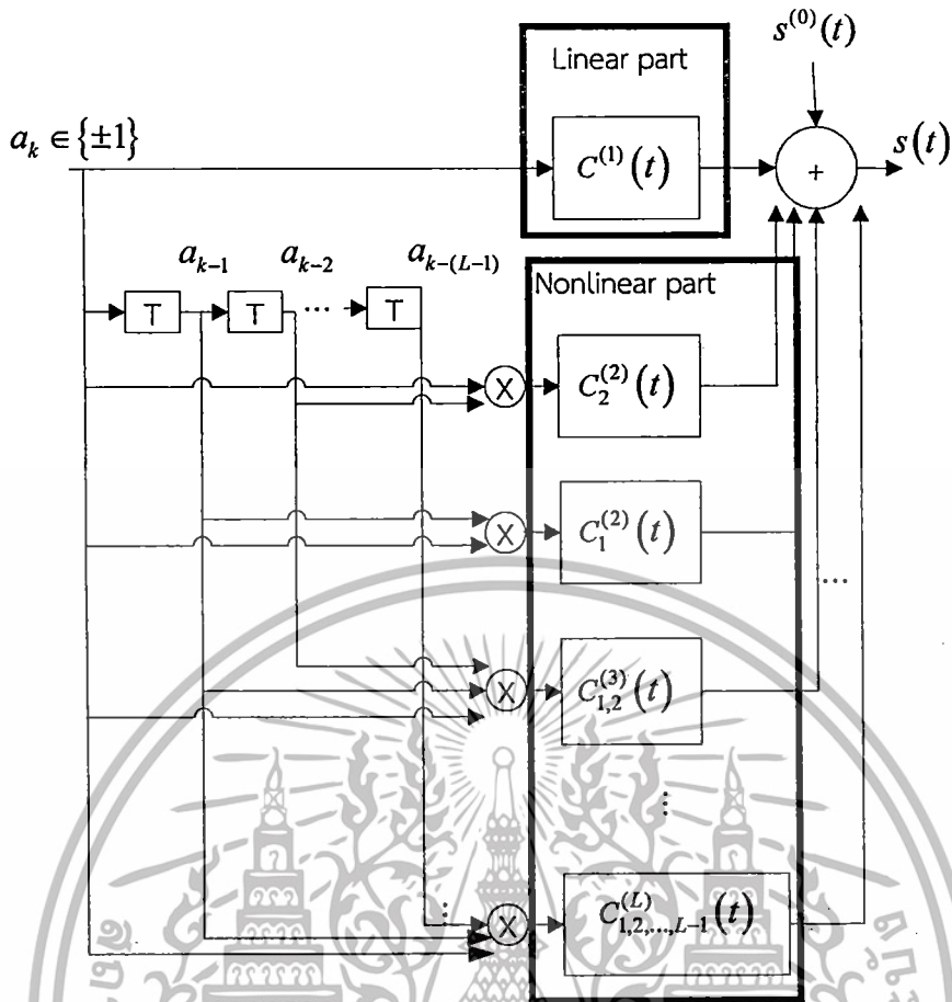
รูปที่ 2.20 แบบจำลองโวลเทราสำหรับช่องสัญญาณที่ไม่เป็นเชิงเส้น
