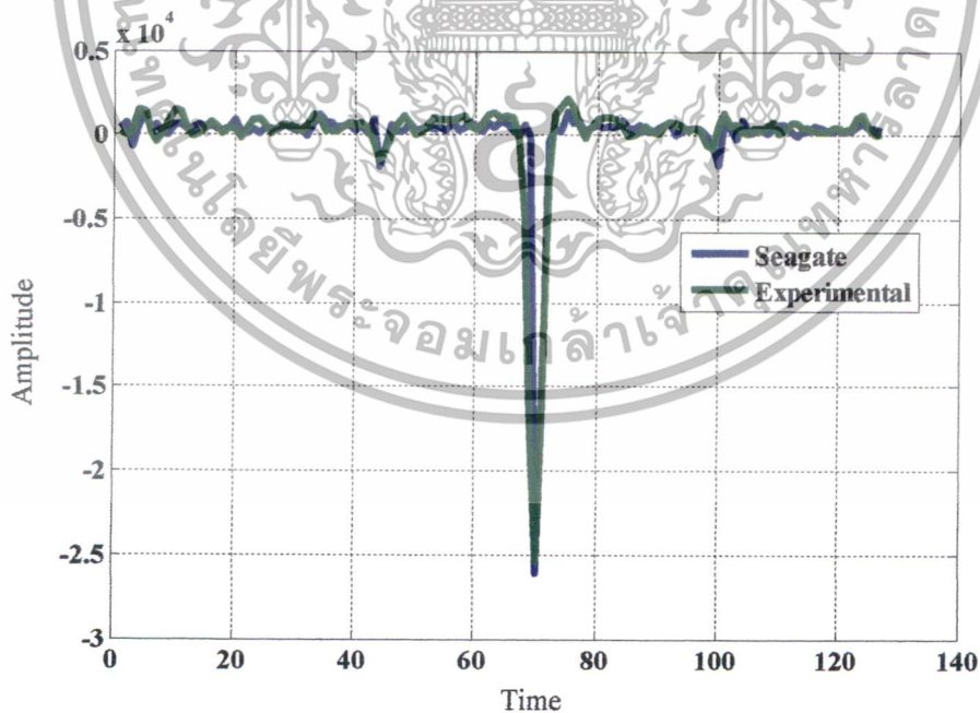
รูปที่ 3.8 สัญญาณพัลส์เดบิตของสัญญาณ 1 คาบ
