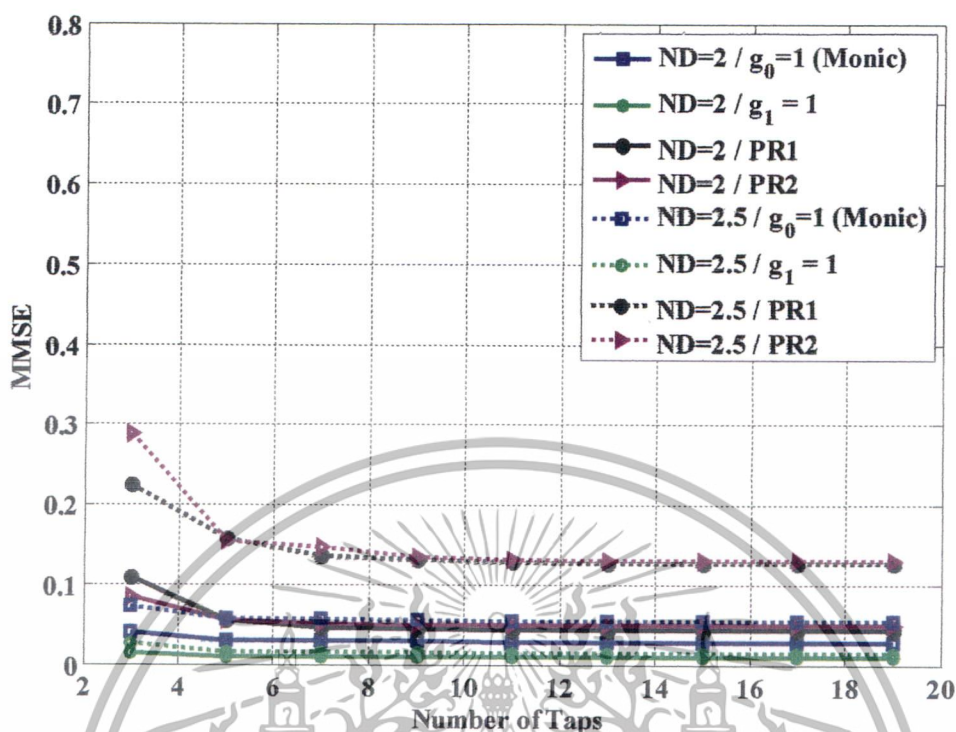
รูปที่ 4.4 ผลเปรียบเทียบค่า MMSE กับจำนวนแท็ปของอีควอไลเซอร์ในช่องสัญญาณที่เป็นเชิงเส้น เมื่อความยาวของทาร์เก็ตเท่ากับ 7
