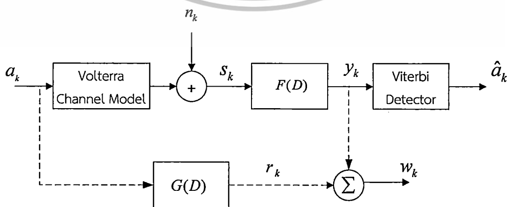
รูปที่ 4.1 แบบจำลองสำหรับการออกแบบทาร์เก็ตด้วยวิธี MMSE
