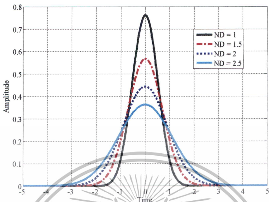
รูปที่ 2.14 ผลตอบสนองโดบิต สำหรับการบันทึกข้อมูลแบบแนวตั้ง [1]
