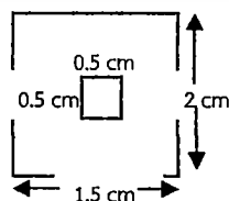
รูปที่ 3.2 ขั้วไฟฟ้าทำงาน
