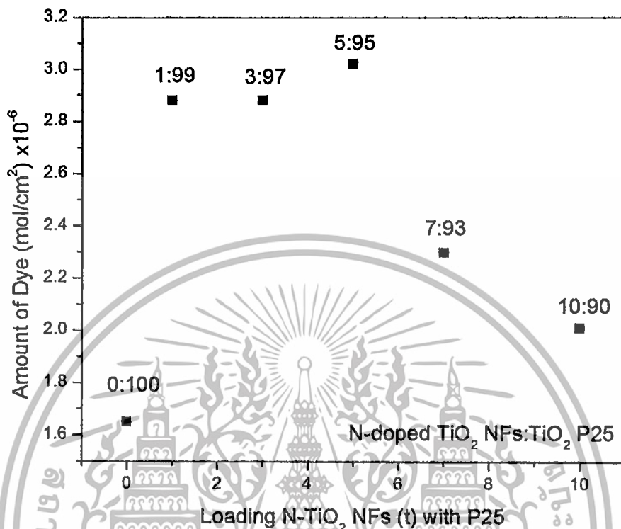
รูปที่ 4.34 การวิเคราะห์ความสัมพันธ์ค่าการดูดกลืนของสีย้อมบนขั้วนำไฟฟ้า กับปริมาณการผสมของเส้นใยไทเทเนียมไดออกไซด์ ที่เจือด้วยธาตุไนโตรเจน 3% กับไทเทเนียมไดออกไซด์ P25
