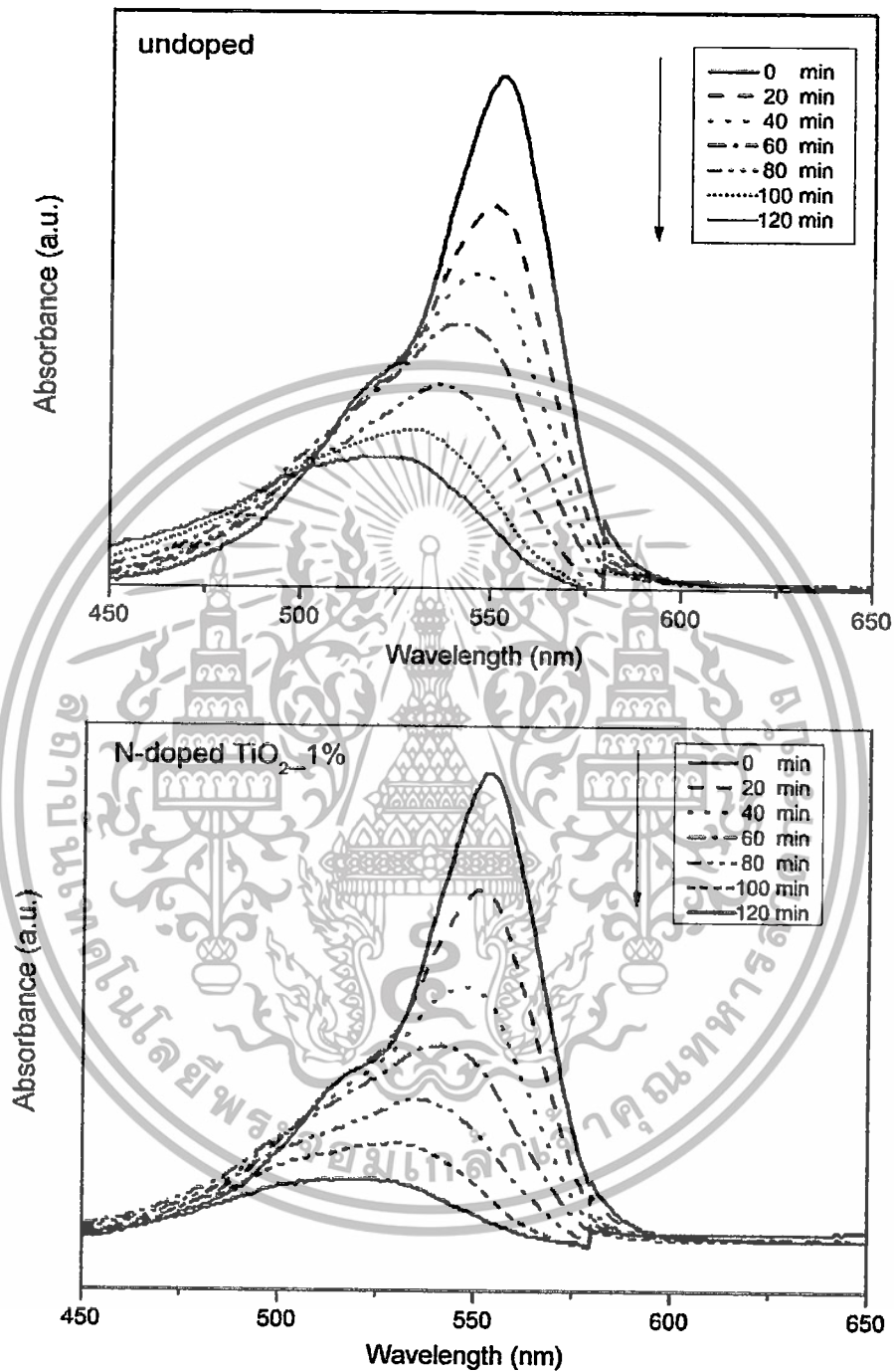
รูปที่ 4.26 กราฟการวิเคราะห์กระบวนกรดูดกลืนแสง ในการย่อยสลายสีย้อม RhB ด้วยเครื่อง UV-Vis Spectroscopy ของเส้นใยนาโนไทเทเนียมไดออกไซด์ ภายใต้เงื่อนไขปริมาณการเจือด้วยธาตุไนโตรเจนที่ 0%, 1%, 3% และ 5% โดยน้ำหนัก ที่เวลา 0, 20, 40, 60, 80, 100 และ 120 นาที
