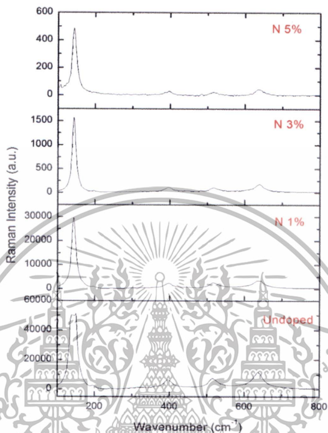
รูปที่ 4.9 กราฟวิเคราะห์โครงสร้างด้วยเทคนิครามานสเปกโตรสโกปี ของเส้นใยนาโนไทเทเนียมไดออกไซด์ ภายใต้เงื่อนไขการเปลี่ยนแปลงปริมาณการเจือธาตุไนโตรเจน ที่ 0%, 1%, 3% และ 5% โดยน้ำหนัก
