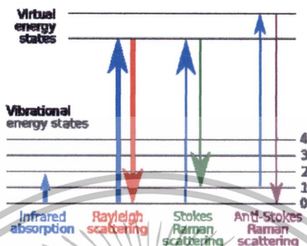
รูปที่ 2.14 การกระเจิงแบบรามาน
