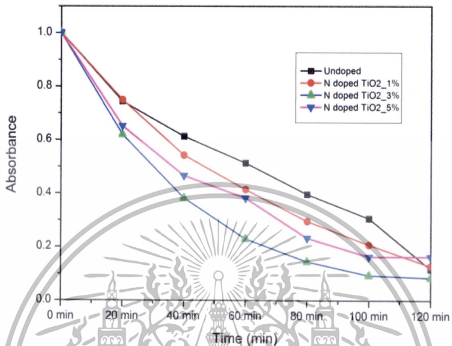
รูปที่ 4.27 กราฟการวิเคราะห์อัตราการเร่งปฏิกิริยาด้วยแสง ของเส้นใยนาโนไทเทเนียมไดออกไซด์ ภายใต้เงื่อนไขการเปลี่ยนแปลงปริมาณการเจือธาตุไนโตรเจน ที่ 0%, 1%, 3% และ 5% โดยน้ำหนัก เทียบกับเวลาที่ 0, 20, 40, 60, 80, 100 และ 120 นาที
