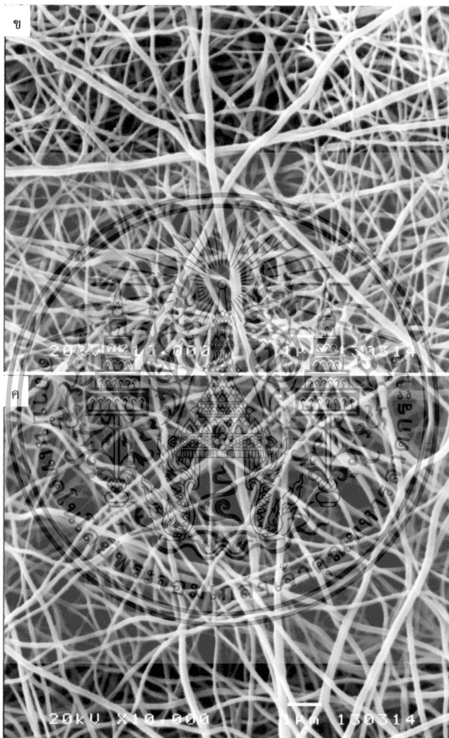
รูปที่ 4.10(ต่อ) ภาพถ่ายทางพื้นผิวของเส้นใยไทยเหนียวไดออกไซด์ ที่เจือด้วยธาตุไนโตรเจนด้วยกลีอง จุลทรรศน์อิเล็กตรอนแบบเลือนกราด ภายใต้เงื่อนไขการเปลี่ยนแปลงปริมาณการเจือธาตุไนโตรเจนที่ (ก) 1% (ข) 3% และ (ค) 5% โดยน้ำหนัก
