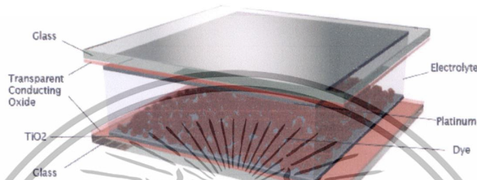
รูปที่ 2.8 ส่วนประกอบของเซลล์แสงอาทิตย์ชนิดสีย้อมไวแสง [11]
