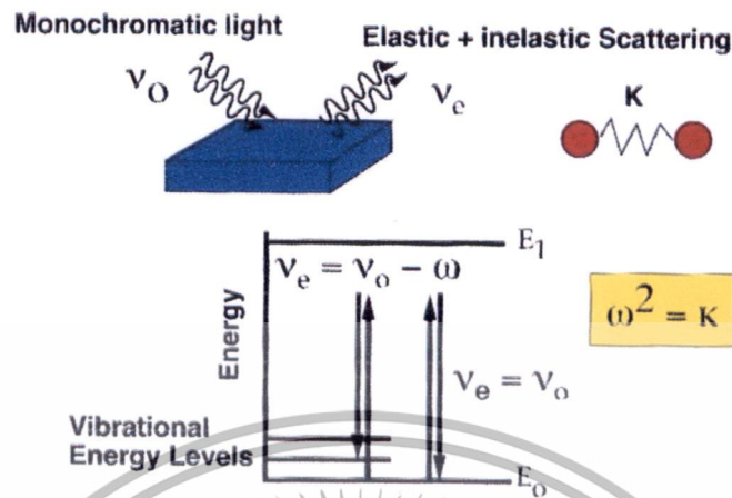
รูปที่ 2.15 แผนภาพการทำงานของรามานสเปกโตรสโกปี
