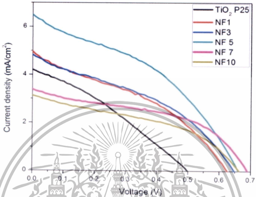
รูปที่ 4.33 กราฟการวิเคราะห์ประสิทธิภาพของขั้วทำงาน ของเส้นใยนาโนไทเทเนียมไดออกไซด์ ที่เจือด้วยธาตุไนโตรเจน3%ผสมกับไทเทเนียมไดออกไซด์P25 ในอัตราส่วน 0:100, 1:99, 3:97, 5:95, 7:93 และ 10:90
