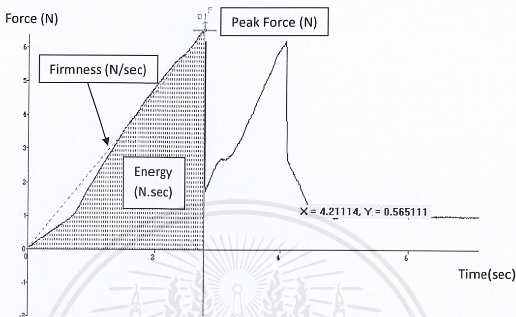
รูปที่ 3.9 กราฟความสัมพันธ์ของแรงและเวลาที่ได้จากการทดสอบแบบหั่วเจาะทรงกระบอก
