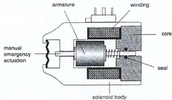
รูป 2.8 ขดลวดโซลินอยด์ชนิดแห้ง (Dry solenoid)
