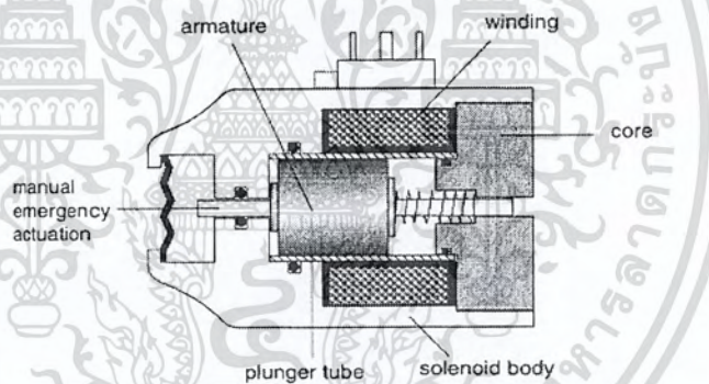
รูป 2.7 ขดลวดโซลินอยด์ชนิดเปียก (Wet solenoid)
