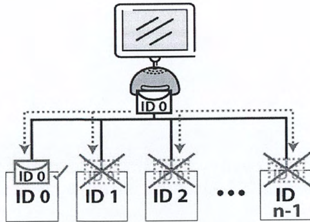
รูป 3.9 การส่งข้อมูลด้วย Bus topology โดยไม่เจาะจงผู้รับ
