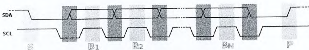
รูป 2.20 ไตอะแกรมเวลาแสดงสถานะต่างๆ ในบัส I 2 C
