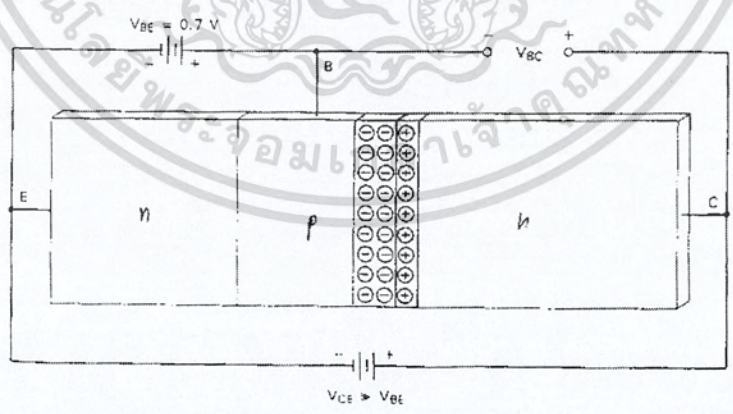
รูป 2.13 การต่อแหล่งจ่ายไฟฟ้าให้ทรานซิสเตอร์ทำงานในบริเวณอิมิตัว
