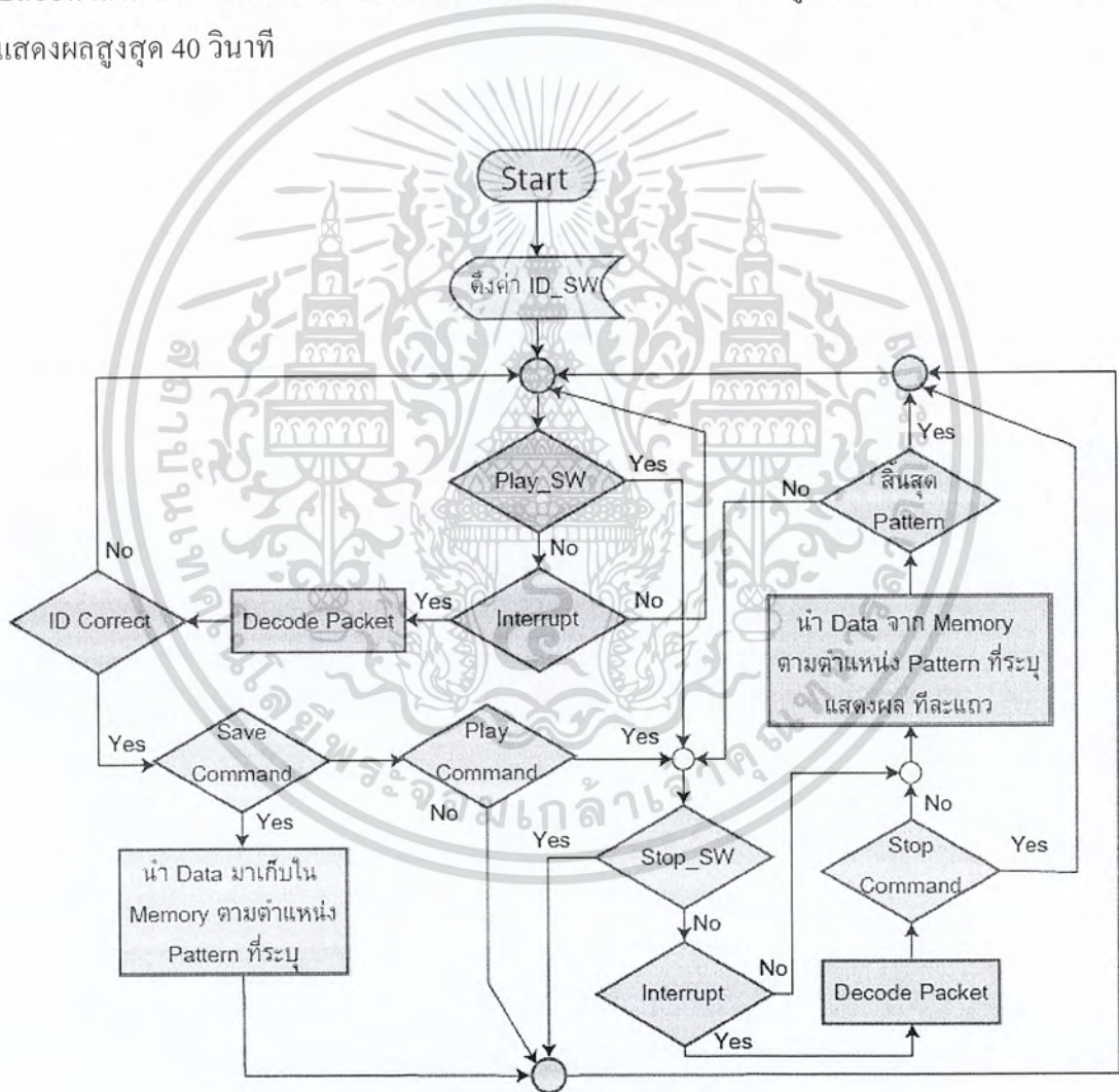
รูป 3.4 การทำงานของชุดแสดงผล
