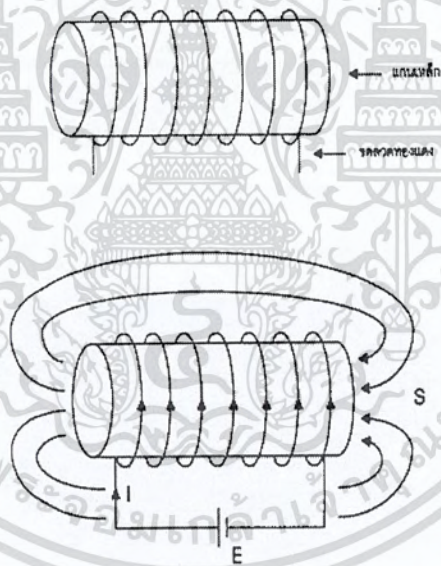
รูป 2.5 ขดลวดโซลินอยด์
