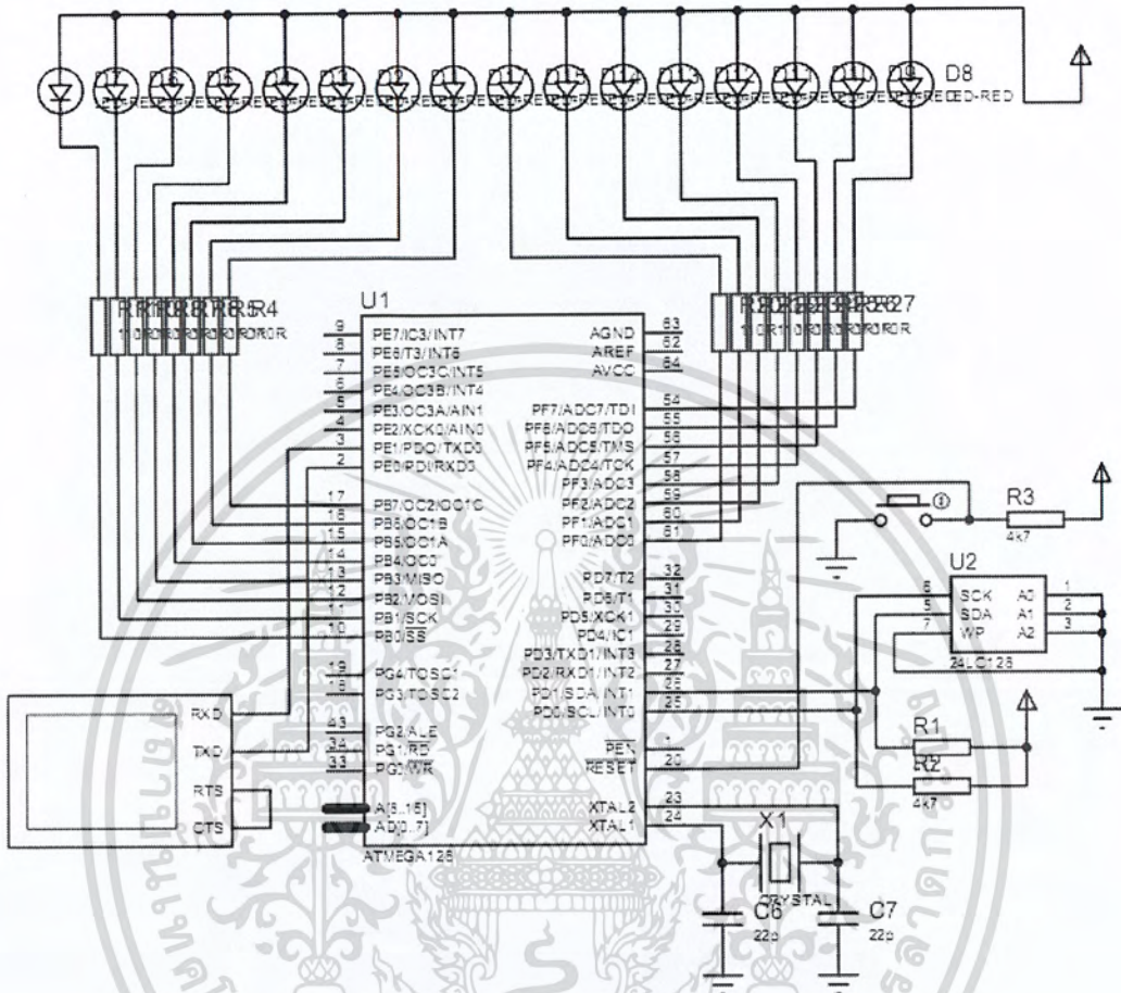
รูป 4.6 วงจรที่เชื่อมต่ออีมูมิออนเข้ากับ ATmega128
