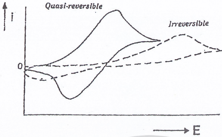
รูปที่ 2.28 ไชคลิก โวลแทม โมแกรมของปฏิกิริยาที่ผันกลับไม่ได้ และผันกลับได้ไม่สมบูรณ์
