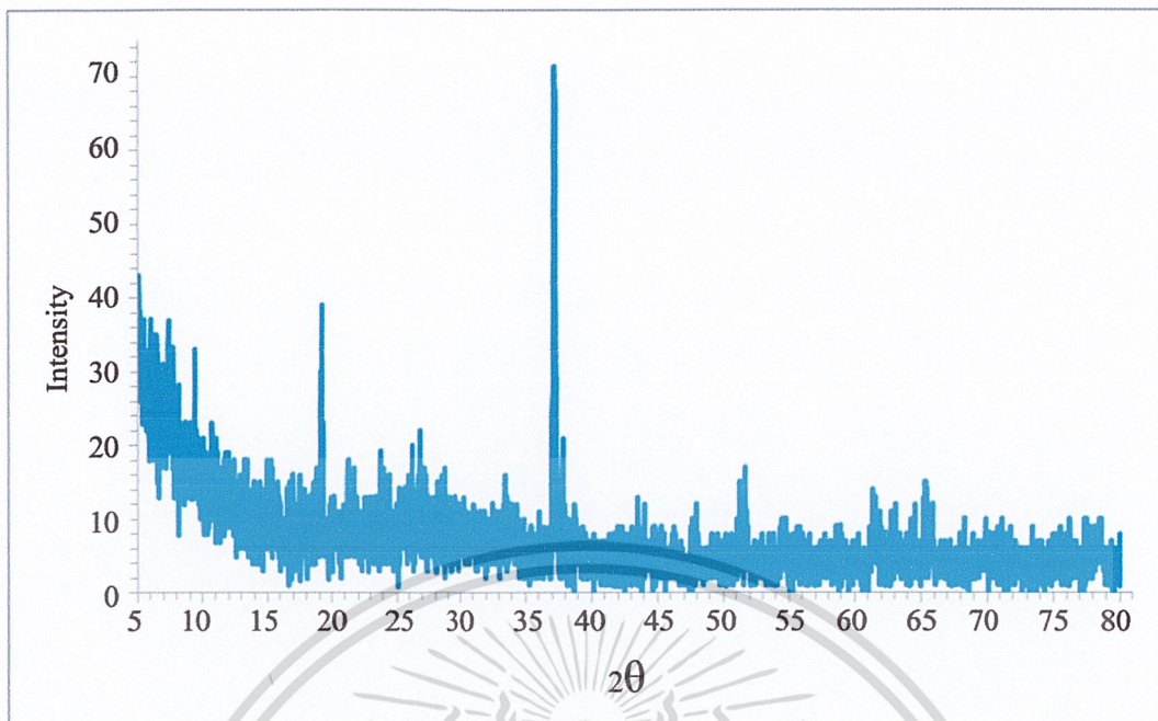
รูปที่ 4.5 กราฟจากเครื่องเอกซเรย์ดิฟแฟรคโทมิเตอร์ของขั้วไฟฟ้าทินออกไซด์เจือฟลูออรีน
