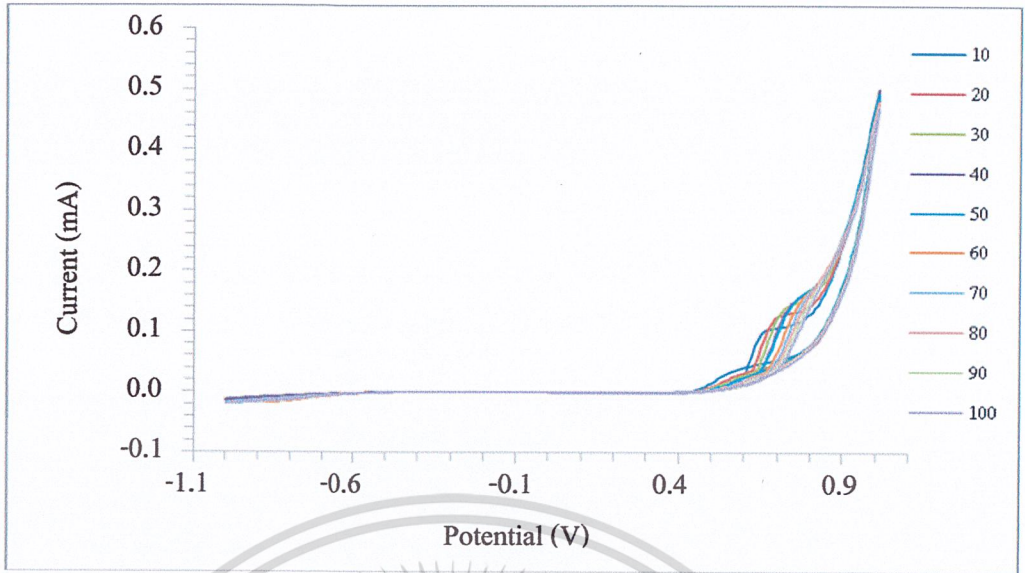
รูปที่ 4.12 ไชคติกโวลแทมโมแกรมของการตรวจวัดไฮโดรเจนเปอร์ออกไซด์ความเข้มข้น 1.00 มิลลิโมลลาร์ ในสารละลายบัฟเฟอร์ฟอสเฟตพีเอช 7 ความเข้มข้น 0.10 โมลาร์ ด้วยขั้วไฟฟ้าทินออกไซด์เจือฟลูออรีนที่ปรับปรุงด้วยโพลีเมอร์ออกไซด์ สแกนศักย์ไฟฟ้าในช่วง -1.0 ถึง +1.0 โวลต์ (เทียบกับขั้วไฟฟ้าอ้างอิง ซิลเวอร์/ซิลเวอร์คลอไรด์) อัตราการสแกน 10, 20, 30, 40, 50, 60, 70, 80, 90 และ 100 มิลลิโวลต์ต่อวินาที
