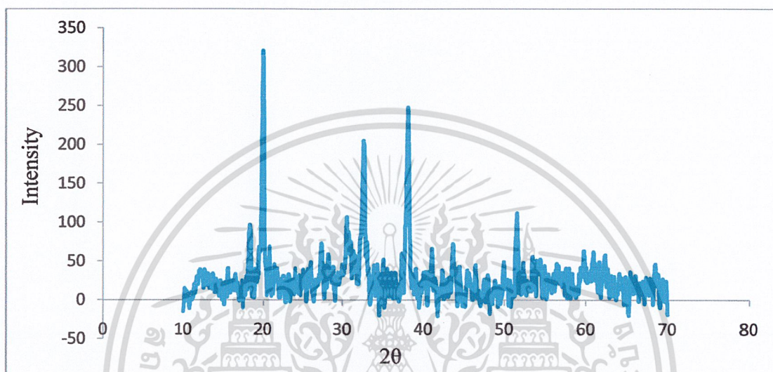
รูปที่ ก.1 กราฟจากเครื่องเอ็กซ์เรย์ดิฟแฟรคโทมิเตอร์ของโคบอลต์ไฮดรอกไซด์ ( \text{Co(OH)}_2 )
