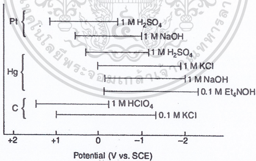
รูปที่ 2.10 แสดงช่วงศักย์ไฟฟ้าที่สามารถให้แก่ขั้วไฟฟ้าแพลทินัม คาร์บอนและเมอร์คิวรี ในอิเล็กโทรไลต์เกี่ยวหนุชนิดต่างๆ
