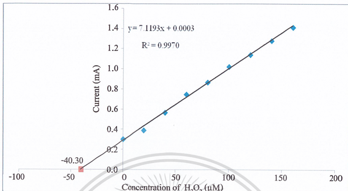
รูปที่ 4.21 กราฟแสดงความสัมพันธ์ระหว่างความเข้มข้นของไฮโดรเจนเปอร์ออกไซด์กับกระแสไฟฟ้าในสารละลายฟอสเฟตบัฟเฟอร์ พีเอช 7 ความเข้มข้น 0.10 โมลาร์ ของสารละลายตัวอย่างตัวอย่าง น้ำยาล้างแผลตามร่างกายตามรายนามกฎพยานาคู
