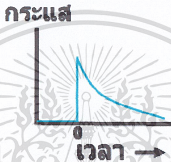
รูปที่ 2.16 กราฟที่ได้จากการวิเคราะห์ โดยเทคนิคแอมเพอโรเมทรี
