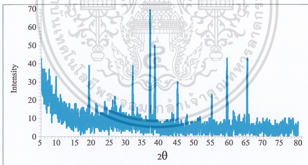
รูปที่ 4.6 กราฟจากเครื่องเอกซเรย์ดิฟแฟรคโทมิเตอร์ของขั้วไฟฟ้าทินออกไซด์เจือฟลูออรีนที่ปรับปรุงด้วยโคบอลต์ออกไซด์
