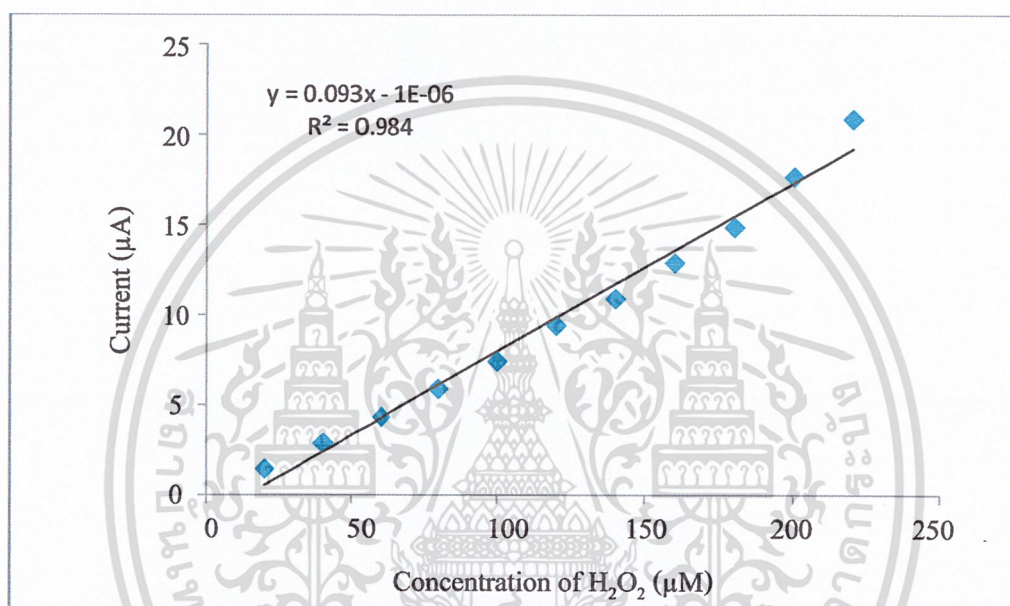
รูปที่ ฉ.2 แสดงกราฟจากการพลอตระหว่างกระแสกับความเข้มข้น ไฮโดรเจนเปอร์ออกไซด์ในสารละลายโพสเฟตบัฟเฟอร์ พีเอช 7 ความเข้มข้น 0.10 โมลาร์
