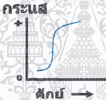
รูปที่ 2.14 กราฟแสดงความสัมพันธ์ระหว่างกระแสกับศักย์ไฟฟ้า โดยการทำแทสต์โพลาโรกราฟี
