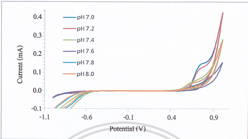
รูปที่ 4.10 ไซคลิกโวลแทมโมแกรมของการตรวจวัดสารละลายไฮโดรเจนเปอร์ออกไซด์ 1.00 มิลลิโมลลาร์ ในสารละลายฟอสเฟตบัฟเฟอร์พีเอช 7.0, 7.2, 7.4, 7.6, 7.8 และ 8.0 ด้วยขั้วไฟฟ้าทินออกไซด์เจือฟลูออรีนที่ปรับปรุงด้วยโกลบอลด์ออกไซด์ สแกนศักย์ไฟฟ้าในช่วง -1.0 ถึง +1.0 โวลต์ (เทียบกับขั้วอ้างอิงซิลเวอร์/ซิลเวอร์คลอไรด์) อัตราการสแกน 50 มิลลิโวลต์ต่อวินาที
