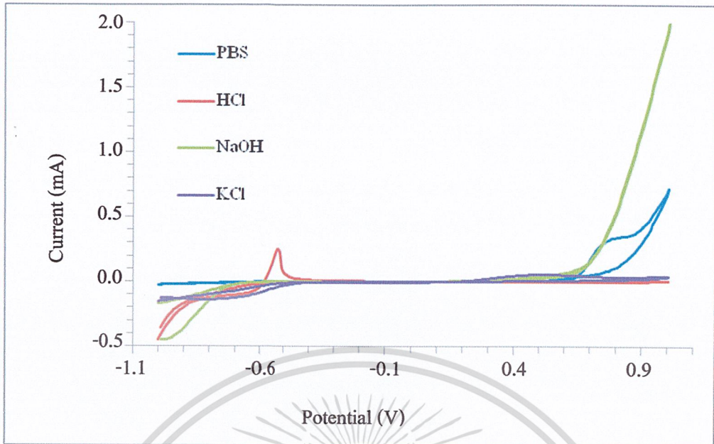
รูปที่ 4.8 ไชคลิกโวลแทมโมแกรมของการตรวจวัดไฮโดรเจนเปอร์ออกไซด์ความเข้มข้น 1.00 มิลลิโมลาร์ ในสารละลายอิเล็กโทรไลต์ชนิดต่างๆ ได้แก่
