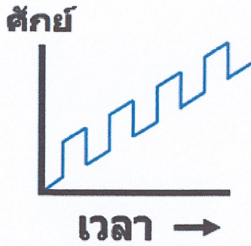
รูปที่ 2.19 กราฟแสดงความสัมพันธ์ระหว่างศักย์ไฟฟ้ากับเวลาของพัลส์โวลแทจเมทรีแบบคิฟเฟอร์เรนเซียสพัลส์
