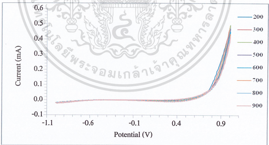
รูปที่ 4.13 ไชคติกโวลแทมโมแกรมของการตรวจวัดไฮโดรเจนเปอร์ออกไซด์ความเข้มข้น 1.00 มิลลิโมลลาร์ ในสารละลายบัฟเฟอร์ฟอสเฟตพีเอช 7 ความเข้มข้น 0.10 โมลาร์ ด้วยขั้วไฟฟ้าทินออกไซด์เจือฟลูออรีนที่ปรับปรุงด้วยโพลีเมอร์ออกไซด์ สแกนศักย์ไฟฟ้า
