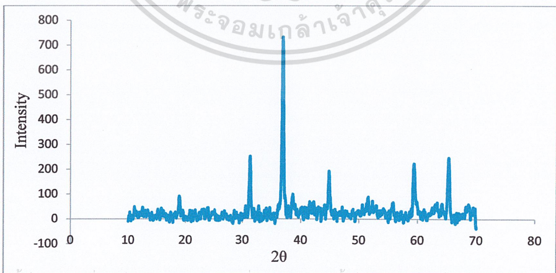
เอกสารนี้เป็นเอกสารที่สงวนไว้สำหรับการใช้งานเพื่อการศึกษาเท่านั้น เมื่อนุญาตให้นำไปใช้ประโยชน์ด้านการค้า รูปที่ ก.2 กราฟจากเครื่องเอ็กซ์เรย์ดิฟแฟรคโทมิเตอร์ของโคบอลต์ออกไซด์ ( \text{Co}_3\text{O}_4 ) ครั้งที่มีการนำไปใช้
