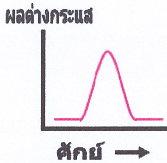
รูปที่ 2.22 กราฟแสดง โวลแทมโมแกรมของพัลส์ โวลแทมเมทรีสแควร์ – เวฟ
