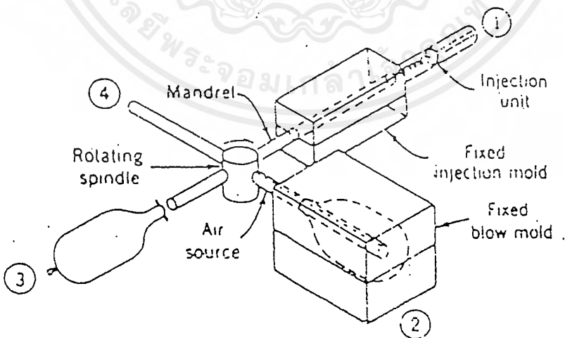
ภาพการทำงานแบบฉีดชนิด Injection Blow Molding
