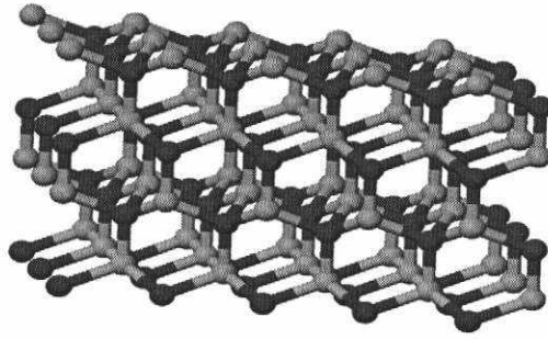
รูปที่ 2.9 โครงสร้างของซิงค์ออกไซด์
