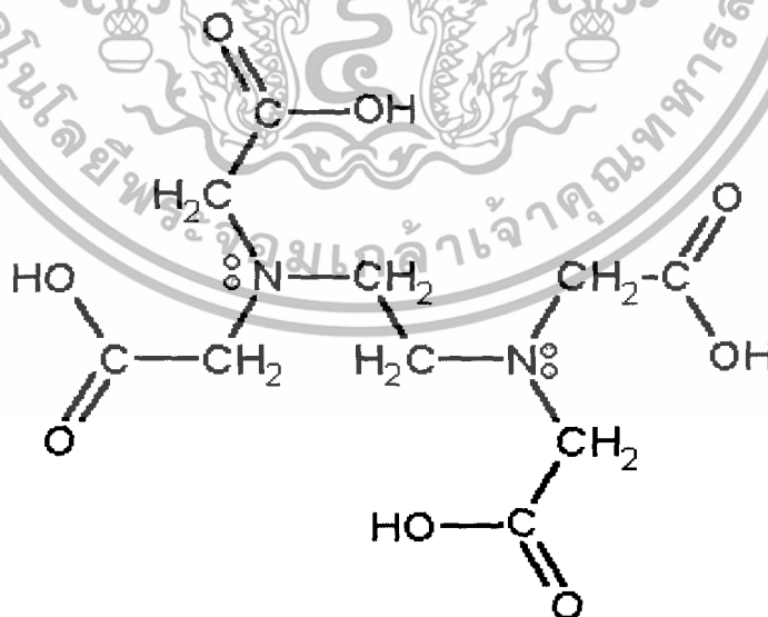
รูปที่ 2.12 สูตร โครงสร้างของอีดีทีเอ
