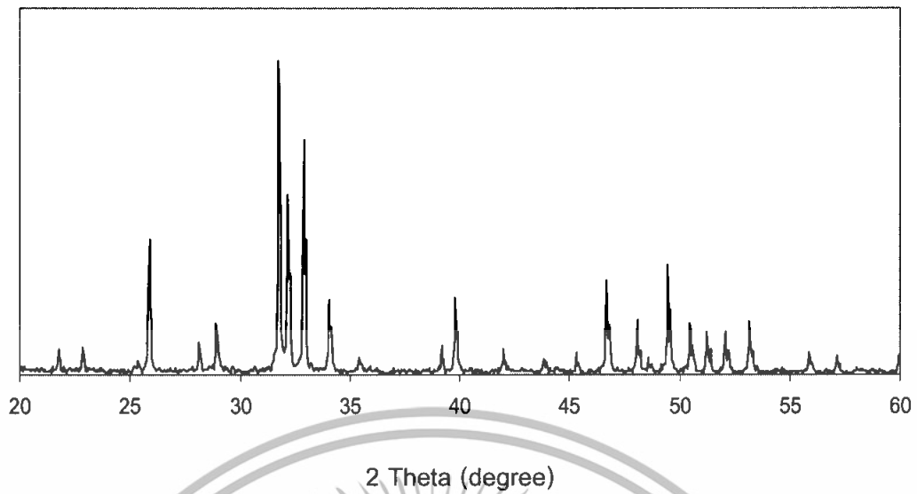
รูปที่ ง-1 รูปแบบการเลี้ยวเบนรังสีเอ็กซ์ของไฮดรอกซีแอปาทิตที่ผ่านการเผาที่อุณหภูมิ
