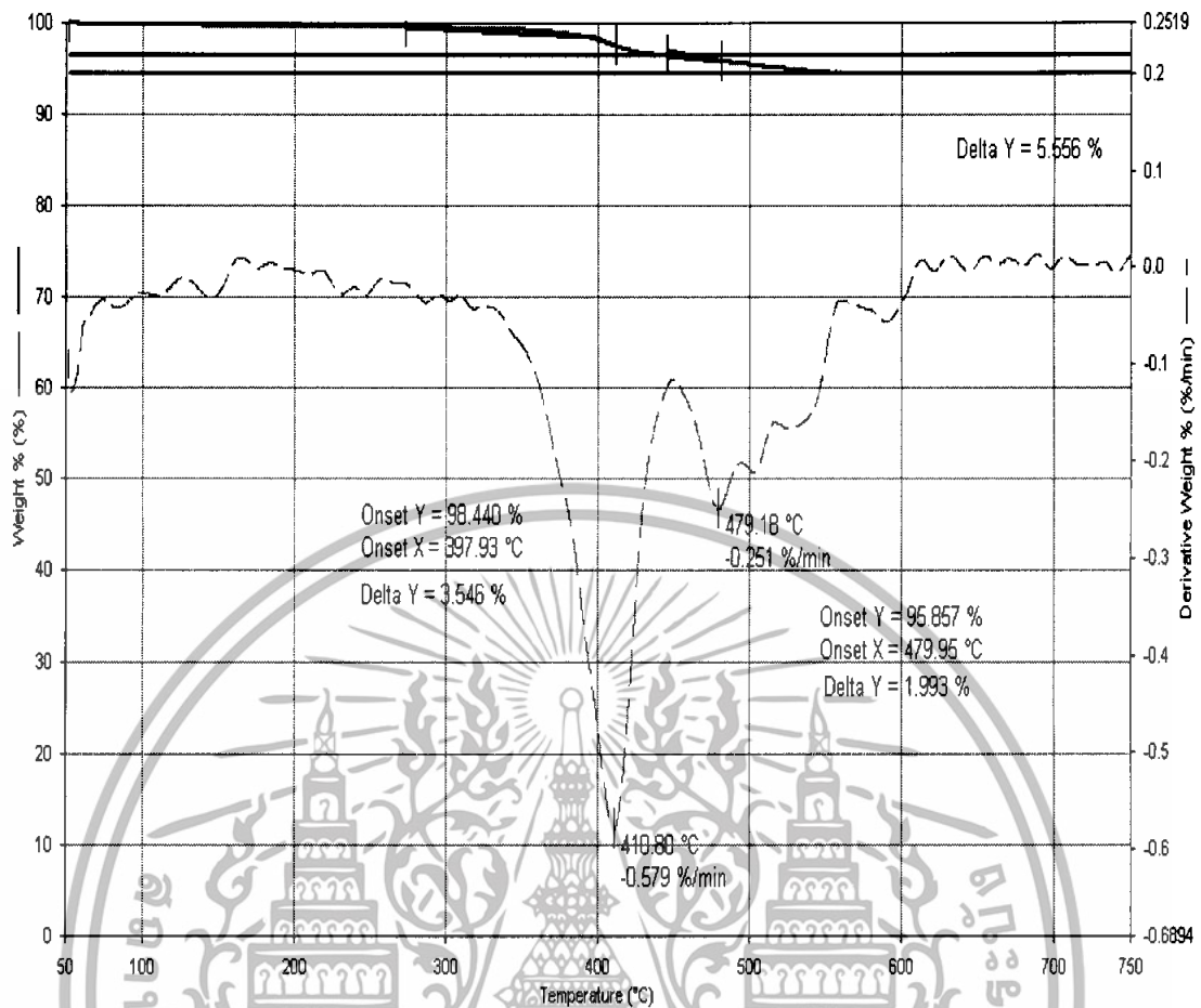
รูปที่ ๓-2 เทอร์โมแกรมจากเครื่อง TGA ของวัสดุประกอบ HAP/PET
