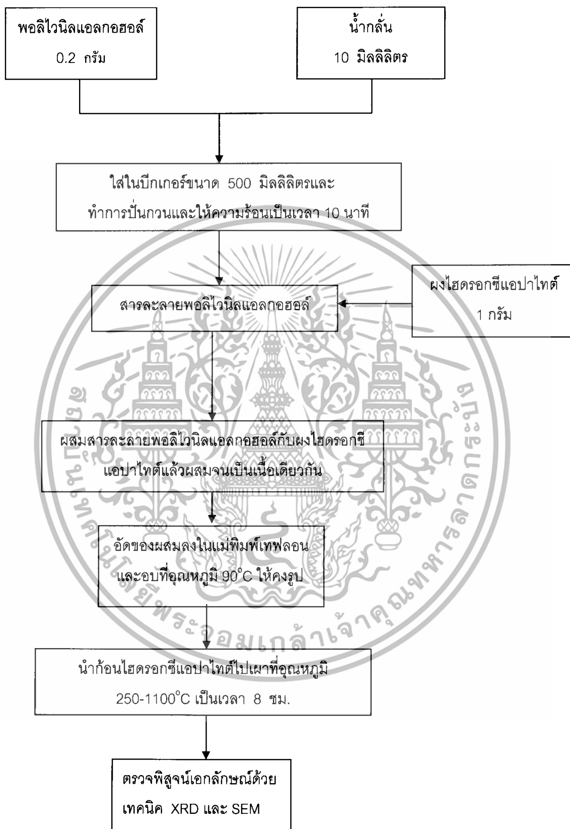
รูปที่ 3.3 แผนงานการขึ้นรูปไฮดรอกซีเอปาทาไทต์
