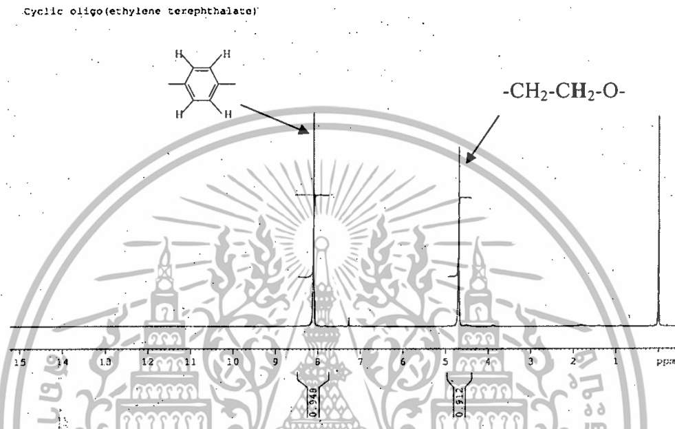
รูปที่ 4.4 สเปกตรัม ^1\text{H-NMR} ของ C-OET ที่สังเคราะห์ได้จากปฏิกิริยาพอลิเมอไรเซชันแบบควบแน่น
