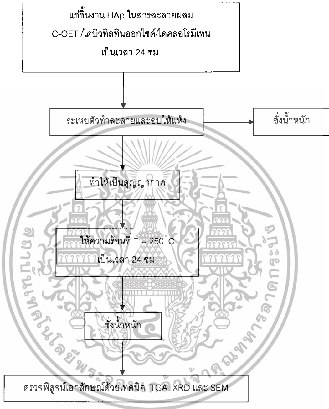
รูปที่ 3.5 แผนงานการเตรียมวัสดุประกอบ HAp/PET
