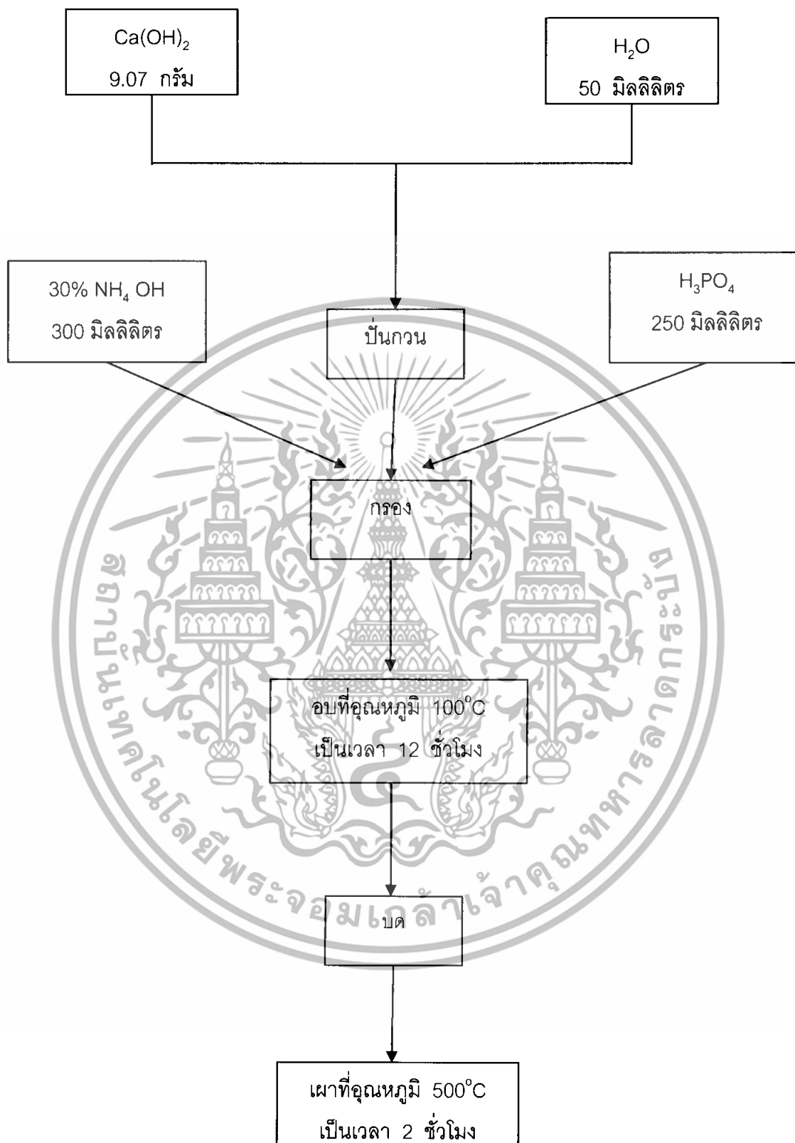
รูปที่ 3.2 แผนงานการสังเคราะห์ไฮดรอกซีแอปาทาइट
