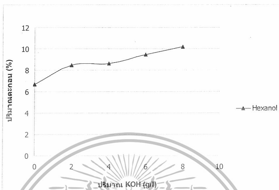
รูปที่ 4.12 ผลของปริมาณโพแทสเซียมไฮดรอกไซด์ที่มีต่อปริมาณตะกอนที่แยกจากน้ำมันหล่อลื่นใช้แล้วเมื่อใช้ตัวทำละลายเฮกซานอล
