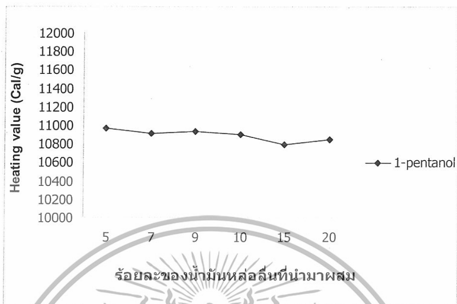
รูปที่ 4.24 ค่าความร้อนของน้ำมันผสมที่ได้จากการสกัดด้วยเพนทานอล
