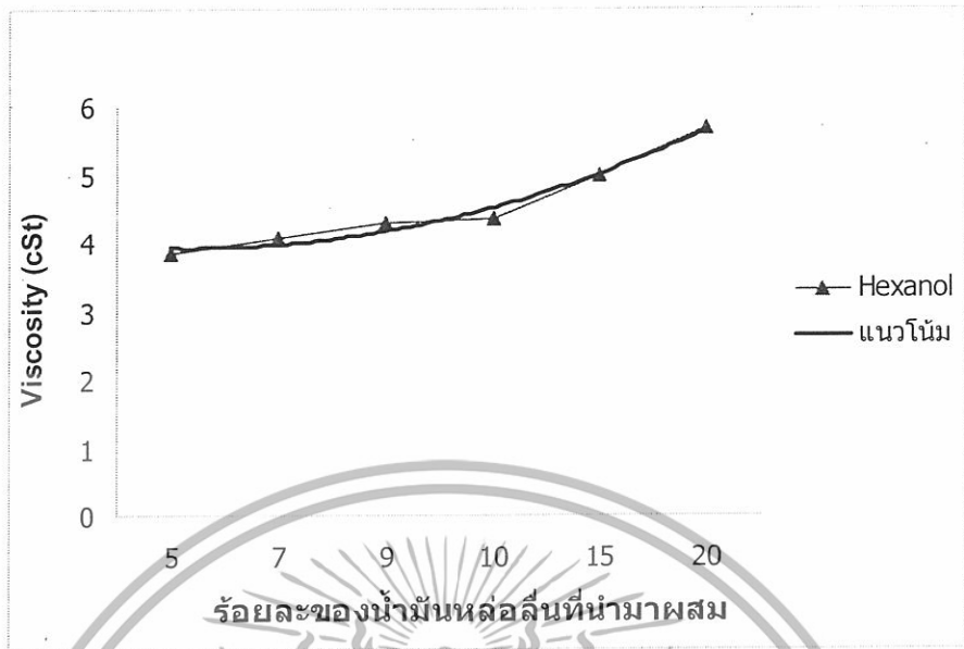
รูปที่ 4.19 แวนโธล์ค่าความหนืดของน้ำมันผสมที่ได้จากการสกัดด้วยเฮกซานอล
