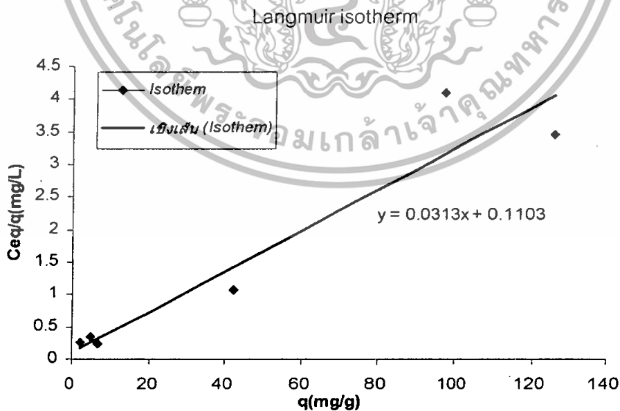
ภาพที่ 12 แสดงสมการเส้นตรงจากผลของการดูดซับแคดเมียมที่ระดับ 20, 40, 80, 160 และ 200 ppm
