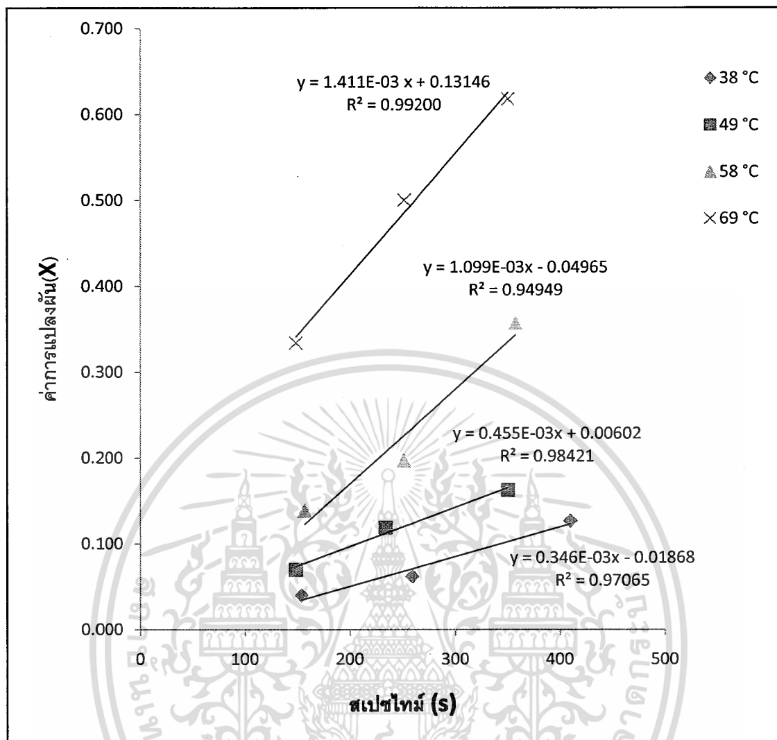
รูปที่ 4.2 กราฟปฏิกิริยาอันดับศูนย์ ที่ความเข้มข้นซูโครสเริ่มต้นเท่ากับ 34.47 กรัมต่อ 100 มิลลิลิตร
