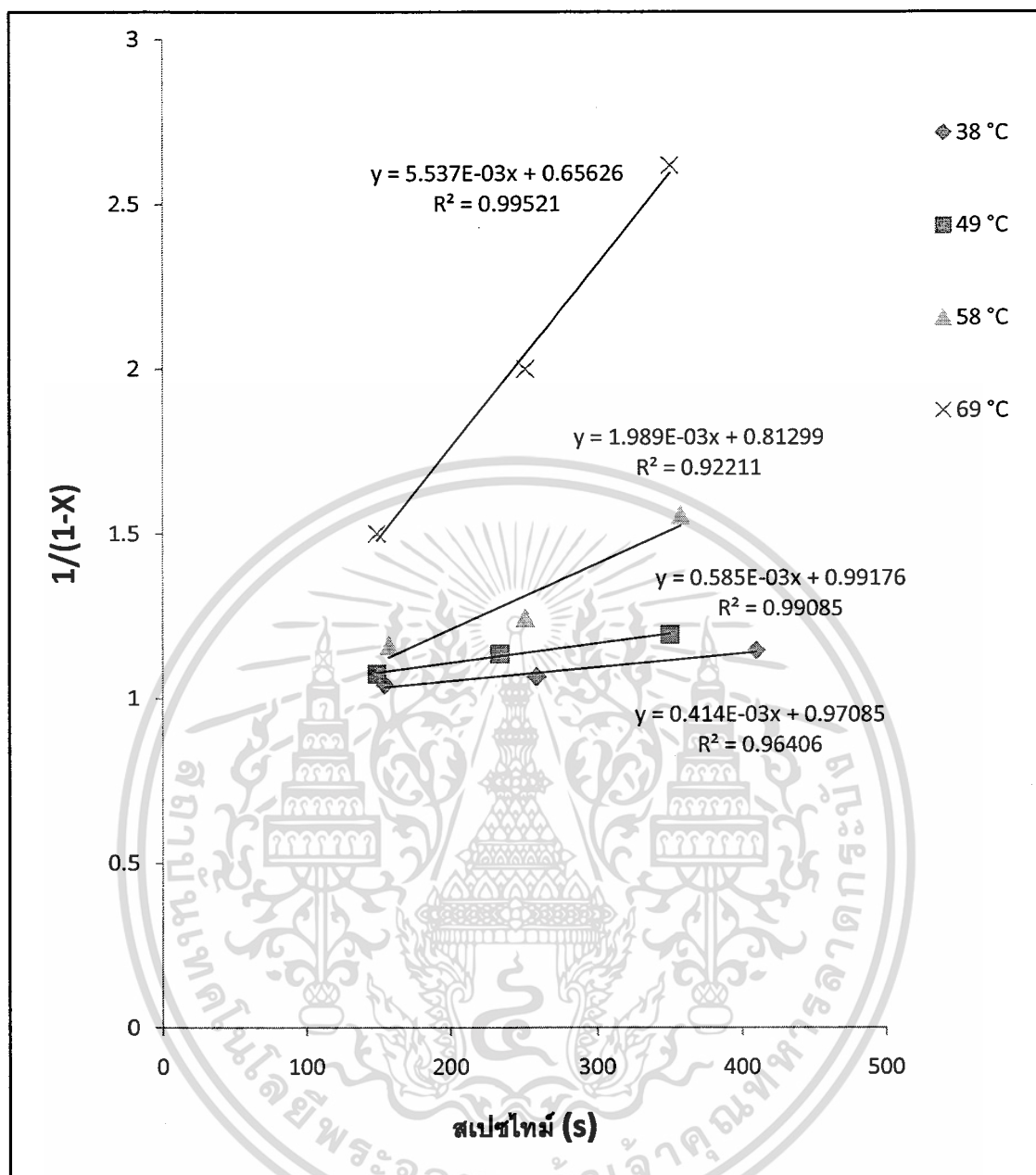
รูปที่ 4.6 กราฟปฏิกิริยาอันดับสอง ที่ความเข้มข้นซูโครสเริ่มต้นเท่ากับ 34.47 กรัมต่อ 100 มิลลิลิตร
