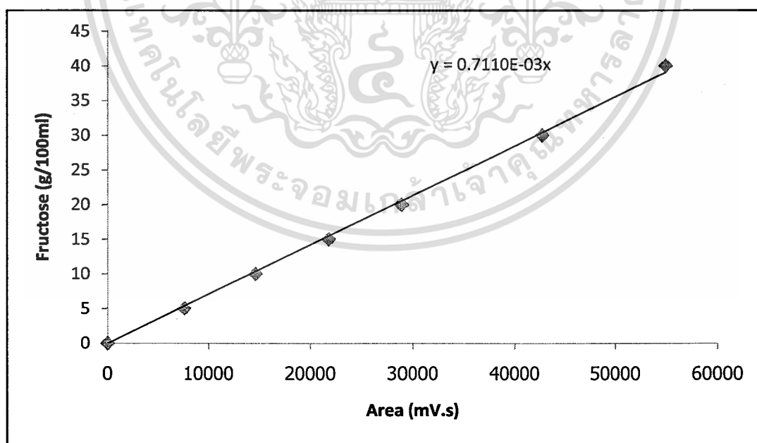
รูปที่ ข3. กราฟวิเคราะห์ปริมาณฟรุคโตส
