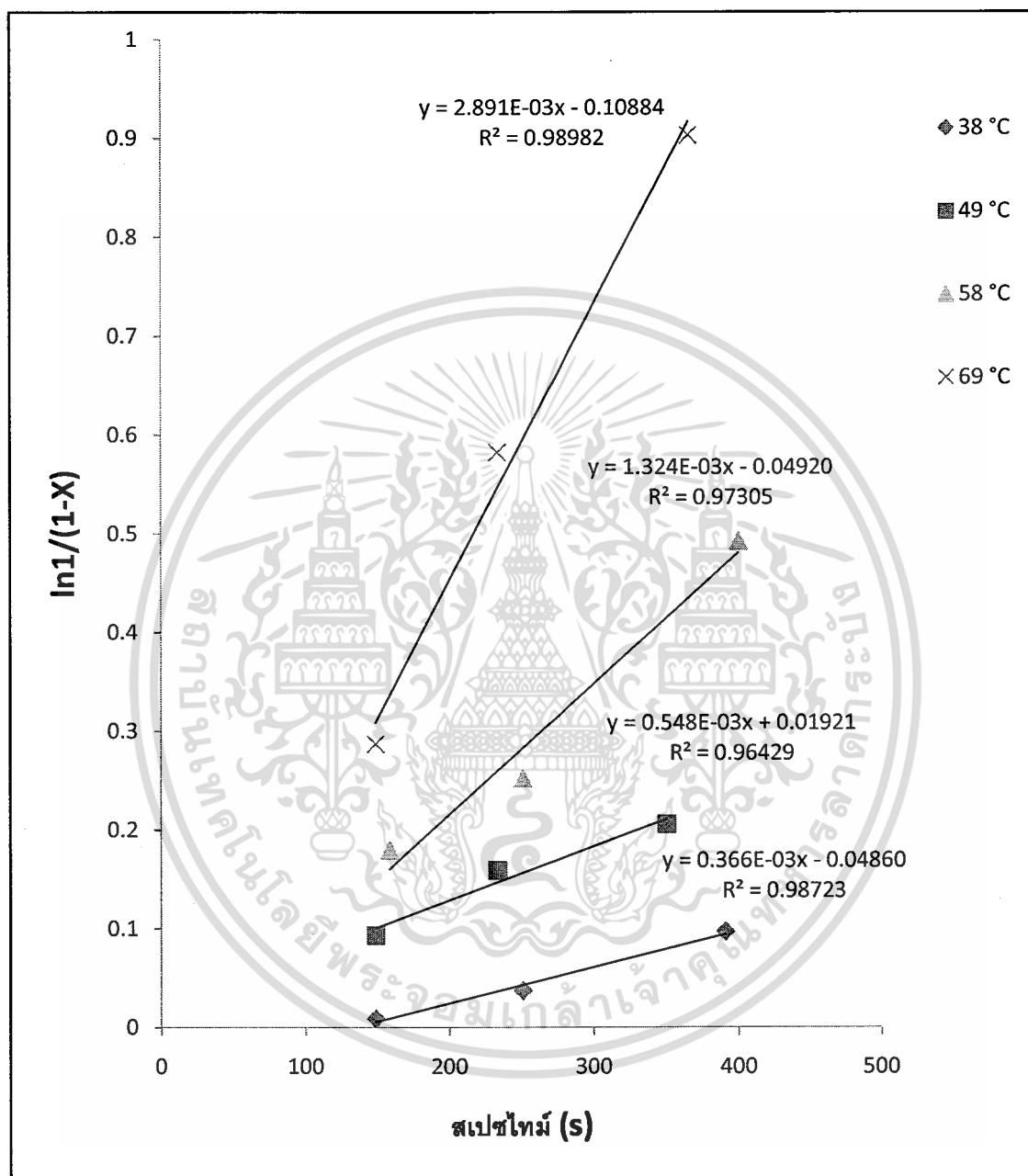
รูปที่ 4.3 กราฟปฏิกิริยาอันดับหนึ่ง ที่ความเข้มข้นซูโครสเริ่มต้นเท่ากับ 16.98 กรัมต่อ 100 มิลลิลิตร
