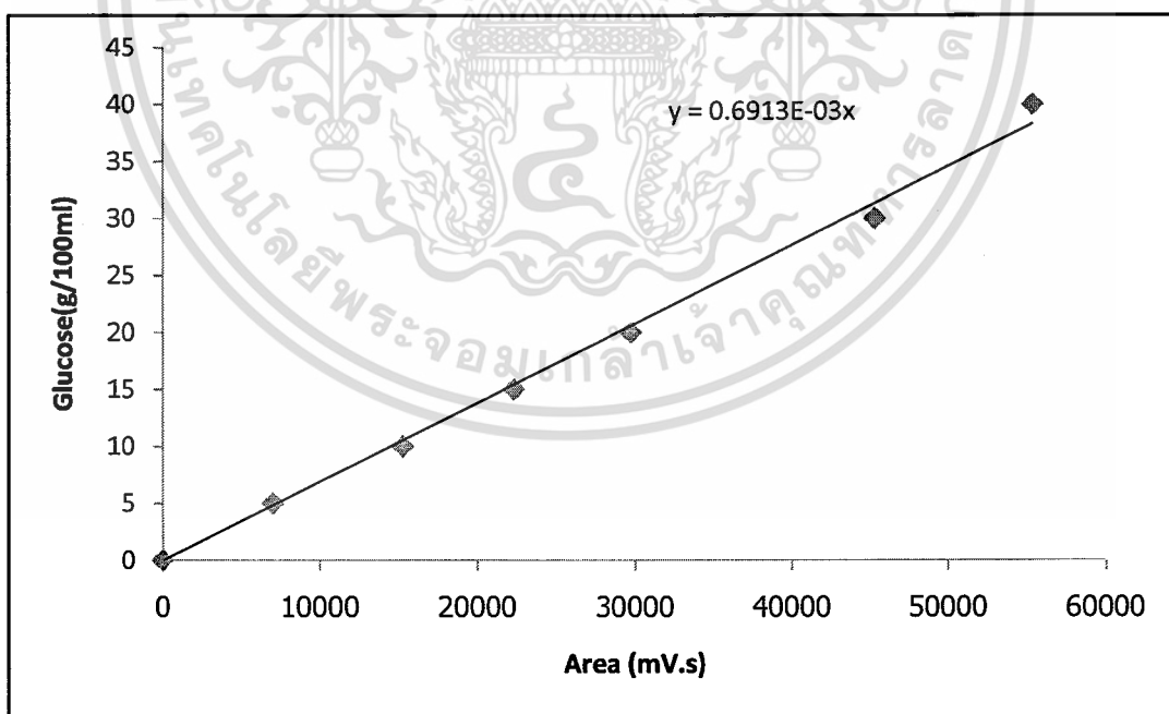
รูปที่ ข2. กราฟวิเคราะห์ปริมาณกลูโคส
