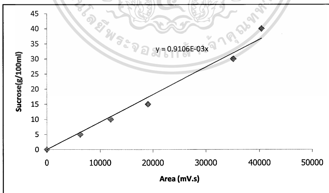
รูปที่ ข1. กราฟวิเคราะห์ปริมาณซูโครส
