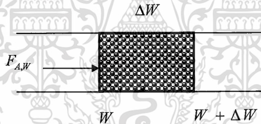
รูปที่ 2.5 เครื่องปฏิกรณ์แบบเบดบรรจุ
