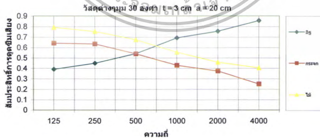
รูปที่ 5.202 สัมประสิทธิ์การดูดซึมเสียงของวัสดุต่างๆ \theta = 30^\circ ที่ t = 3 \text{ cm} a = 20 \text{ cm}
