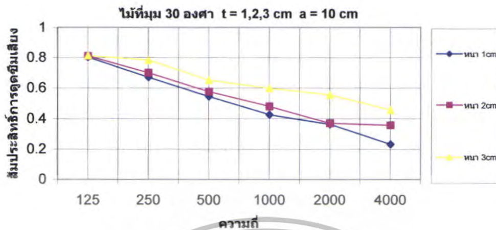
รูปที่ 5.107 สัมประสิทธิ์การดูดซับเสียงของไม้ที่ \theta = 30^\circ t = 1,2,3 \text{ cm} a = 10 \text{ cm}
