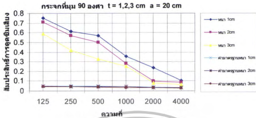
รูปที่ 5.65 สัมประสิทธิ์การดูดซับเสียงของกระจกที่ \theta = 90^\circ t = 1,2,3 \text{ cm} a = 20 \text{ cm}
