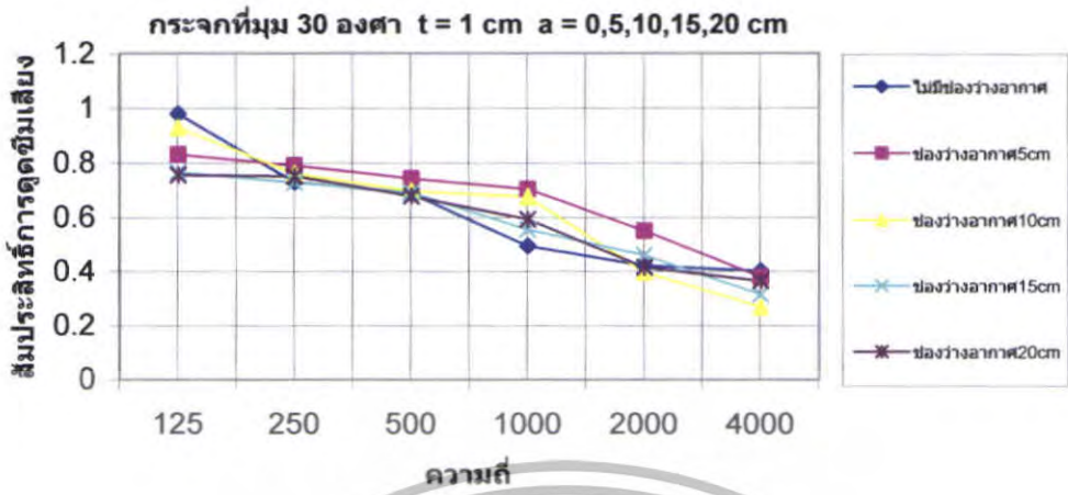
รูปที่ 5.78 สัมประสิทธิ์การดูดซับเสียงของกระจกที่ \theta = 30^\circ t = 1 \text{ cm} a = 5,10,15,20 \text{ cm}
