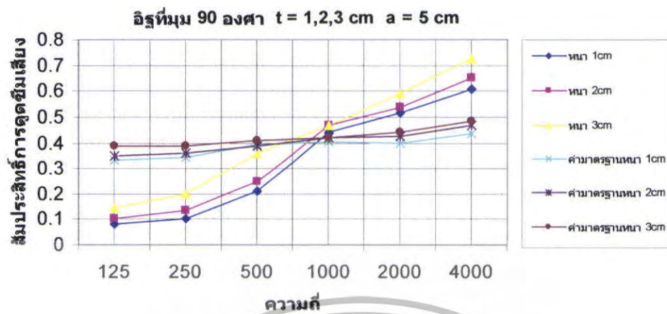
รูปที่ 5.6 สัมประสิทธิ์การดัดขี้มเสถียงของอิฐที่ \theta = 90^\circ t = 1,2,3 \text{ cm} a = 5 \text{ cm}
