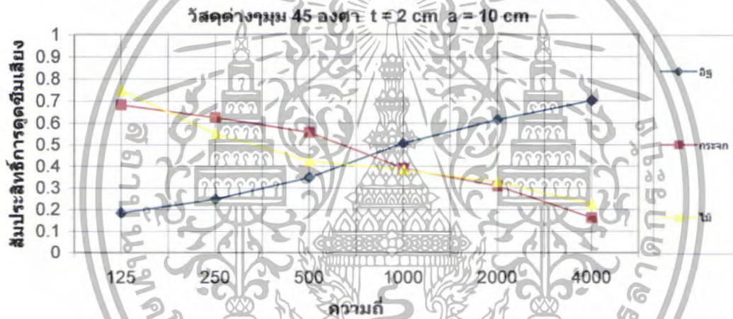
รูปที่ 5.174 สัมประสิทธิ์การดัดขีมิเปลี่ยนของวัสดุต่างๆ \theta = 45^\circ ที่ t = 2 \text{ cm} a = 10 \text{ cm}
