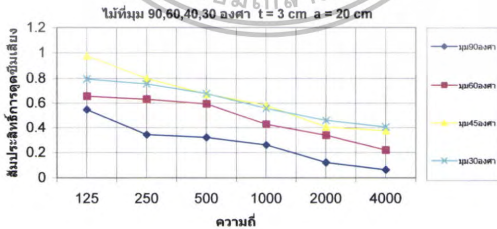
รูปที่ 5.142 สัมประสิทธิ์การดูดซับเสียงของไม้ \theta = 90^\circ, 60^\circ, 45^\circ, 30^\circ ที่ t = 3 \text{ cm} a = 20 \text{ cm}
