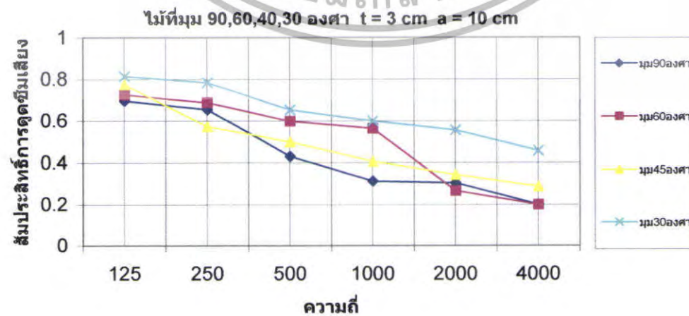
รูปที่ 5.136 สัมประสิทธิ์การหดขี้นเสียงของไม้ \theta = 90^\circ, 60^\circ, 45^\circ, 30^\circ ที่ t = 3 cm a = 10 cm
