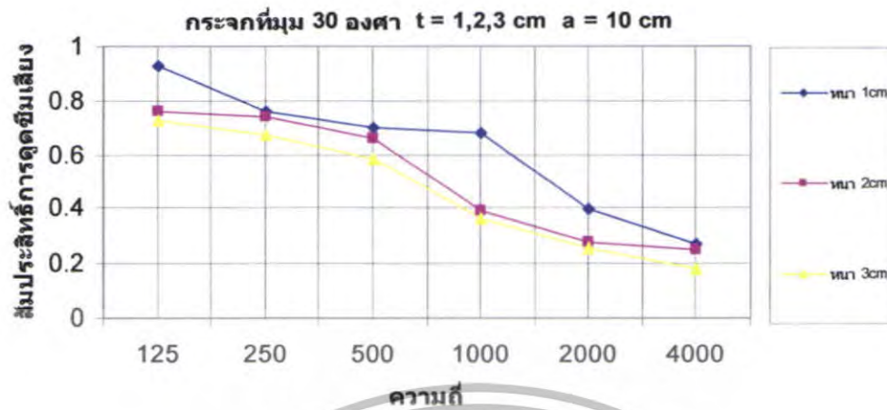
รูปที่ 5.60 สัมประสิทธิ์การดูดซับเสียงของกระฉากที่ \theta = 30^\circ t = 1,2,3 \text{ cm} a = 10 \text{ cm}
