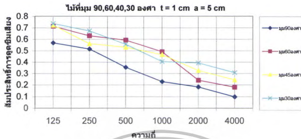
รูปที่ 5.131 สัมประสิทธิ์การดูดซึมเสียงของไม้ \theta = 90^\circ, 60^\circ, 45^\circ, 30^\circ ที่ t = 1 \text{ cm} a = 5 \text{ cm}
