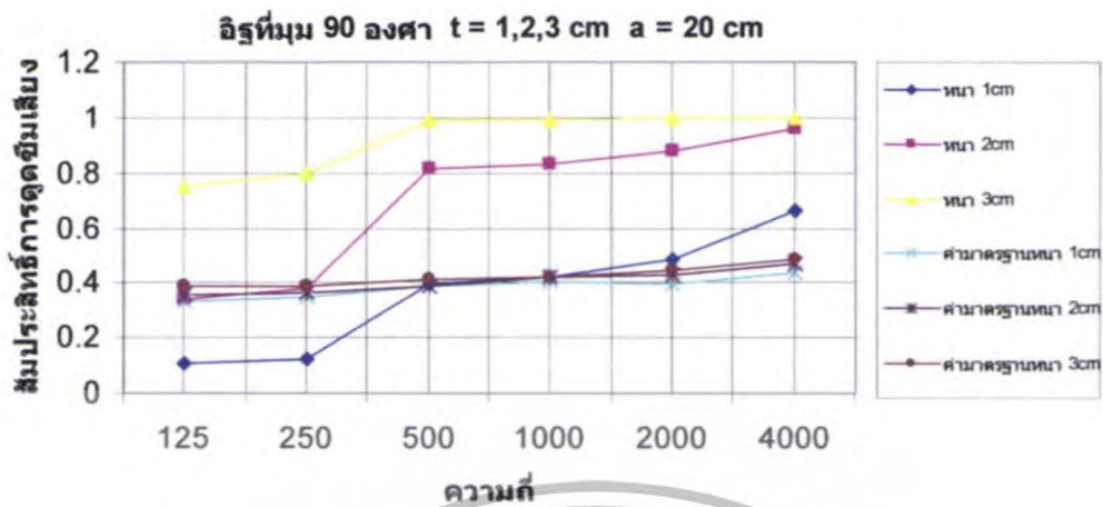
รูปที่ 5.18 สัมประสิทธิ์การดูดซึมเสื่อมของอิฐที่ \theta = 90^\circ t = 1,2,3 \text{ cm} a = 20 \text{ cm}
