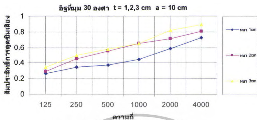
รูปที่ 5.13 สัมประสิทธิ์การดูดซับเสียงของอิฐที่ \theta = 30^\circ t = 1,2,3 cm a = 10 cm
