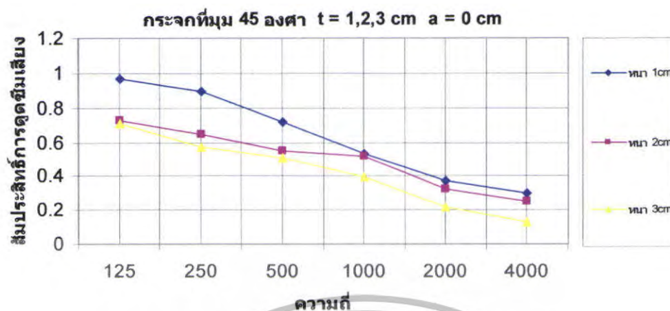
รูปที่ 5.51 สัมประสิทธิ์การดูดซับเสียงของกระจกที่ \theta = 45^\circ t = 1,2,3 \text{ cm} a = 0 \text{ cm}
