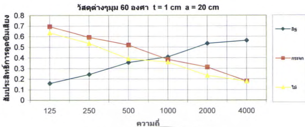
รูปที่ 5.194 สัมประสิทธิ์การดูดซับเสียงของวัสดุต่างๆ \theta = 60^\circ ที่ t = 1 \text{ cm} a = 20 \text{ cm}
