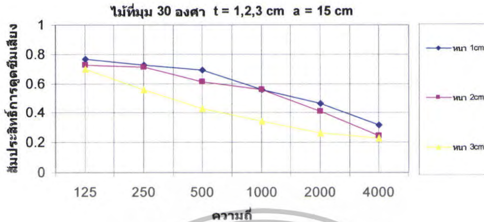
รูปที่ 5.64 สัมประสิทธิ์การดัดขึ้นเสียดังของกระจกที่ \theta = 30^\circ t = 1,2,3 \text{ cm} a = 15 \text{ cm}
