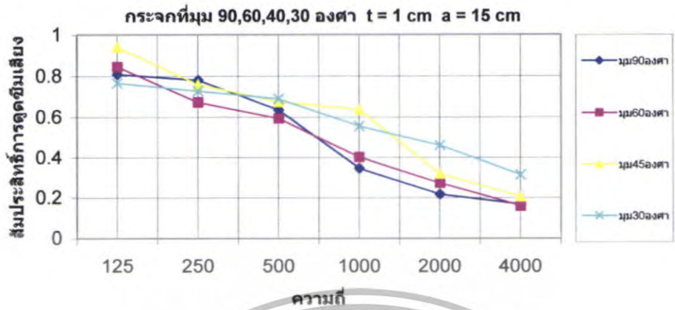
รูปที่ 5.90 สัมประสิทธิ์การดูดซึมเสียงของกระบอก \theta = 90^\circ, 60^\circ, 45^\circ, 30^\circ ที่ t = 1 \text{ cm} a = 15 \text{ cm}
