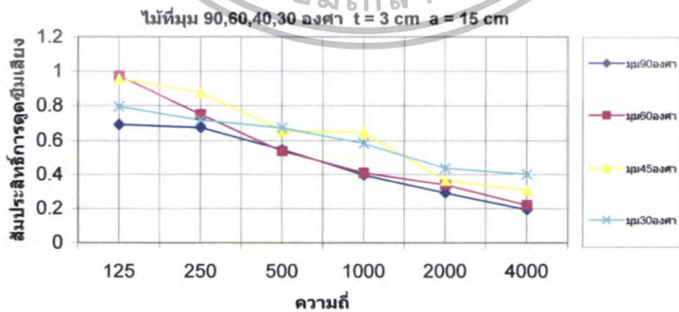
รูปที่ 5.139 สัมประสิทธิ์การหดขีมีเปลี่ยนแปลงของไม้ \theta = 90^{\circ}, 60^{\circ}, 45^{\circ}, 30^{\circ} ที่ t = 3 cm a = 15 cm
