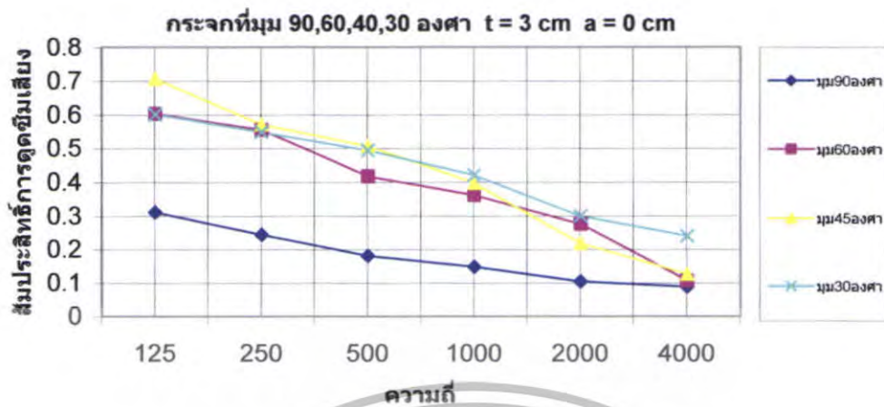
รูปที่ 5.83 สัมประสิทธิ์การดูดซึมเสียงของกระจก \theta = 90^\circ, 60^\circ, 45^\circ, 30^\circ ที่ t = 3 \text{ cm} a = 0 \text{ cm}
