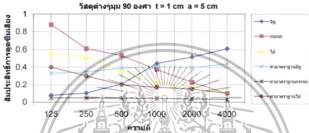
รูปที่ 5.155 สัมประสิทธิ์การดูดซึมเสียงของวัสดุต่างๆ \theta = 90^\circ ที่ t = 1 cm a = 5 cm
