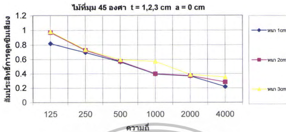
รูปที่ 5.98 สัมประสิทธิ์การดูดซับเสียงของไม้ที่ \theta = 45^\circ t = 1,2,3 \text{ cm} a = 0 \text{ cm}
