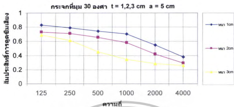
รูปที่ 5.56 สัมประสิทธิ์การดูดซึมเสียงของกระจกที่ \theta = 30^\circ t = 1,2,3 \text{ cm} a = 5 \text{ cm}
