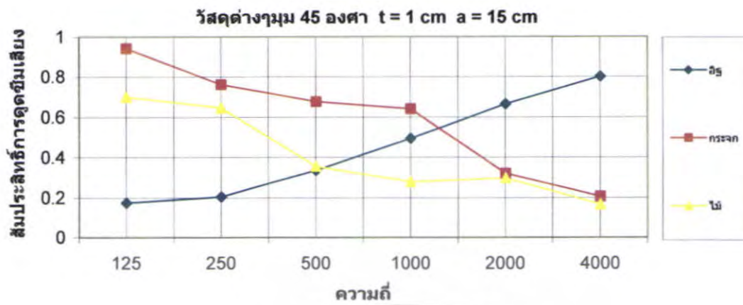
รูปที่ 5.185 สัมประสิทธิ์การดัดขี้นเฉียงของวัสดุต่างๆ \theta = 45^\circ ที่ t = 1 \text{ cm} a = 15 \text{ cm}
