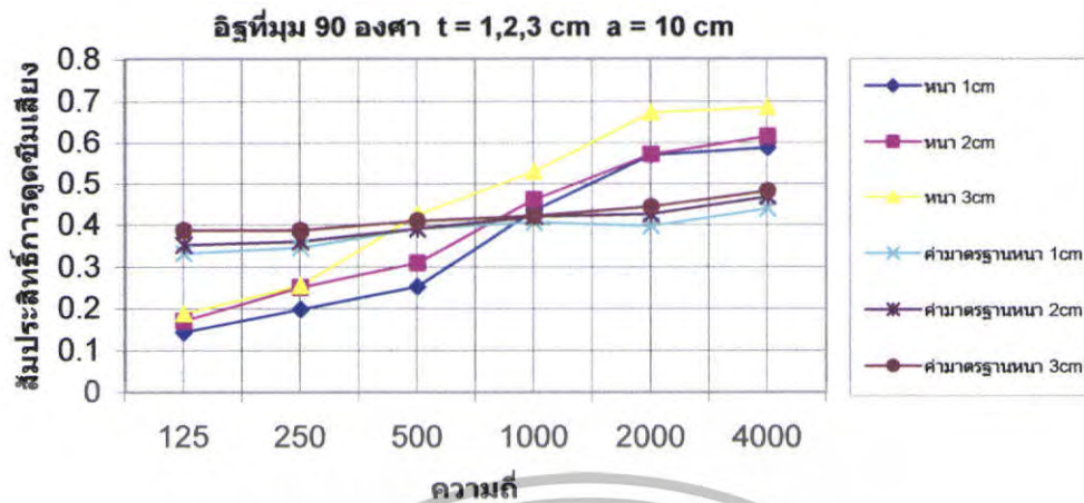
รูปที่ 5.10 สัมประสิทธิ์การดูดซึ่มเสียงของอิฐที่ \theta = 90^\circ t = 1,2,3 \text{ cm} a = 10 \text{ cm}
