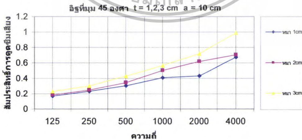
รูปที่ 5.12 สัมประสิทธิ์การดูดซึ่มเสียงของอิฐที่ \theta = 45^\circ t = 1,2,3 \text{ cm} a = 10 \text{ cm}
