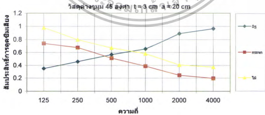
รูปที่ 5.199 สัมประสิทธิ์การดัดขี้นเสียงของวัสดุต่างๆ \theta = 45^\circ ที่ t = 3 \text{ cm} a = 20 \text{ cm}
