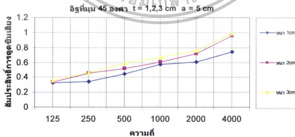
รูปที่ 5.8 สัมประสิทธิ์การดัดขี้มเสถียงของอิฐที่ \theta = 45^\circ t = 1,2,3 \text{ cm} a = 5 \text{ cm}
