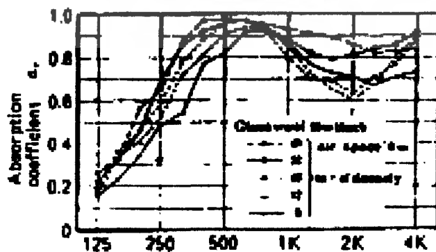
รูปที่ 3.16 สัมประสิทธิ์การดูดซับเสียงใยแก้ว ที่ความหนาแน่นต่าง ๆ
