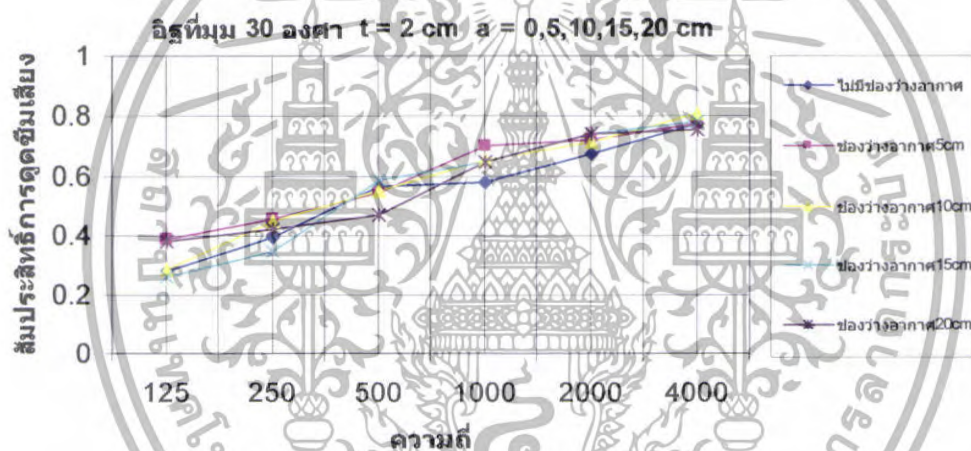
รูปที่ 5.32 สัมประสิทธิ์การดูดซับเสียงของอิฐที่ \theta = 30^\circ t = 2 \text{ cm} a = 5,10,15,20 \text{ cm}
