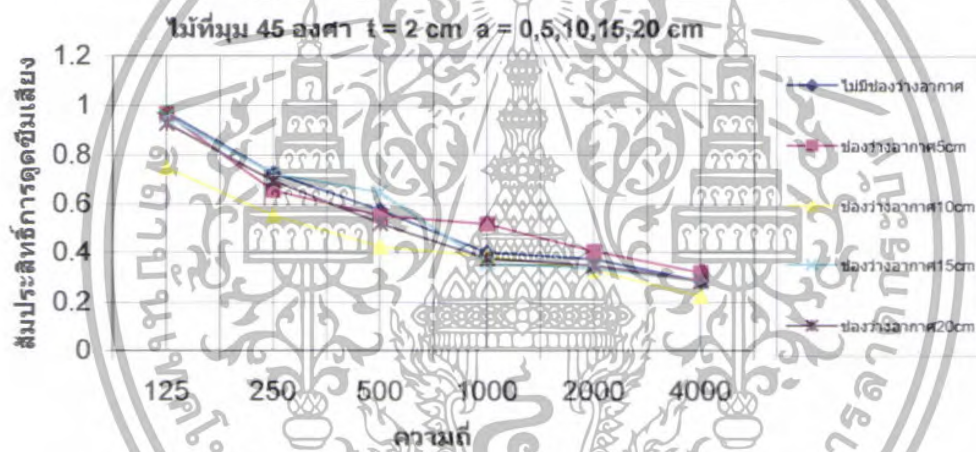
รูปที่ 5.123 สัมประสิทธิ์การดัดขี้นเสียงของไม้ที่ \theta = 45^\circ t = 2 cm a = 5,10,15,20 cm
