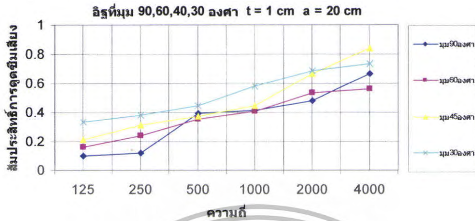
รูปที่ 5.46 สัมประสิทธิ์การดัดขีมิเสียงของอิฐ \theta = 90^{\circ}, 60^{\circ}, 45^{\circ}, 30^{\circ} ที่ t = 1 \text{ cm} a = 20 \text{ cm}
