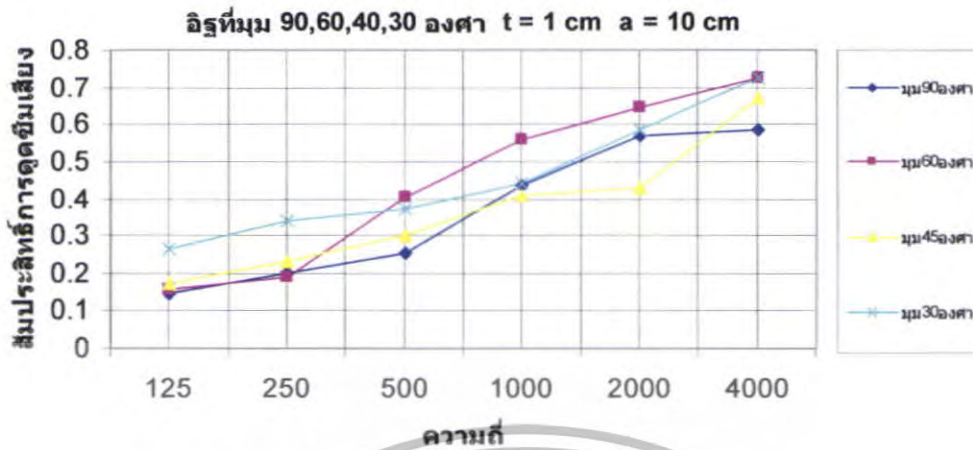
รูปที่ 5.40 สัมประสิทธิ์การดูดซึ่มเสียงของฉักร \theta = 90^\circ, 60^\circ, 45^\circ, 30^\circ ที่ t = 1 cm a = 10 cm
