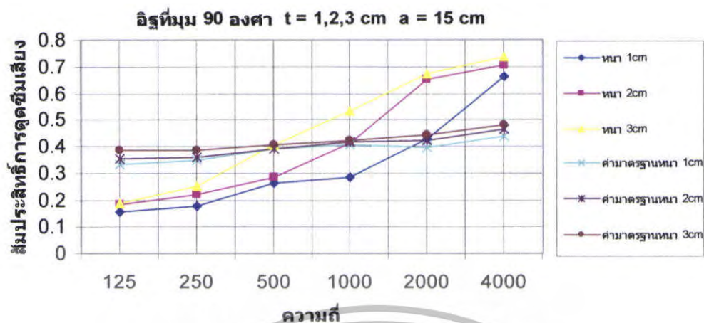
รูปที่ 5.14 สัมประสิทธิ์การดูดซึมน้ำของอิฐที่ \theta = 90^\circ t = 1,2,3 \text{ cm} a = 15 \text{ cm}
