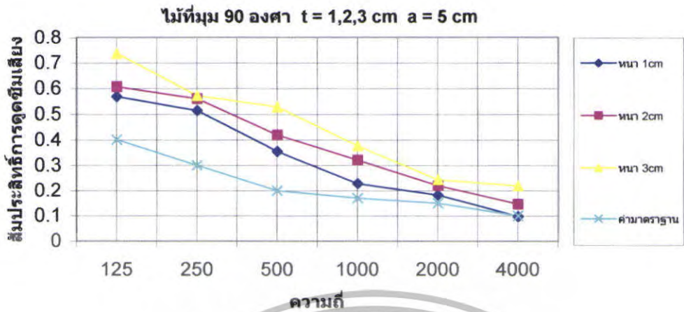
รูปที่ 5.100 สัมประสิทธิ์การดูดซับเชิงเสถียรของไม้ที่ \theta = 90^\circ t = 1,2,3 \text{ cm} a = 5 \text{ cm}
