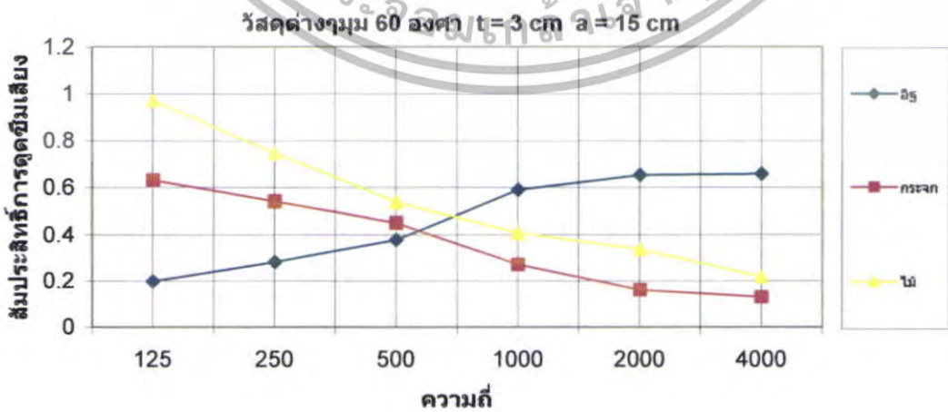
รูปที่ 5.184 สัมประสิทธิ์การดัดขี้นเคียงของวัสดุต่างๆ \theta = 60^\circ ที่ t = 3 \text{ cm} a = 15 \text{ cm}
