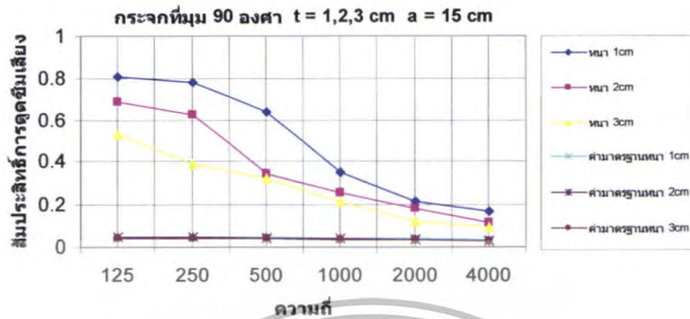
รูปที่ 5.61 สัมประสิทธิ์การดูดซับเสียงของกระบอกที่ \theta = 90^\circ t = 1,2,3 \text{ cm} a = 15 \text{ cm}
