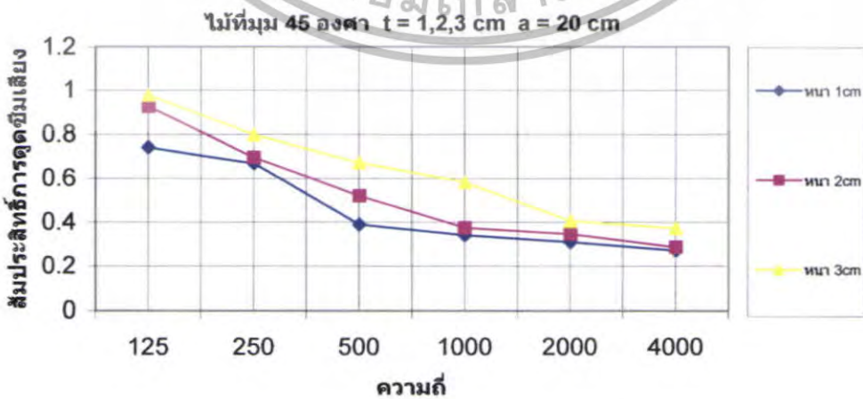
รูปที่ 5.114 สัมประสิทธิ์การดัดขี้นเคียงของไม้ที่ \theta = 45^\circ t = 1,2,3 \text{ cm} a = 20 \text{ cm}
