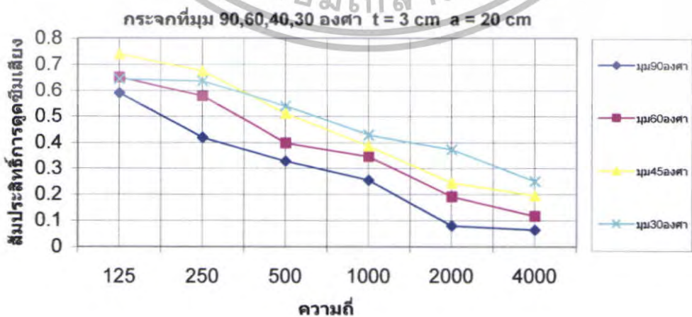
รูปที่ 5.95 สัมประสิทธิ์การดูดซับเสียงของกระจก \theta = 90^\circ, 60^\circ, 45^\circ, 30^\circ ที่ t = 3 \text{ cm} a = 20 \text{ cm} เอกสารนี้เป็นเอกสารที่สงวนไว้สำหรับการใช้งานเพื่อการศึกษาเท่านั้น ไม่อนุญาตให้นำไปใช้ประโยชน์ด้านการค้า ไม่ว่าจะกรณีใดๆทั้งสิ้น อีกทั้งห้ามมิให้ตัดแปลงเนื้อหา และต้องอ้างอิงถึงเจ้าของเอกสารทุกครั้งที่มีการนำไปใช้
