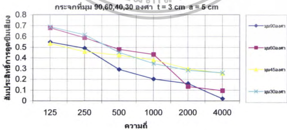
รูปที่ 5.86 สัมประสิทธิ์การดูดซับเสียงของกระบอก \theta = 90^{\circ}, 60^{\circ}, 45^{\circ}, 30^{\circ} ที่ t = 3 cm a = 5 cm
