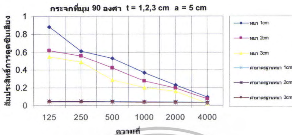
รูปที่ 5.53 สัมประสิทธิ์การดุดซึ่มเสียงของกระฉากที่ \theta = 90^\circ t = 1,2,3 \text{ cm} a = 5 \text{ cm}
