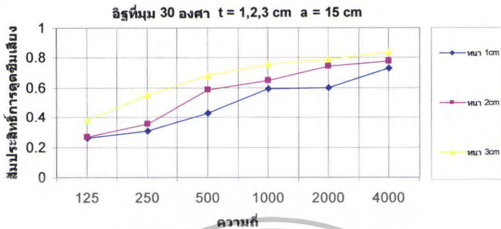
รูปที่ 5.17 สัมประสิทธิ์การดูดซับเสียงของอิฐที่ \theta = 30^\circ t = 1, 2, 3 cm a = 15 cm
