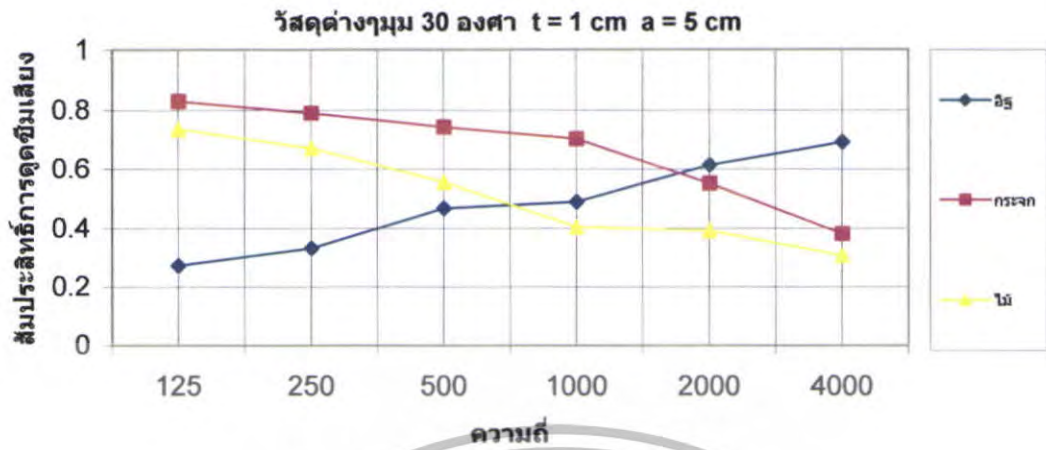
รูปที่ 5.164 สัมประสิทธิ์การดูดซับเสียงของวัสดุต่างๆ \theta = 30^\circ ที่ t = 1 \text{ cm} a = 5 \text{ cm}
