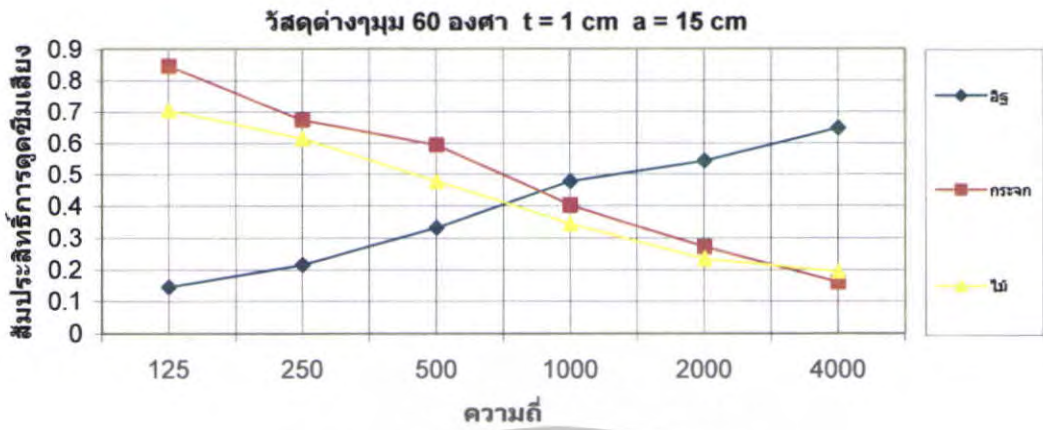
รูปที่ 5.182 สัมประสิทธิ์การดัดขี้นเคียงของวัสดุต่างๆ \theta = 60^\circ ที่ t = 1 \text{ cm} a = 15 \text{ cm}
