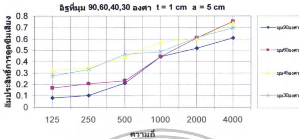
รูปที่ 5.37 สัมประสิทธิ์การดัดขี้นเสียงของอิฐ \theta = 90^\circ, 60^\circ, 45^\circ, 30^\circ ที่ t = 1 \text{ cm} a = 5 \text{ cm}
