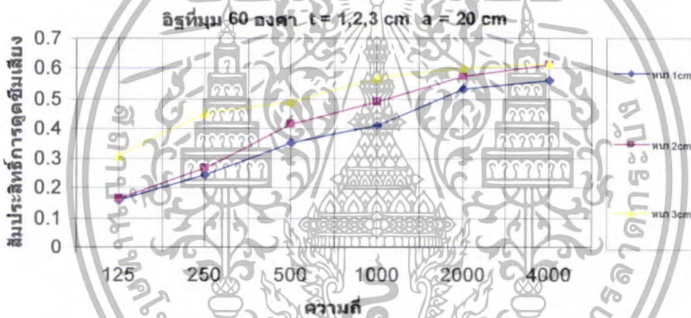
รูปที่ 5.19 สัมประสิทธิ์การดูดซึมเสื่อมของอิฐที่ \theta = 60^\circ t = 1,2,3 \text{ cm} a = 20 \text{ cm}
