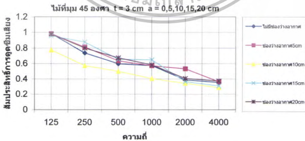
รูปที่ 5.124 สัมประสิทธิ์การดัดขี้นเสียงของไม้ที่ \theta = 45^\circ t = 3 cm a = 5,10,15,20 cm
