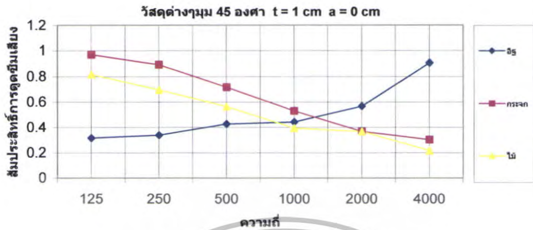
รูปที่ 5.149 สัมประสิทธิ์การดูดซึมเสียงของวัสดุต่างๆ \theta = 45^\circ ที่ t = 1 \text{ cm} a = 0 \text{ cm}
