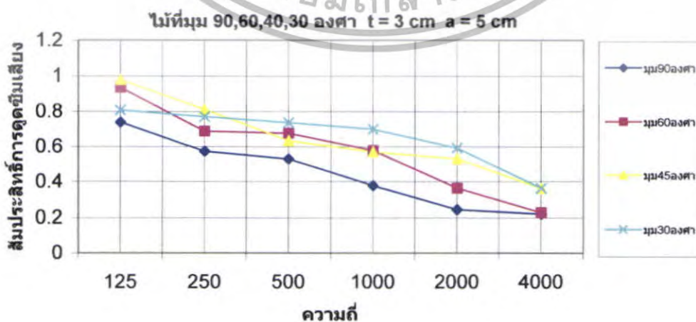
รูปที่ 5.133 สัมประสิทธิ์การดูดซึมเสียงของไม้ \theta = 90^\circ, 60^\circ, 45^\circ, 30^\circ ที่ t = 3 \text{ cm} a = 5 \text{ cm}
