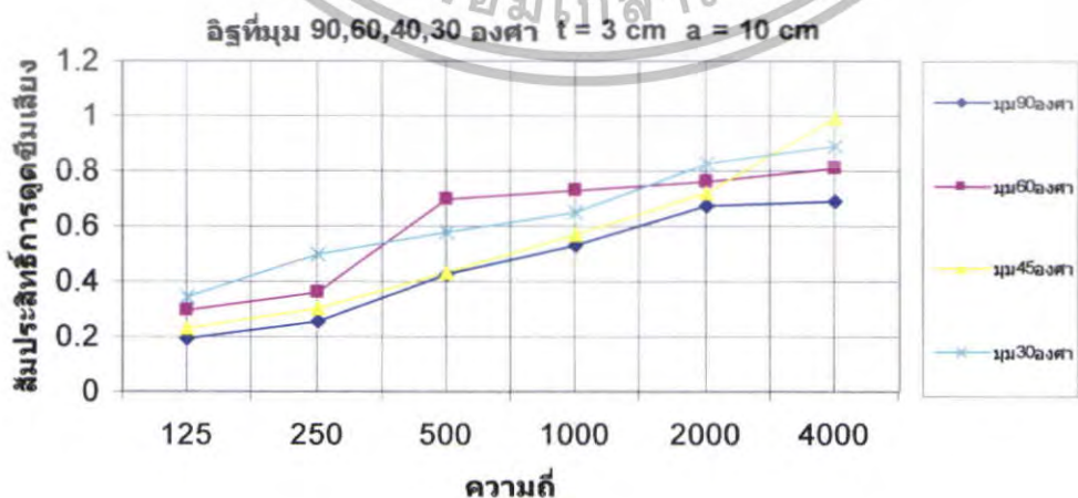
รูปที่ 5.42 สัมประสิทธิ์การดูดซึ่มเสียงของฉักร \theta = 90^\circ, 60^\circ, 45^\circ, 30^\circ ที่ t = 3 cm a = 10 cm
