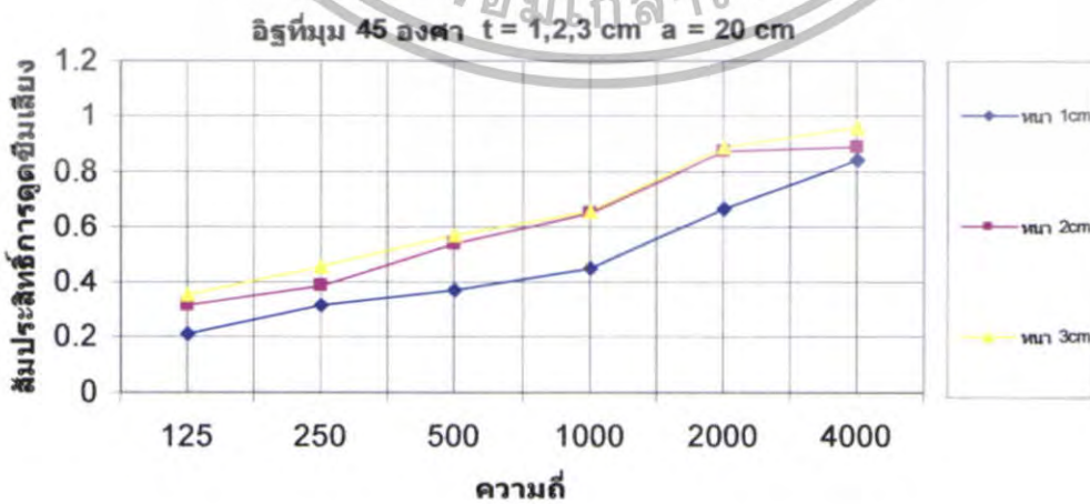
รูปที่ 5.20 สัมประสิทธิ์การดูดซึมเสื่อมของอิฐที่ \theta = 45^\circ t = 1,2,3 \text{ cm} a = 20 \text{ cm}
