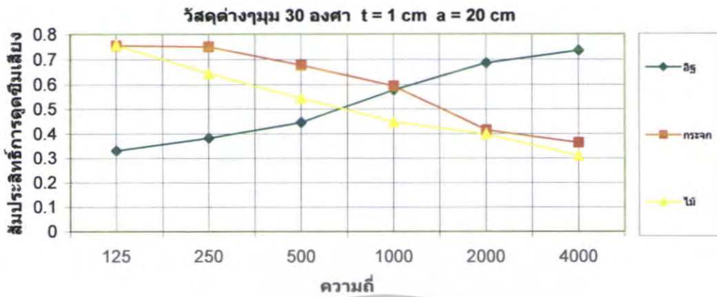
รูปที่ 5.200 สัมประสิทธิ์การดูดซึมเสียงของวัสดุต่างๆ \theta = 30^\circ ที่ t = 1 \text{ cm} a = 20 \text{ cm}
