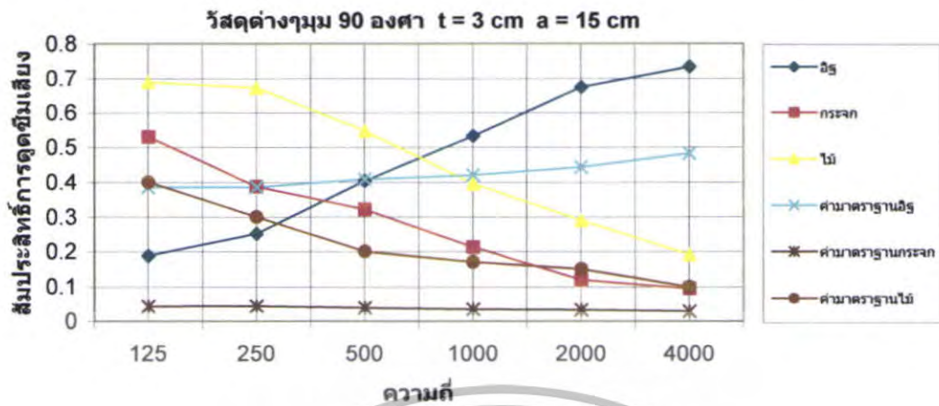
รูปที่ 5.181 สัมประสิทธิ์การดูดซับเสียงของวัสดุต่างๆ \theta = 90^\circ ที่ t = 3 \text{ cm} a = 15 \text{ cm}
