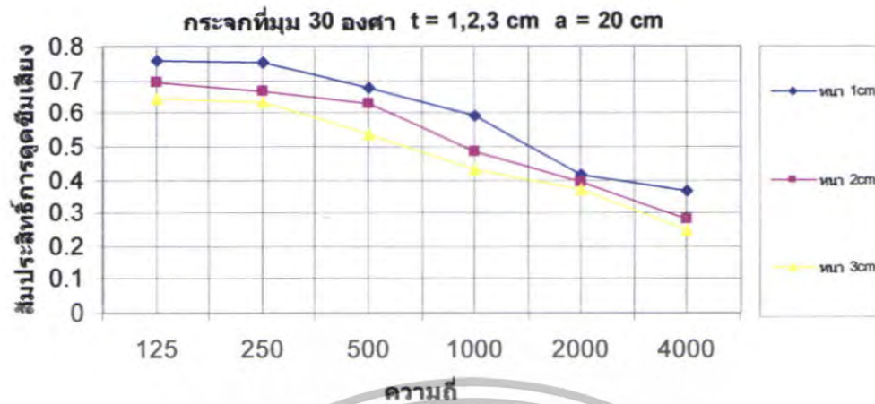
รูปที่ 5.68 สัมประสิทธิ์การดูดซับเสียงของกระจกที่ \theta = 30^\circ t = 1,2,3 \text{ cm} a = 20 \text{ cm}
