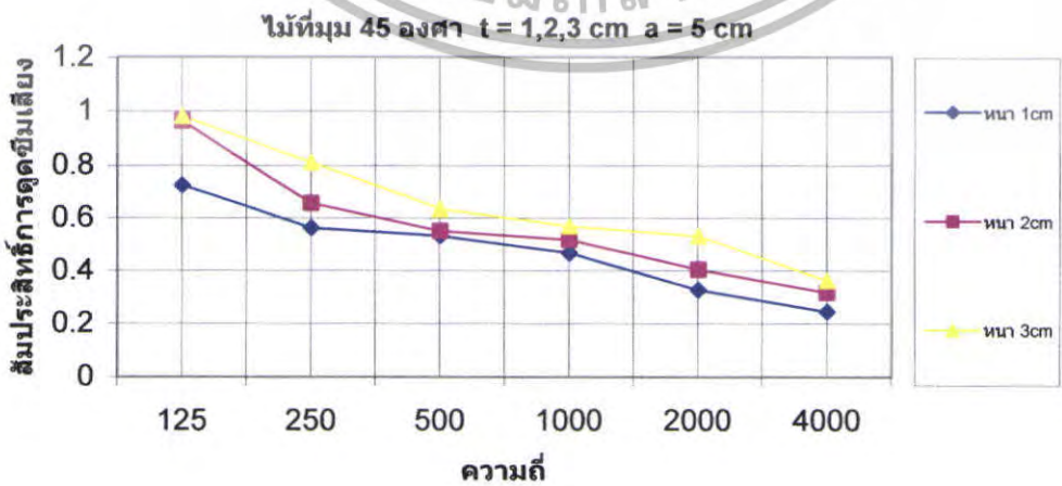
รูปที่ 5.102 สัมประสิทธิ์การดูดซับเชิงเสถียรของไม้ที่ \theta = 45^\circ t = 1,2,3 \text{ cm} a = 5 \text{ cm}
