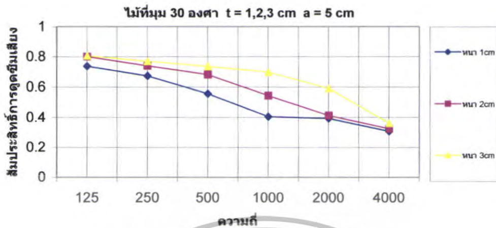
รูปที่ 5.103 สัมประสิทธิ์การดูดซับเสียงของไม้ที่ \theta = 30^\circ t = 1, 2, 3 cm a = 5 cm
