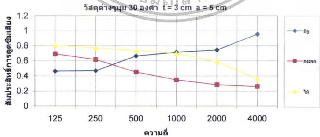
รูปที่ 5.166 สัมประสิทธิ์การดูดซับเสียงของวัสดุต่างๆ \theta = 30^\circ ที่ t = 3 \text{ cm} a = 5 \text{ cm}
