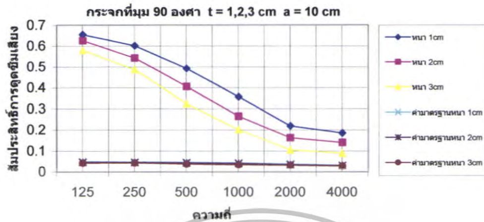
รูปที่ 5.57 สัมประสิทธิ์การดูดซับเสียงของกระเจกที่ \theta = 90^\circ t = 1,2,3 \text{ cm} a = 10 \text{ cm}
