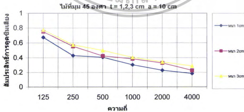
รูปที่ 5.106 สัมประสิทธิ์การดัดขี้นเสียงของไม้ที่ \theta = 45^\circ t = 1,2,3 \text{ cm} a = 10 \text{ cm}
