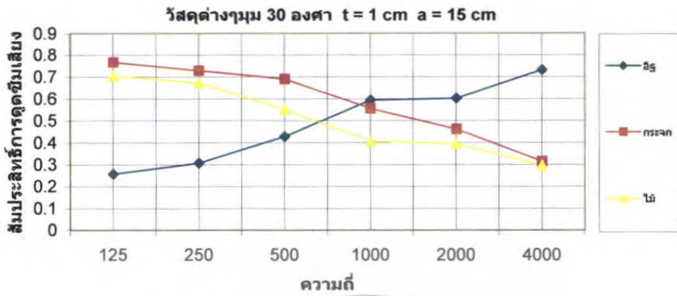
รูปที่ 5.188 สัมประสิทธิ์การดูดซับเชิงเสถียรของวัสดุต่างๆ \theta = 30^\circ ที่ t = 1 \text{ cm} a = 15 \text{ cm}
