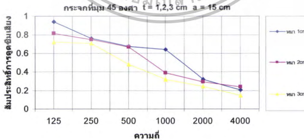
รูปที่ 5.63 สัมประสิทธิ์การดูดซับเสียงของกระบอกที่ \theta = 45^\circ t = 1,2,3 \text{ cm} a = 15 \text{ cm}
