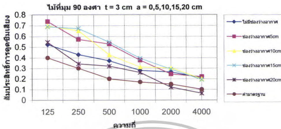
รูปที่ 5.118 สัมประสิทธิ์การดูดซับเสียงของไม้ที่ \theta = 90^\circ t = 3 \text{ cm} a = 5, 10, 15, 20 \text{ cm}
