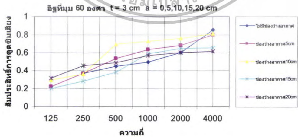
รูปที่ 5.27 สัมประสิทธิ์การดูดซับเสียงของฉลุที่ \theta = 60^\circ t = 3\text{ cm} a = 5,10,15,20\text{ cm}
