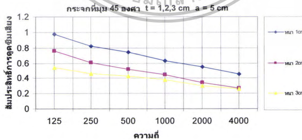
รูปที่ 5.55 สัมประสิทธิ์การดุดซึ่มเสียงของกระฉากที่ \theta = 45^\circ t = 1,2,3 \text{ cm} a = 5 \text{ cm}
