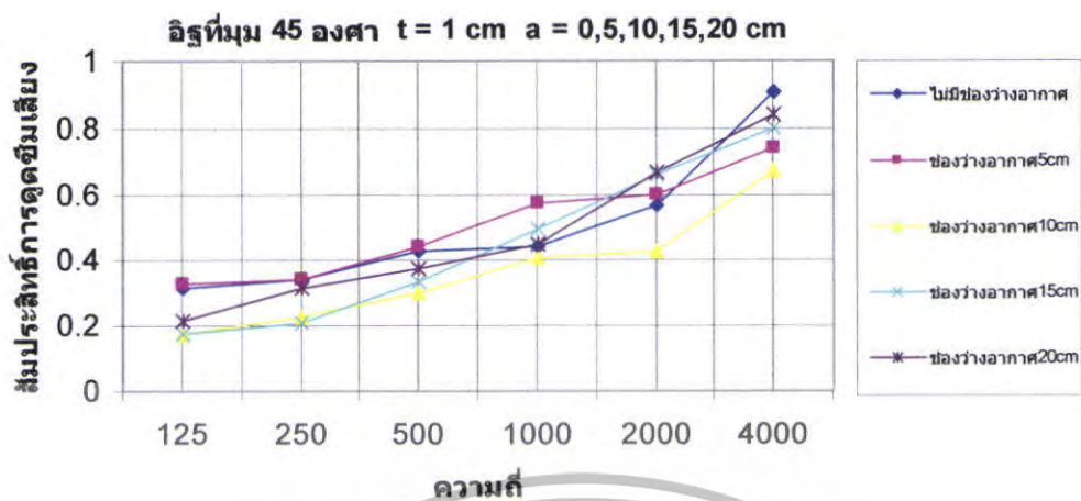
รูปที่ 5.28 สัมประสิทธิ์การดูดซึมเสียงของฉลุที่ \theta = 45^\circ t = 1 \text{ cm} a = 5,10,15,20 \text{ cm}
