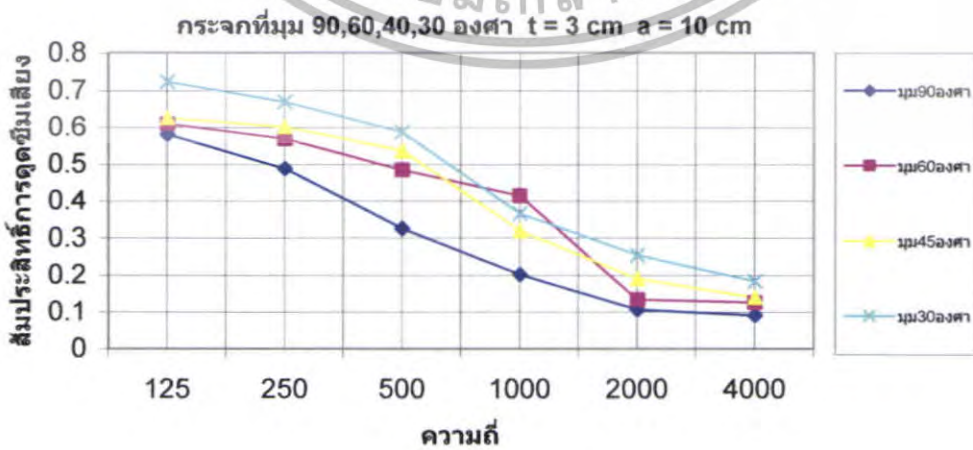
รูปที่ 5.89 สัมประสิทธิ์การดูดซึ่มเสียงของกระจก \theta = 90^\circ, 60^\circ, 45^\circ, 30^\circ ที่ t = 3 cm a = 10 cm เอกสารนี้เป็นเอกสารที่สงวนลิขสิทธิ์สำหรับการใช้งานเพื่อการศึกษาเท่านั้น เมื่อนุญาตเห็นาไปใช้ประโยชน์ด้านการค้า ไม่ว่าจะกรณีใดๆทั้งสิ้น อีกทั้งห้ามมิให้ตัดแปลงเนื้อหา และต้องอ้างอิงถึงเจ้าของเอกสารทุกครั้งที่มีการนำไปใช้
