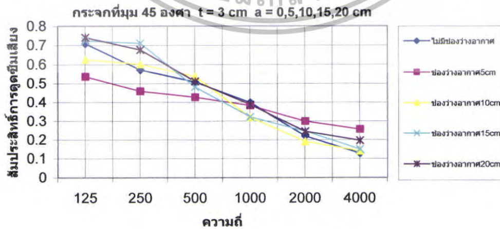
รูปที่ 5.77 สัมประสิทธิ์การดูดซึมเสียงของกระเจกที่ \theta = 45^\circ t = 3 cm a = 5,10,15,20 cm
