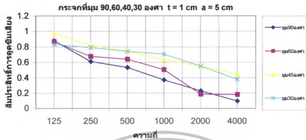
รูปที่ 5.84 สัมประสิทธิ์การดูดซับเสียงของกระบอก \theta = 90^{\circ}, 60^{\circ}, 45^{\circ}, 30^{\circ} ที่ t = 1 cm a = 5 cm
