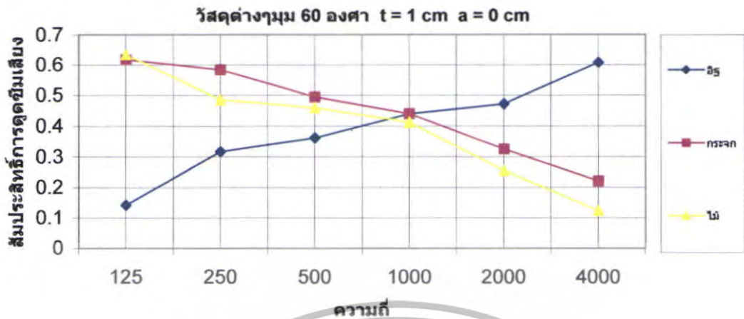
รูปที่ 5.146 สัมประสิทธิ์การดูดซับเสียงของวัสดุต่างๆ \theta = 60^\circ ที่ t = 1 cm a = 0 cm
