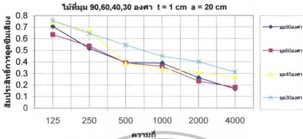
รูปที่ 5.140 สัมประสิทธิ์การดูดซับเสียงของไม้ \theta = 90^\circ, 60^\circ, 45^\circ, 30^\circ ที่ t = 1 \text{ cm} a = 20 \text{ cm}
