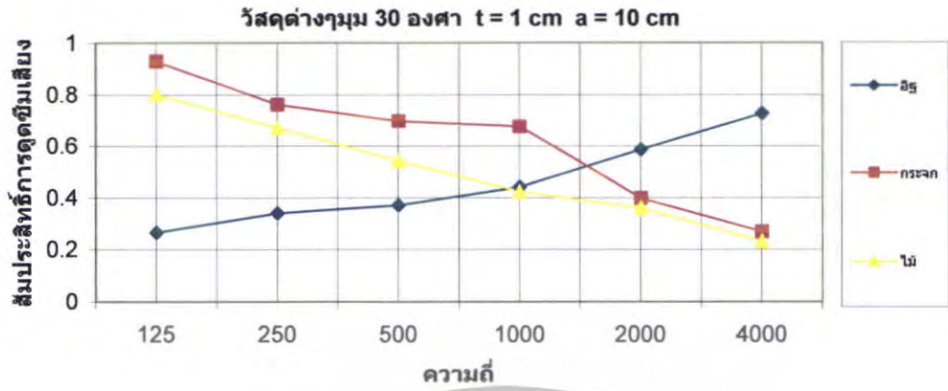
รูปที่ 5.176 สัมประสิทธิ์การดูดซึมเสียงของวัสดุต่างๆ \theta = 30^\circ ที่ t = 1 \text{ cm} a = 10 \text{ cm}
