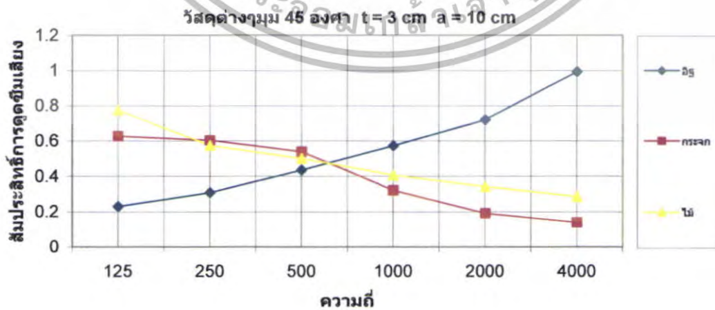
รูปที่ 5.175 สัมประสิทธิ์การดัดขีมิเปลี่ยนของวัสดุต่างๆ \theta = 45^\circ ที่ t = 3 \text{ cm} a = 10 \text{ cm}
