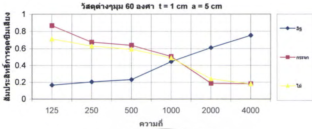
รูปที่ 5.158 สัมประสิทธิ์การดูดซับเสียงของวัสดุต่างๆ \theta = 60^\circ ที่ t = 1 cm a = 5 cm
