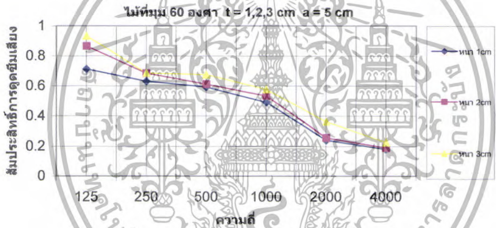
รูปที่ 5.101 สัมประสิทธิ์การดูดซับเชิงเสถียรของไม้ที่ \theta = 60^\circ t = 1,2,3 \text{ cm} a = 5 \text{ cm}
