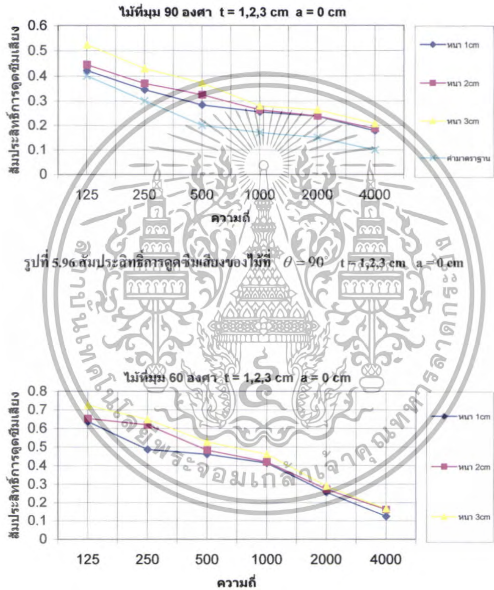
รูปที่ 5.97 สัมประสิทธิ์การดูดซึมเสียงของไม้ที่ \theta = 60^\circ t = 1,2,3 cm a = 0 cm
