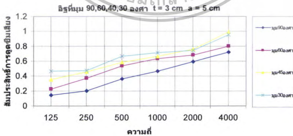
รูปที่ 5.39 สัมประสิทธิ์การดัดขี้นเสียงของอิฐ \theta = 90^\circ, 60^\circ, 45^\circ, 30^\circ ที่ t = 3 \text{ cm} a = 5 \text{ cm}
