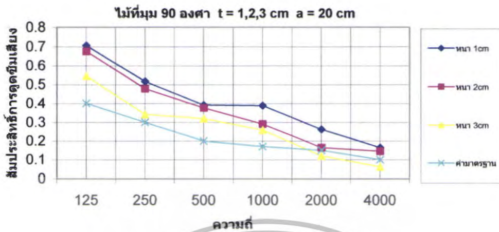
รูปที่ 5.112 สัมประสิทธิ์การดัดขี้นเคียงของไม้ที่ \theta = 90^\circ t = 1,2,3 \text{ cm} a = 20 \text{ cm}
