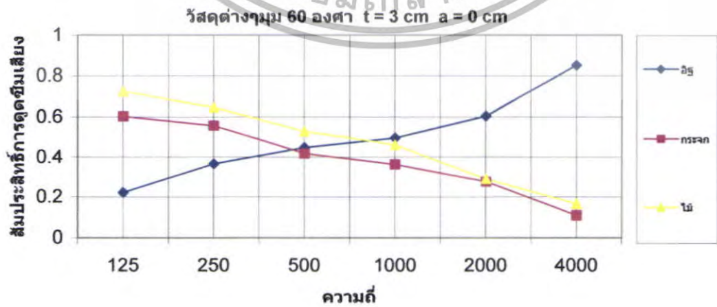
รูปที่ 5.148 สัมประสิทธิ์การดูดซับเสียงของวัสดุต่างๆ \theta = 60^\circ ที่ t = 3 cm a = 0 cm
