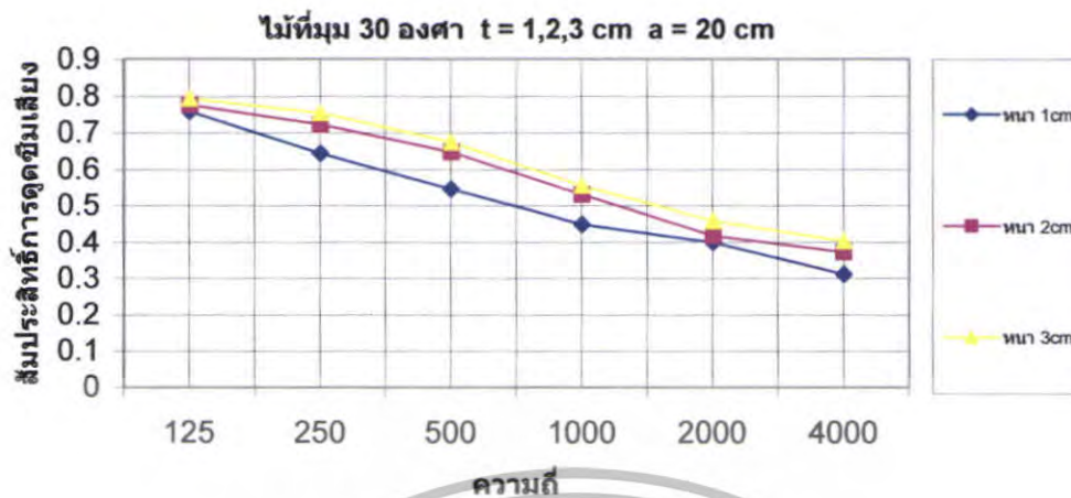
รูปที่ 5.115 สัมประสิทธิ์การดุดับเชิงมุมของไม้ที่ \theta = 30^\circ t = 1,2,3 \text{ cm} a = 20 \text{ cm}
