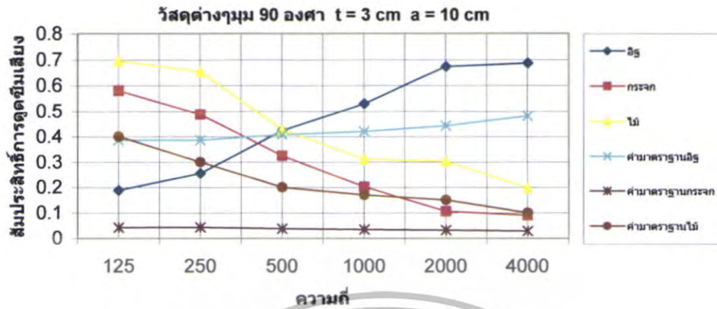
รูปที่ 5.169 สัมประสิทธิ์การดูดซับเสียงของวัสดุต่างๆ \theta = 90^\circ ที่ t = 3 \text{ cm} a = 10 \text{ cm}
