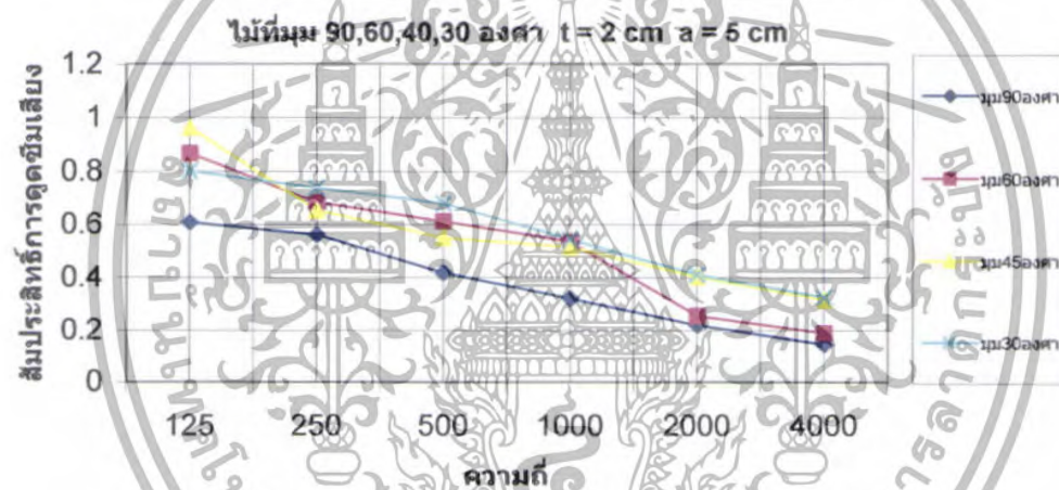
รูปที่ 5.132 สัมประสิทธิ์การดูดซึมเสียงของไม้ \theta = 90^\circ, 60^\circ, 45^\circ, 30^\circ ที่ t = 2 \text{ cm} a = 5 \text{ cm}
