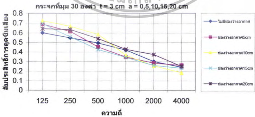
รูปที่ 5.80 สัมประสิทธิ์การดูดซับเสียงของกระจกที่ \theta = 30^\circ t = 3 \text{ cm} a = 5,10,15,20 \text{ cm}
