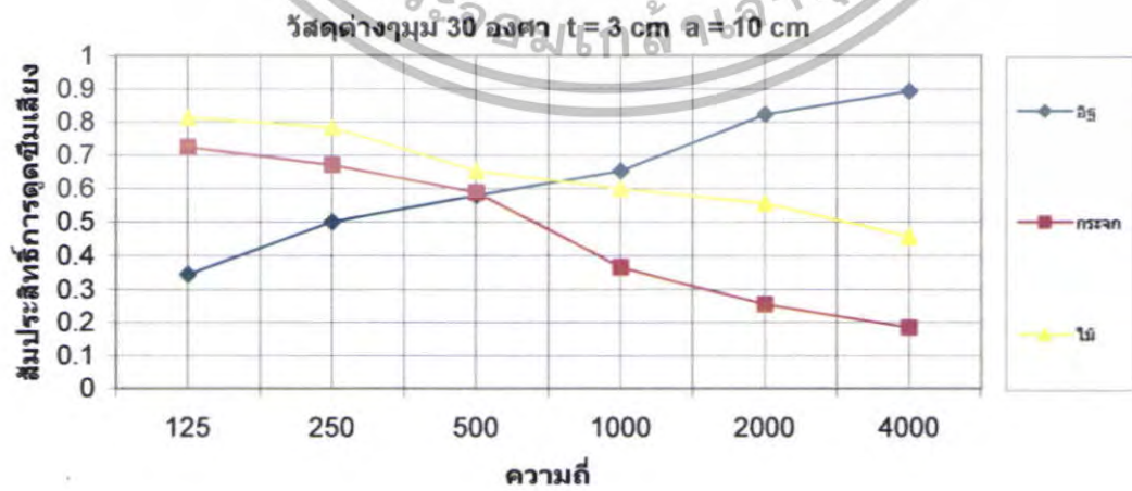
รูปที่ 5.178 สัมประสิทธิ์การดูดซึมเสียงของวัสดุต่างๆ \theta = 30^\circ ที่ t = 3 \text{ cm} a = 10 \text{ cm}
