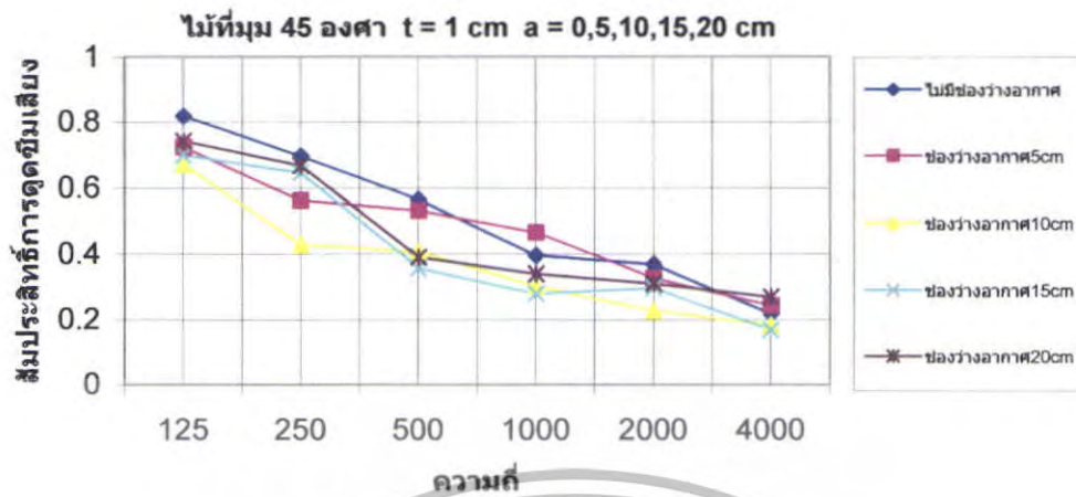
รูปที่ 5.122 สัมประสิทธิ์การดัดขี้นเสียงของไม้ที่ \theta = 45^\circ t = 1 cm a = 5,10,15,20 cm
