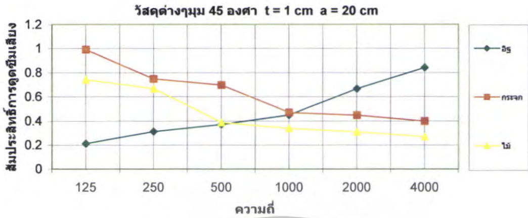
รูปที่ 5.197 สัมประสิทธิ์การดัดขี้นเสียงของวัสดุต่างๆ \theta = 45^\circ ที่ t = 1 \text{ cm} a = 20 \text{ cm}
