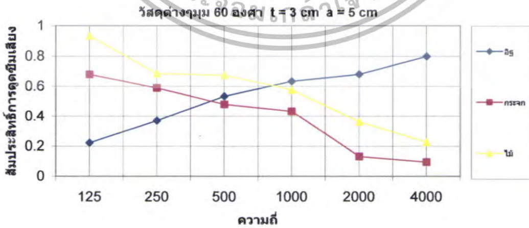
รูปที่ 5.160 สัมประสิทธิ์การดูดซับเสียงของวัสดุต่างๆ \theta = 60^\circ ที่ t = 3 cm a = 5 cm
