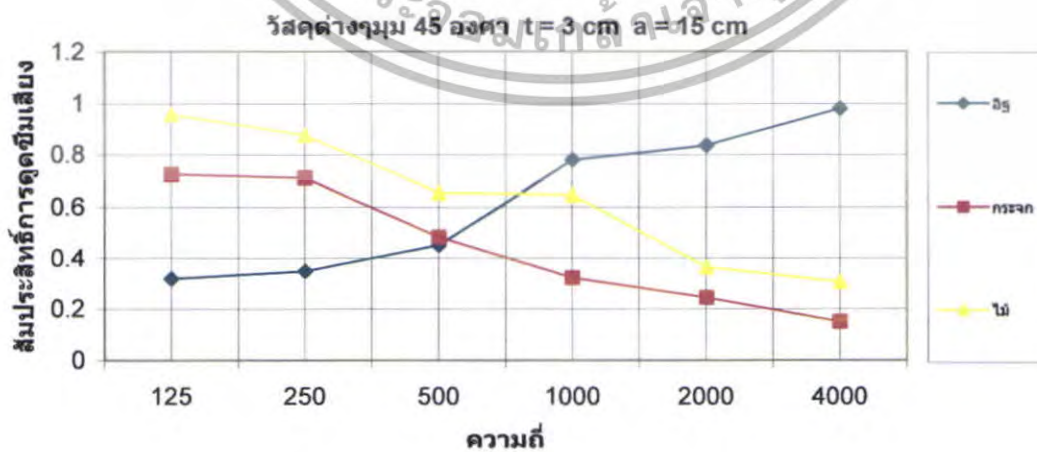
รูปที่ 5.187 สัมประสิทธิ์การดัดขี้นเฉียงของวัสดุต่างๆ \theta = 45^\circ ที่ t = 3 \text{ cm} a = 15 \text{ cm}
