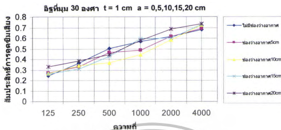
รูปที่ 5.31 สัมประสิทธิ์การดูดซับเสียงของอิฐที่ \theta = 30^\circ t = 1 \text{ cm} a = 5,10,15,20 \text{ cm}
