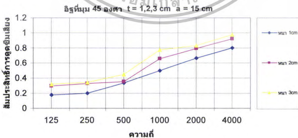
รูปที่ 5.16 สัมประสิทธิ์การดูดซึมน้ำของอิฐที่ \theta = 45^\circ t = 1,2,3 \text{ cm} a = 15 \text{ cm}
