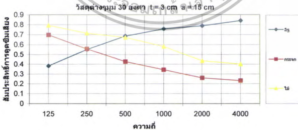
รูปที่ 5.190 สัมประสิทธิ์การดูดซับเชิงเสถียรของวัสดุต่างๆ \theta = 30^\circ ที่ t = 3 \text{ cm} a = 15 \text{ cm}
