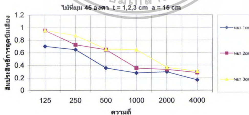
รูปที่ 5.110 สัมประสิทธิ์การดูดซับเสียงของไม้ที่ \theta = 45^\circ t = 1,2,3 \text{ cm} a = 15 \text{ cm}
