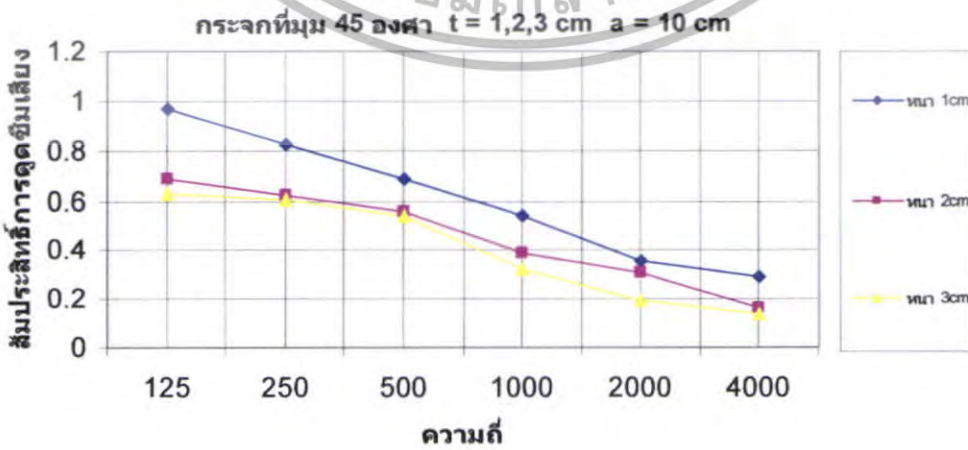
รูปที่ 5.59 สัมประสิทธิ์การดูดซับเสียงของกระเจกที่ \theta = 45^\circ t = 1,2,3 \text{ cm} a = 10 \text{ cm}
