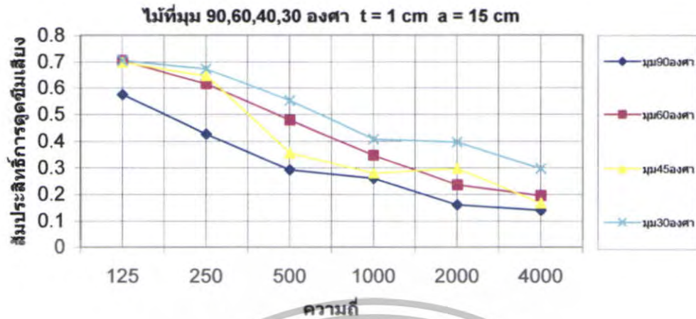
รูปที่ 5.137 สัมประสิทธิ์การหดขีมีเปลี่ยนแปลงของไม้ \theta = 90^{\circ}, 60^{\circ}, 45^{\circ}, 30^{\circ} ที่ t = 1 cm a = 15 cm
