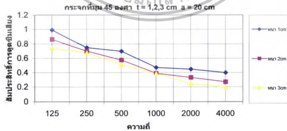
รูปที่ 5.67 สัมประสิทธิ์การดูดซับเสียงของกระจกที่ \theta = 45^\circ t = 1,2,3 \text{ cm} a = 20 \text{ cm}
