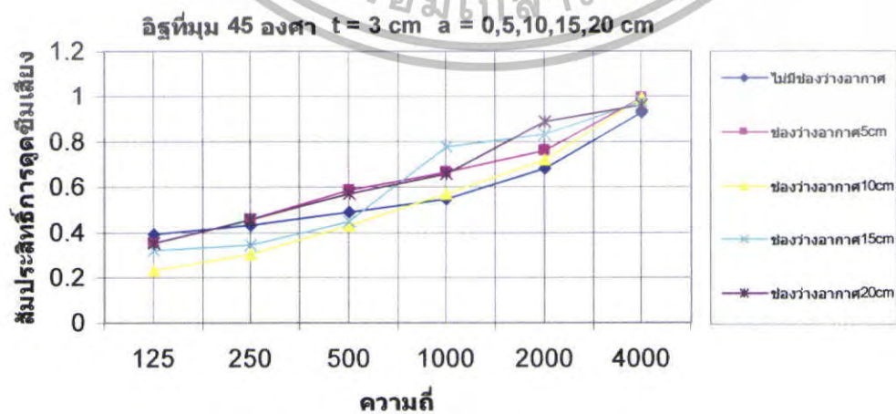
รูปที่ 5.30 สัมประสิทธิ์การดูดซึมเสียงของฉลุที่ \theta = 45^\circ t = 3 \text{ cm} a = 5,10,15,20 \text{ cm}
