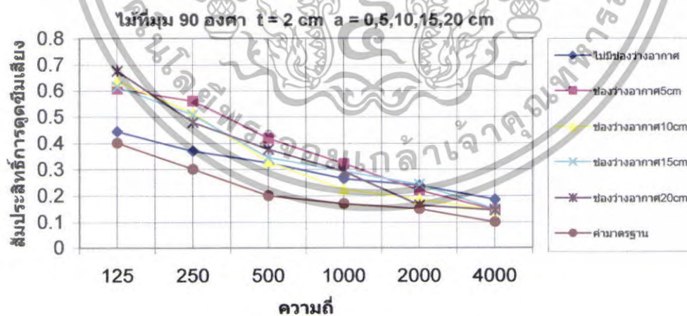
รูปที่ 5.117 สัมประสิทธิ์การดูดซึมเสียงของไม้ที่ \theta = 90^\circ t = 2 cm a = 5,10,15,20 cm
