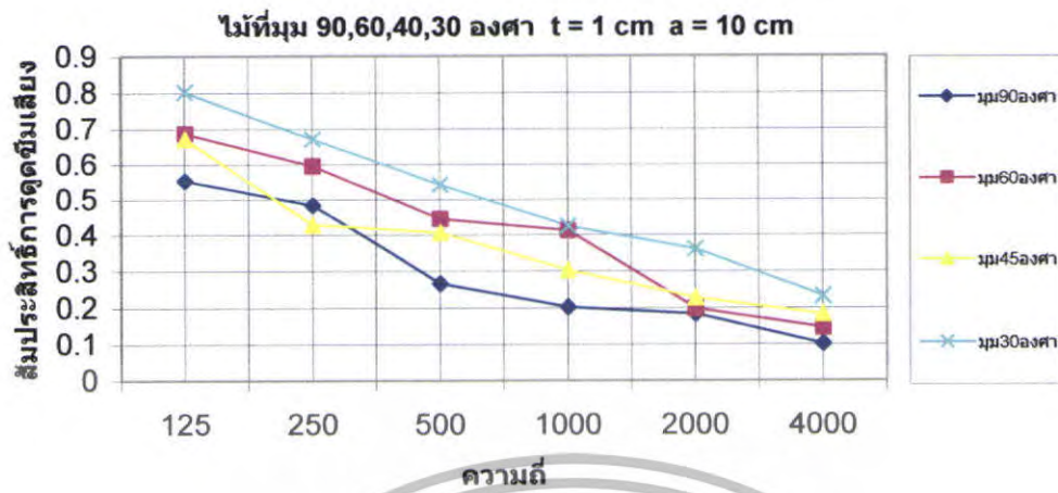
รูปที่ 5.134 สัมประสิทธิ์การหดขี้นเสียงของไม้ \theta = 90^\circ, 60^\circ, 45^\circ, 30^\circ ที่ t = 1 cm a = 10 cm
