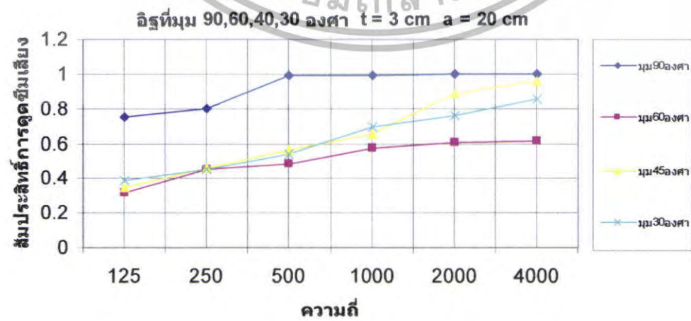
รูปที่ 5.48 สัมประสิทธิ์การดัดขีมิเสียงของอิฐ \theta = 90^{\circ}, 60^{\circ}, 45^{\circ}, 30^{\circ} ที่ t = 3 \text{ cm} a = 20 \text{ cm}
