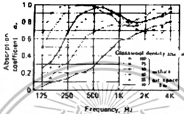
รูปที่ 3.14 สัมประสิทธิ์การดูดซับเสียงของใยแก้ว ที่ความหนาต่าง ๆ
