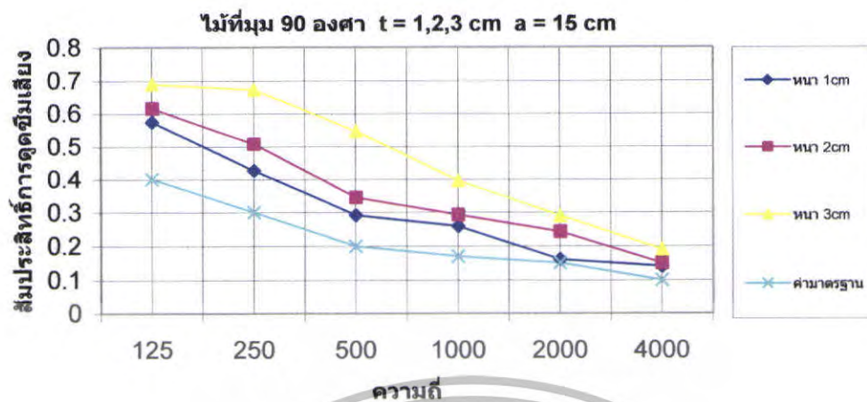
รูปที่ 5.108 สัมประสิทธิ์การดูดซับเสียงของไม้ที่ \theta = 90^\circ t = 1,2,3 \text{ cm} a = 15 \text{ cm}
