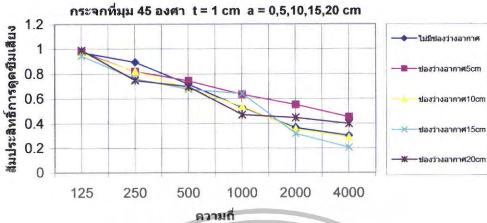
รูปที่ 5.75 สัมประสิทธิ์การดูดซึมเสียงของกระเจกที่ \theta = 45^\circ t = 1 cm a = 5,10,15,20 cm
