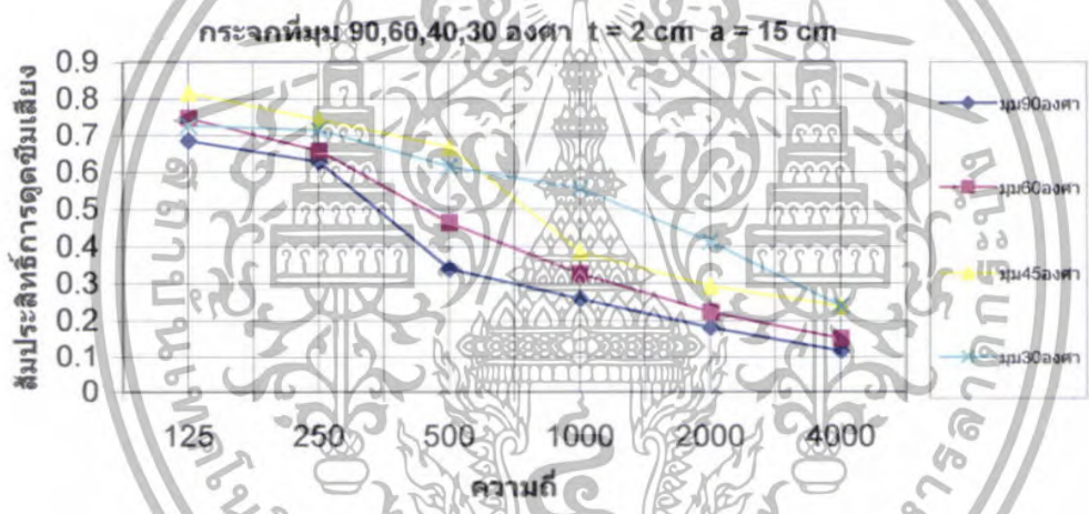
รูปที่ 5.91 สัมประสิทธิ์การดูดซึมเสียงของกระบอก \theta = 90^\circ, 60^\circ, 45^\circ, 30^\circ ที่ t = 2 \text{ cm} a = 15 \text{ cm}
