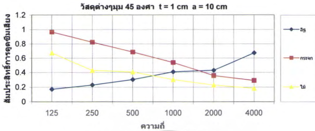
รูปที่ 5.173 สัมประสิทธิ์การดัดขีมิเปลี่ยนของวัสดุต่างๆ \theta = 45^\circ ที่ t = 1 \text{ cm} a = 10 \text{ cm}
