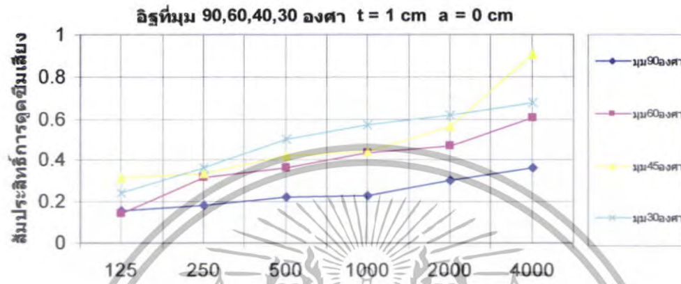
รูปที่ 5.34 สัมประสิทธิ์การดูดซึมเสียงของอิฐ \theta = 90^\circ, 60^\circ, 45^\circ, 30^\circ ที่ t = 1 \text{ cm} a = 0 \text{ cm}
