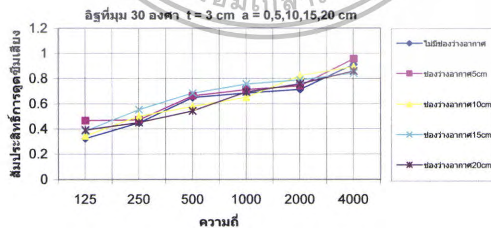
รูปที่ 5.33 สัมประสิทธิ์การดูดซับเสียงของอิฐที่ \theta = 30^\circ t = 3 \text{ cm} a = 5,10,15,20 \text{ cm}
