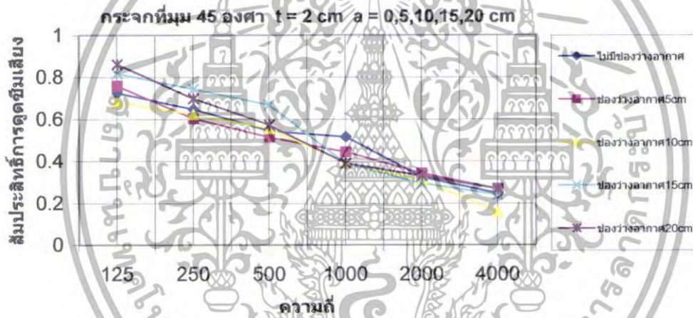
รูปที่ 5.76 สัมประสิทธิ์การดูดซึมเสียงของกระเจกที่ \theta = 45^\circ t = 2 cm a = 5,10,15,20 cm
