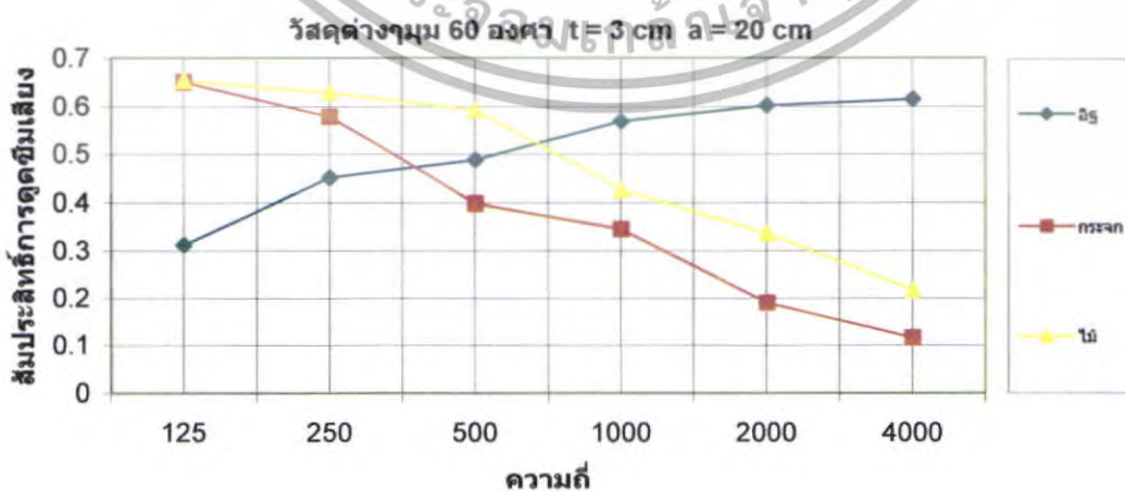
รูปที่ 5.196 สัมประสิทธิ์การดูดซับเสียงของวัสดุต่างๆ \theta = 60^\circ ที่ t = 3 \text{ cm} a = 20 \text{ cm}
