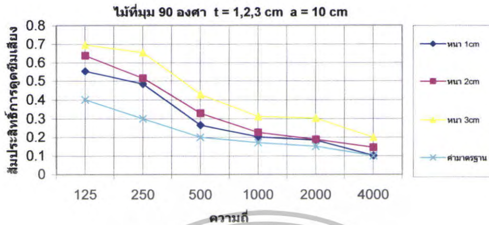
รูปที่ 5.104 สัมประสิทธิ์การดัดขี้นเสียงของไม้ที่ \theta = 90^\circ t = 1,2,3 \text{ cm} a = 10 \text{ cm}
