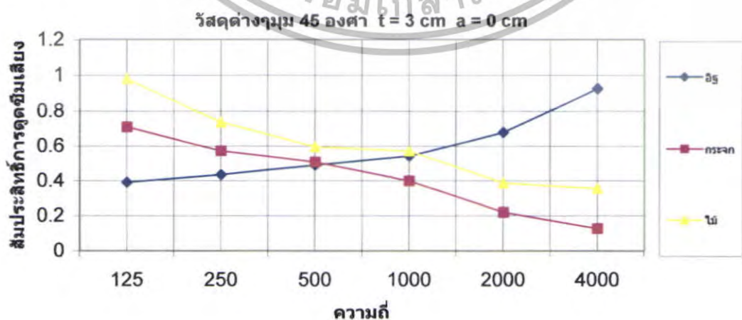
รูปที่ 5.151 สัมประสิทธิ์การดูดซึมเสียงของวัสดุต่างๆ \theta = 45^\circ ที่ t = 3 \text{ cm} a = 0 \text{ cm}
