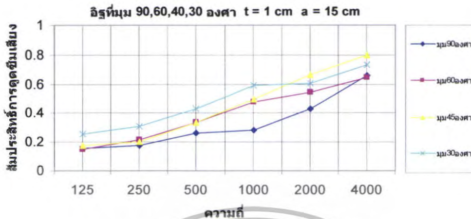
รูปที่ 5.43 สัมประสิทธิ์การดัดขี้นเสียงของอิฐ \theta = 90^\circ, 60^\circ, 45^\circ, 30^\circ ที่ t = 1 \text{ cm} a = 15 \text{ cm}
