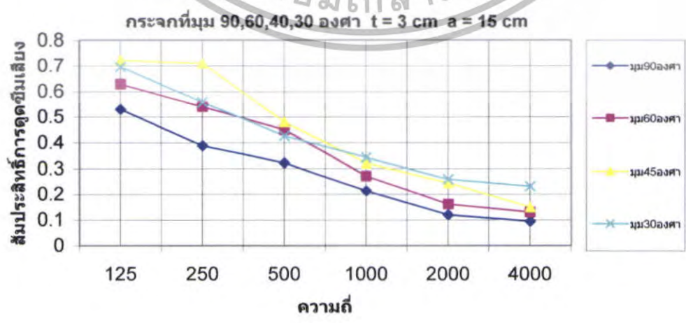
รูปที่ 5.92 สัมประสิทธิ์การดูดซึมเสียงของกระบอก \theta = 90^\circ, 60^\circ, 45^\circ, 30^\circ ที่ t = 3 \text{ cm} a = 15 \text{ cm}
