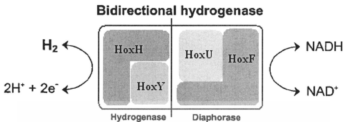
รูปที่ 2.8 แบบจำลองโครงสร้างและการทำงานของเอนไซม์รีเวอร์สซิบิลไฮโดรจีเนส ที่มา : Tamagnini และคณะ (2002)
