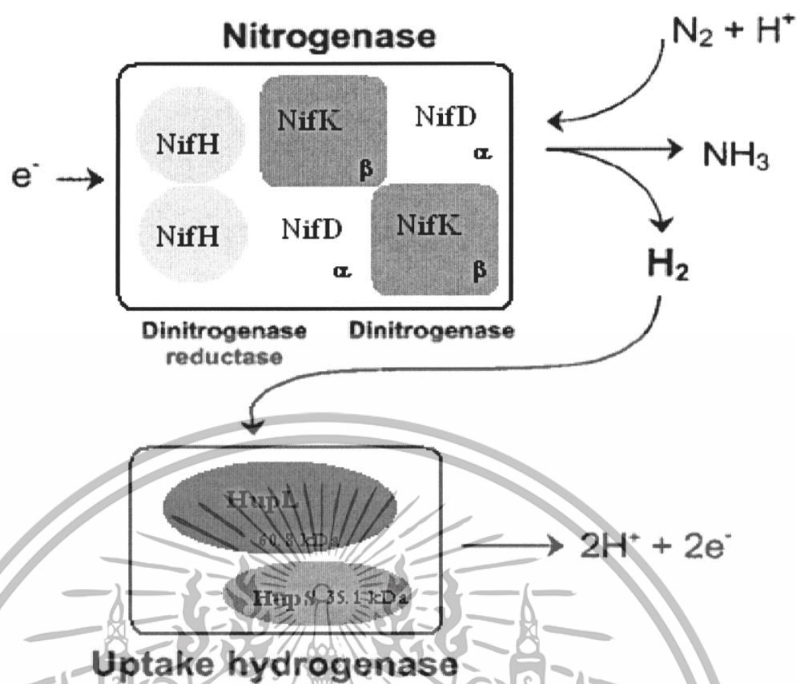
รูปที่ 2.7 แบบจำลองโครงสร้างของอินอ็อปเทคไฮโดรจีเนส
