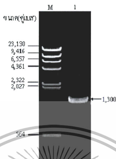
รูปที่ 4.7 ผลึกทัศน์ PCR ของไซยาโนแบคทีเรียรูปร่างกลมที่คัดแยกได้ที่ผ่านการทำให้บริสุทธิ์ด้วยชุดแยกดีเอ็นเอออกจากเจล
