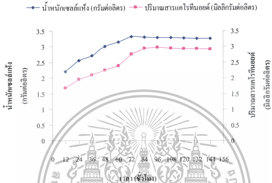
รูปที่ 15 ผลของเวลาที่มีต่อน้ำหนักเซลล์แห้งและปริมาณของสารแคโรทีนอยด์ที่ได้จากเชื้อยีสต์ R. glutinis ในอาหารที่เป็นสารสกัดจากกากส้มปรีดที่สกัดด้วยสารละลายกรด
