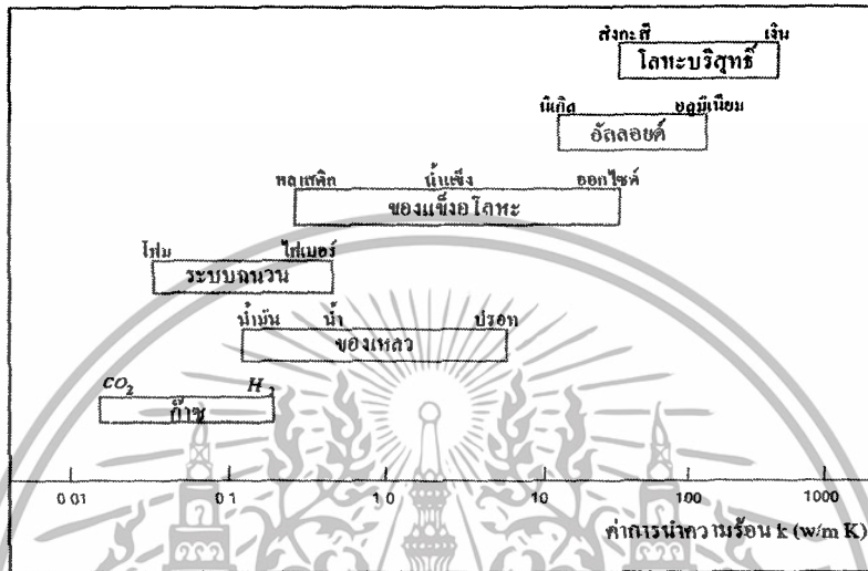
รูปที่ 2.20 ช่วงค่าการนำความร้อนของสารต่างๆ
