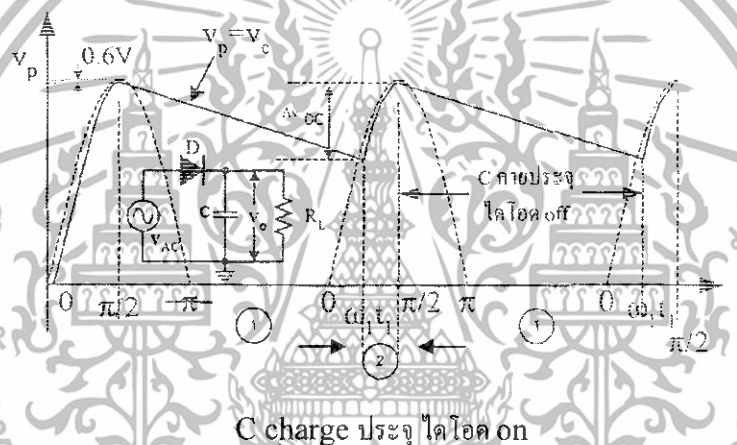
ภาพที่ 2-7 การทำงานของตัวเก็บประจุกรองไฟ ในสถานะที่มีโหลด
