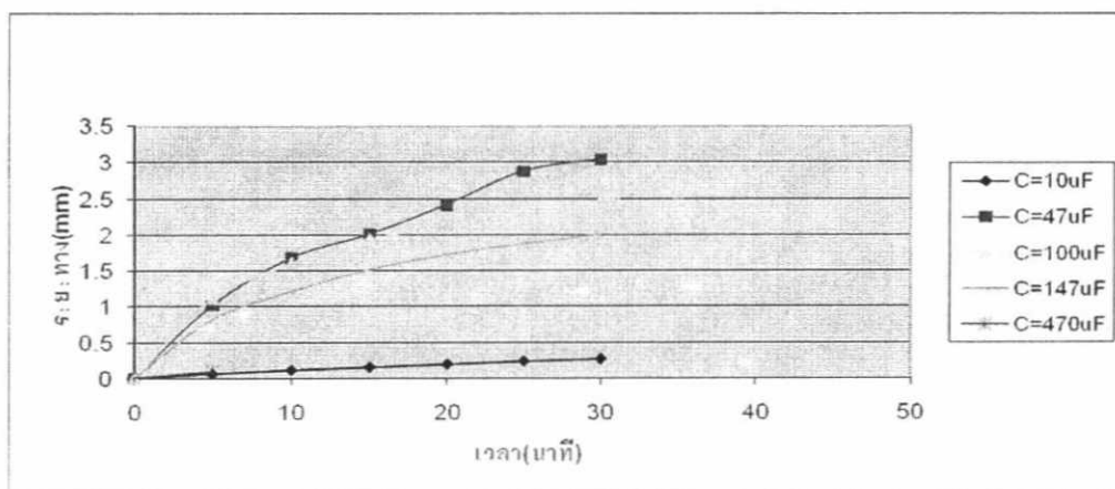
ภาพที่ 4-1 กราฟแสดงความสัมพันธ์ระหว่างระยะทางและเวลา
