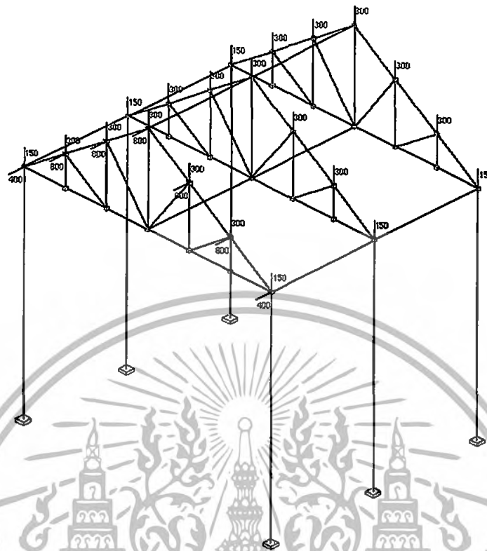
รูปที่ 4.17 โครงสร้าง Truss พร้อมแรงที่กระทำต่อโครงสร้าง
