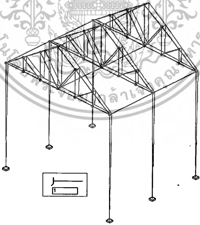
รูปที่ 4.18 การอ่อนแอนในโครงสร้าง Truss เมื่อใช้ Over Scale 1 เท่า
