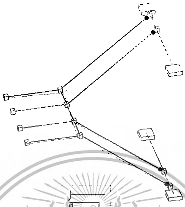
รูปที่ 4.61 การแอนแอนในโครงสร้าง Dog Leg Stair เมื่อใช้ Over Scale 1 เท่า (ภาพสามมิติ) (3)
