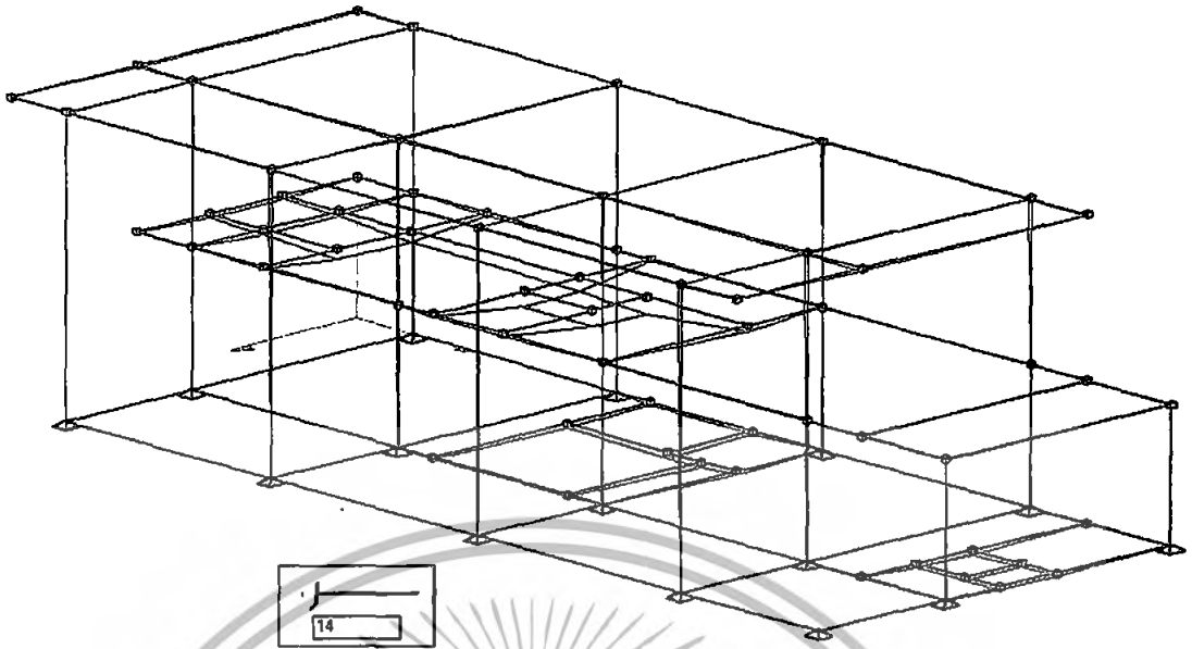
รูปที่ 4.91 การแ่่นแอนในโครงสร้าง บ้านพักอาศัยสองชั้นเมื่อใช้ Over Scale 14 เท่า
