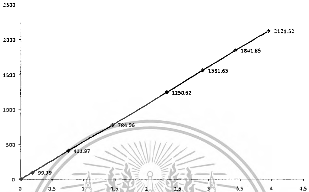
รูปที่ 4.32 Bending Moment Diagram ที่เสาในโครงสร้าง Flat Slab
