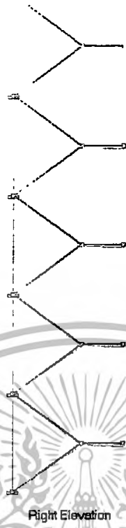
รูปที่ 4.123 การแอนนอบันได Dog Leg ในอาคารพักอาศัยหกชั้นชั้น เมื่อใช้ Over Scale 14 เท่า
