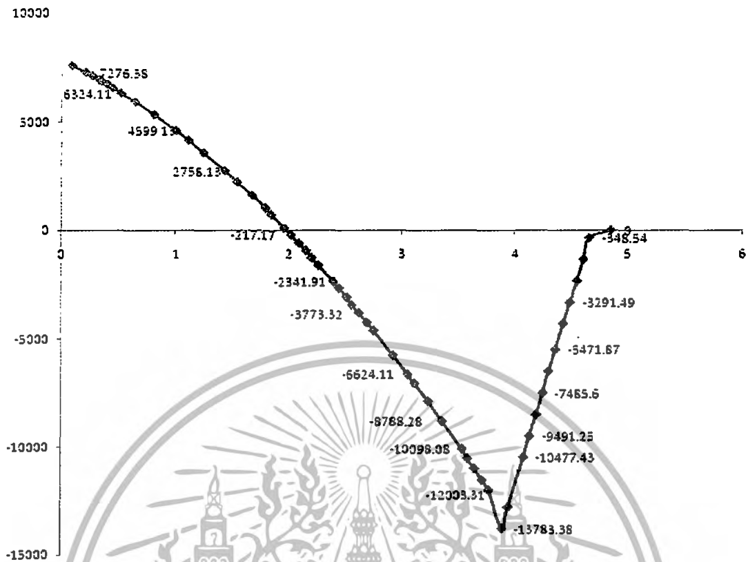
รูปที่ 4.97 Bending Moment Diagram เฉพาะค่าที่ Critical ชั้นสอง (2)
