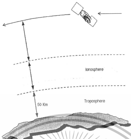
รูปที่ 2.13 แสดงชั้นบรรยากาศโทรโพสเฟียร์
