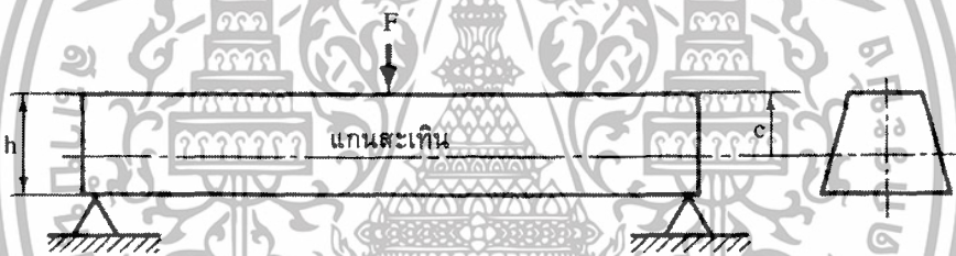
รูปที่ 2.12 คานและแกนสะเทิน
