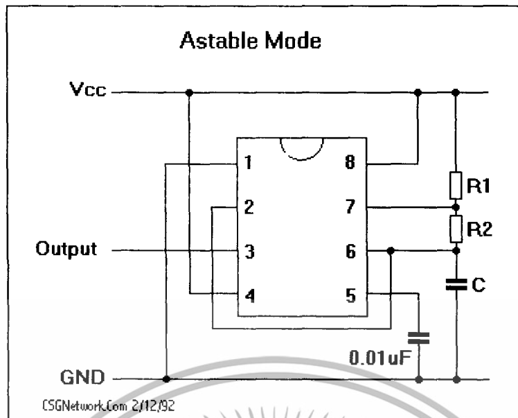
รูปที่ 2.38 แสดงวงจร ออสเตเบิลมีคิตไวยเบรเตอร์ 38 kHz
