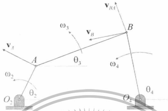
รูปที่ 2.9 การวิเคราะห์ความเร็วโดยวิธีคณิตวิเคราะห์
