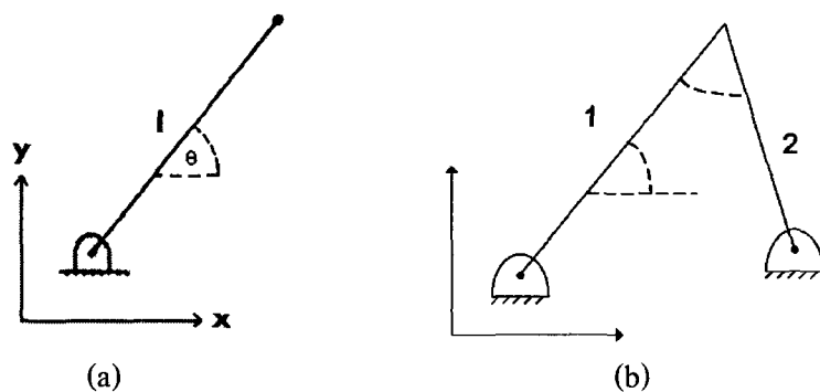
รูปที่ 2.6 ลักษณะการเชื่อมต่อและระดับอิสระในการเคลื่อนที่ของชิ้นต่อโยง
