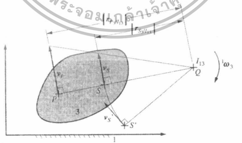
รูปที่ 2.8 การใช้จุดศูนย์กลางชั่วขณะในการวิเคราะห์หาความเร็วของกลไก
