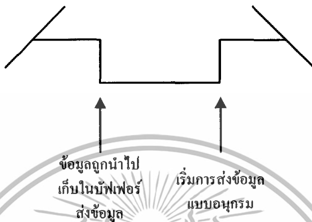
รูปที่ 2.19 สัญญาณค่าได้อินพุทสโตรบ
