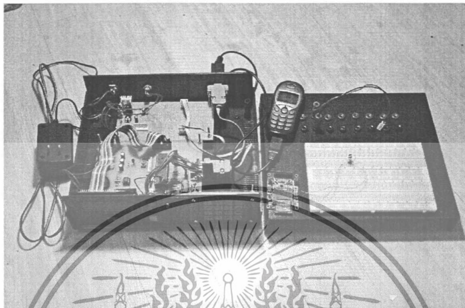
รูปที่ 3.24 โครงสร้างภายในของเครื่องบันทึกข้อมูลและการเตือนแบบ SMS
