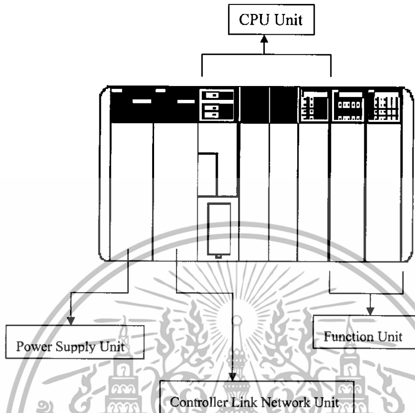
รูปที่ 2.15 ส่วนประกอบของทีแอลซี
