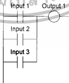
รูปที่ 2.7 ภาษา Ladder Diagram
