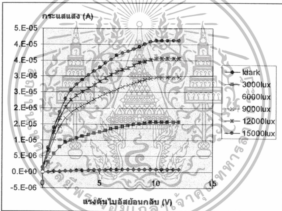
รูปที่ 4.7 ผลของกระแสแสงกับความเข้มแสงค่าต่าง ๆ ของซิลิคอนโฟโอดีไดโอดชนิด PIN แบบแนวตั้งแถวยาว
