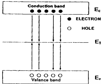
รูปที่ 2.17 กระบวนการรวมตัวใหม่ในสารกึ่งตัวนำแบบโคออร์ดิเนต
