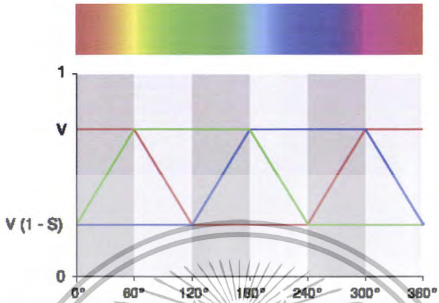
รูปที่ 2.10 กราฟแสดงค่า Hue angle
