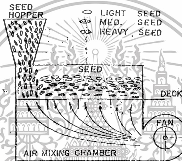
ภาพที่ 2.10 ภาพตัดขวางของเครื่องคัดแยกโดยใช้ลม
